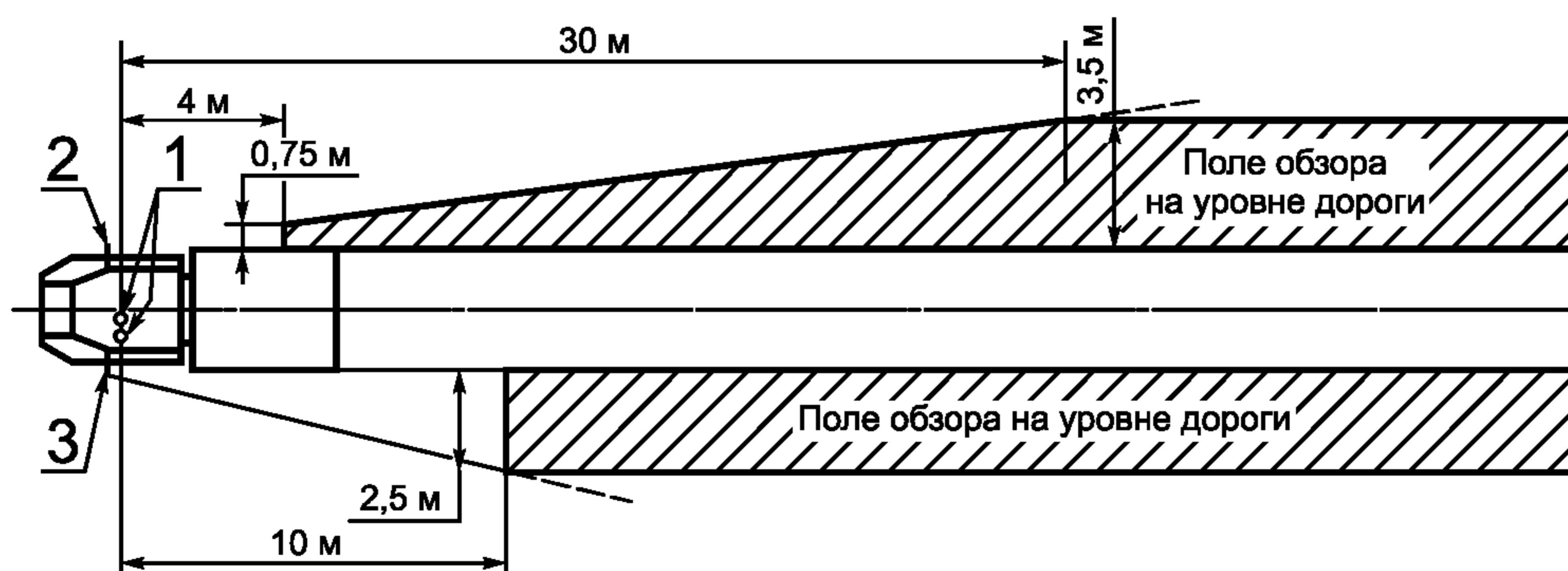
Рисунок 3 — Транспортные средства, помимо предусмотренных на рисунке 4
