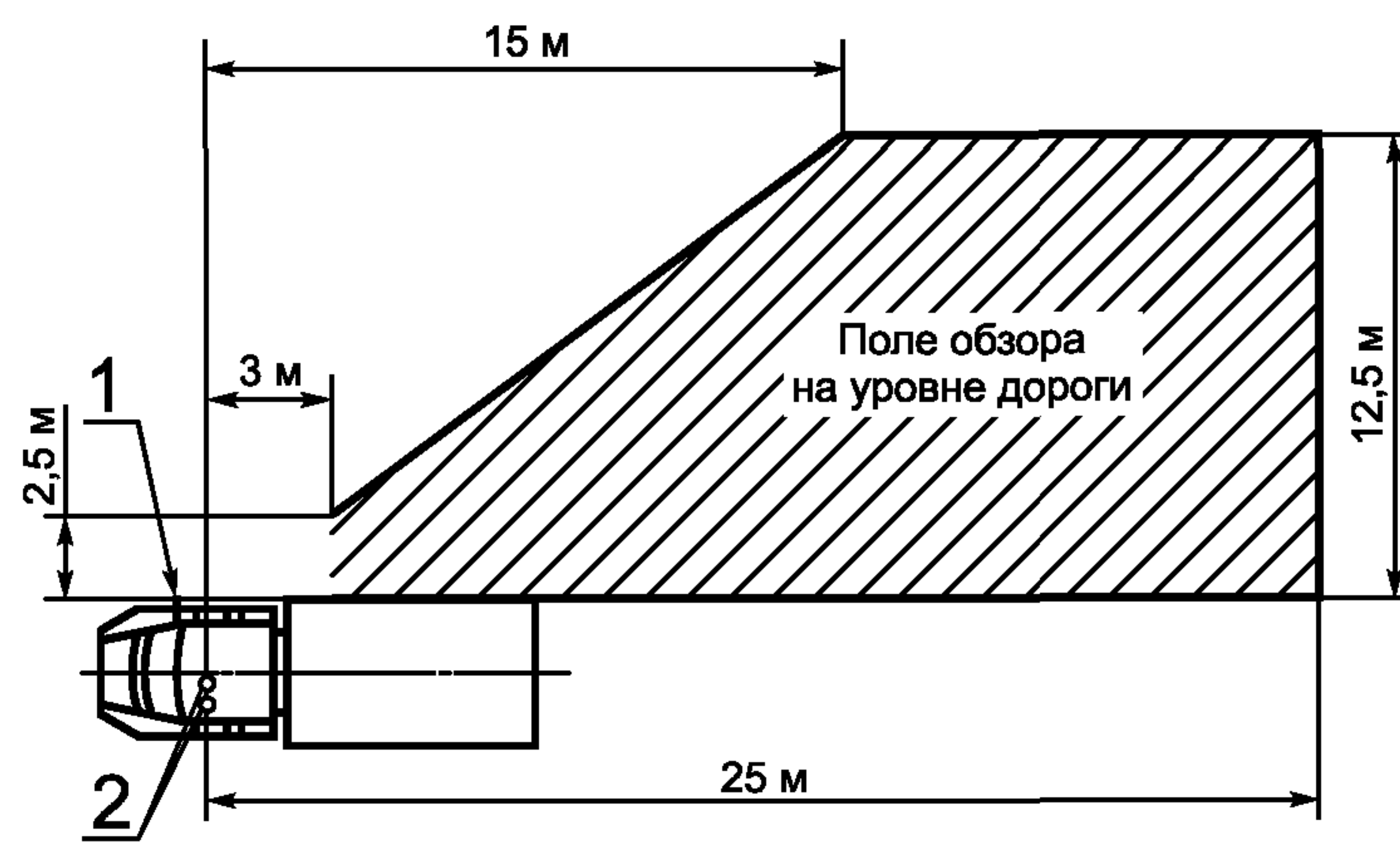
1 — зеркало заднего вида; 2 — окулярные точки водителя
