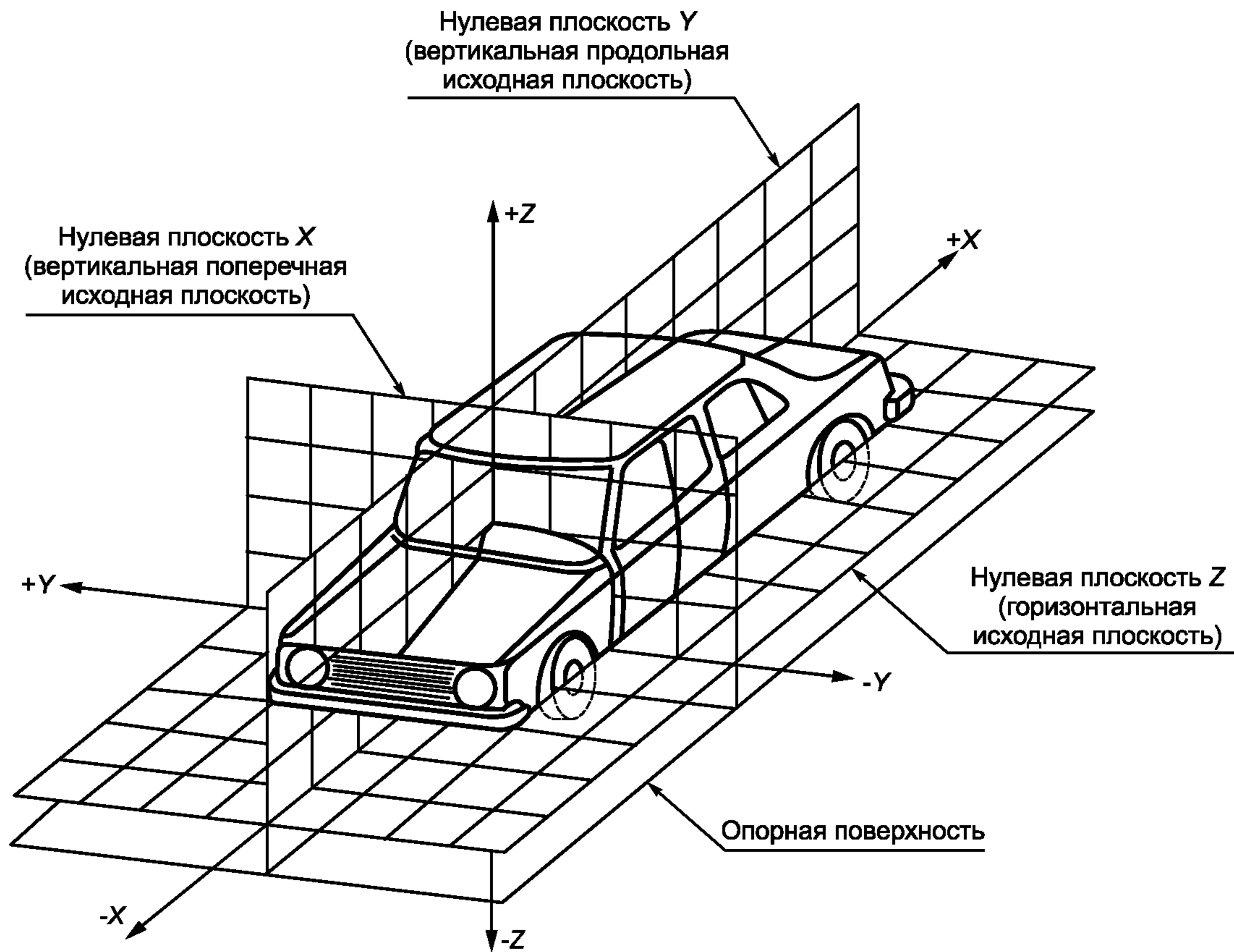
Рисунок — Трехмерная система координат
