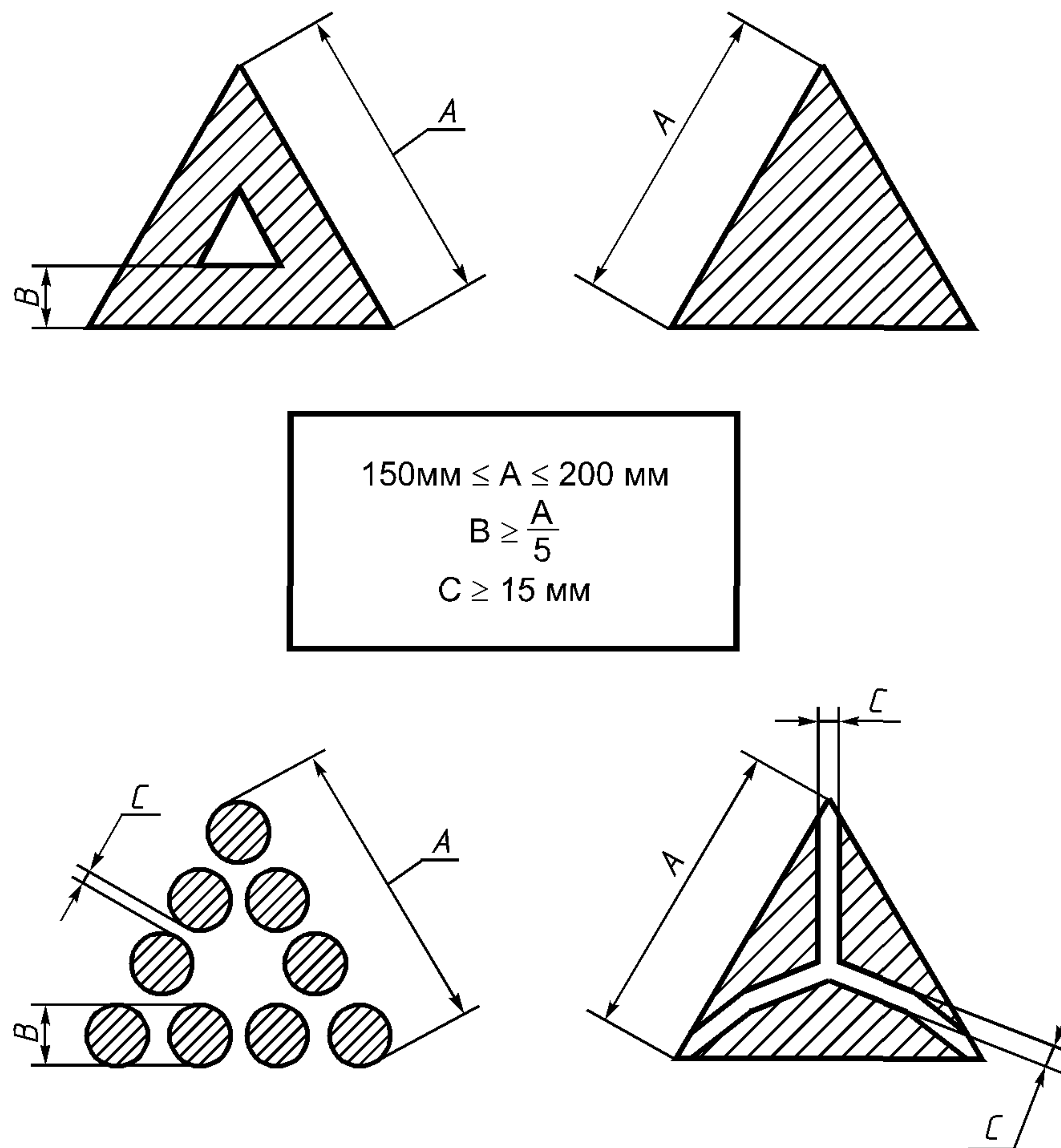
Рисунок 1 — Отражатели света для прицепов класса III A
