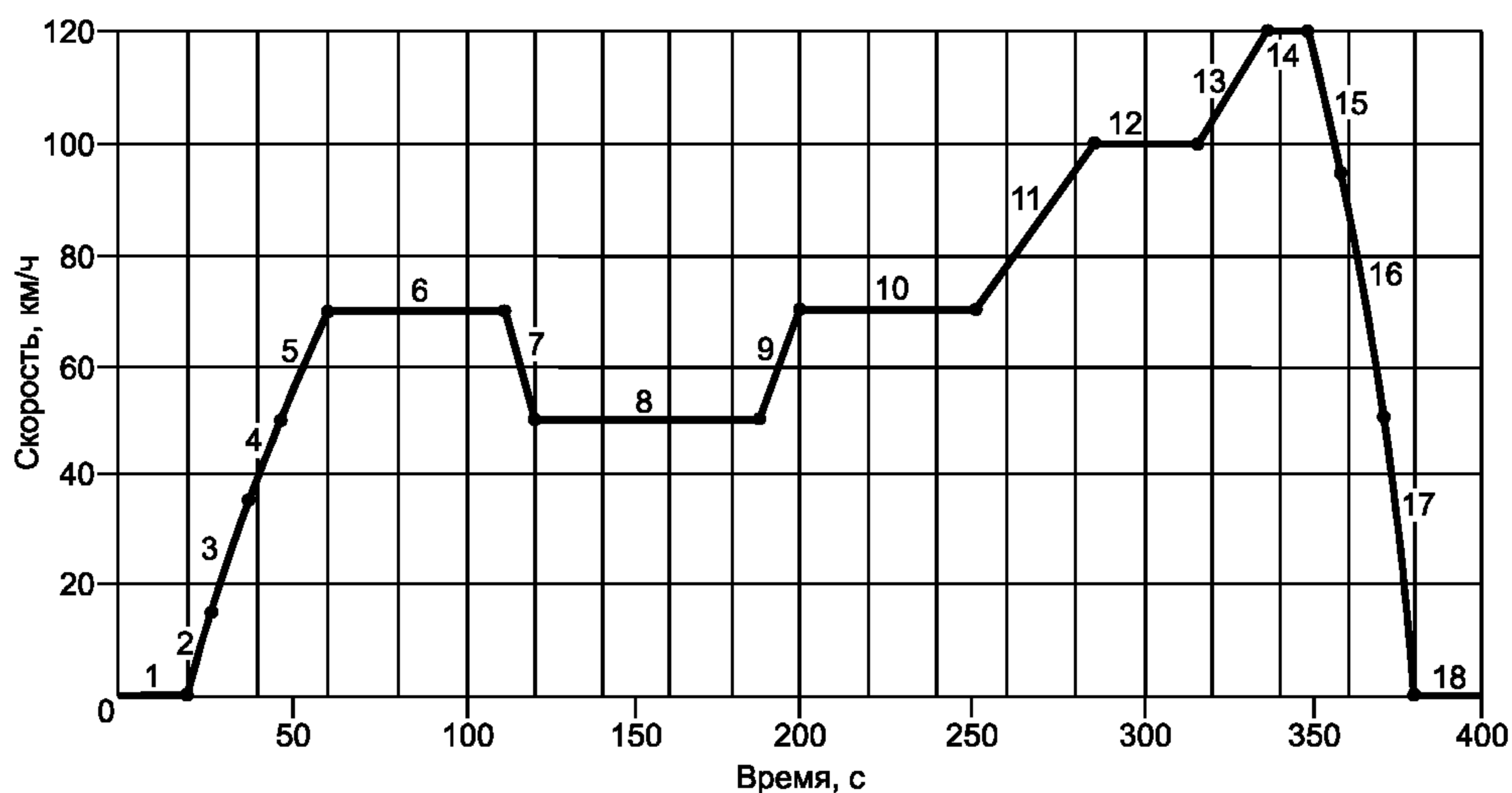
Рисунок 3 — Загородный цикл (400 с)
