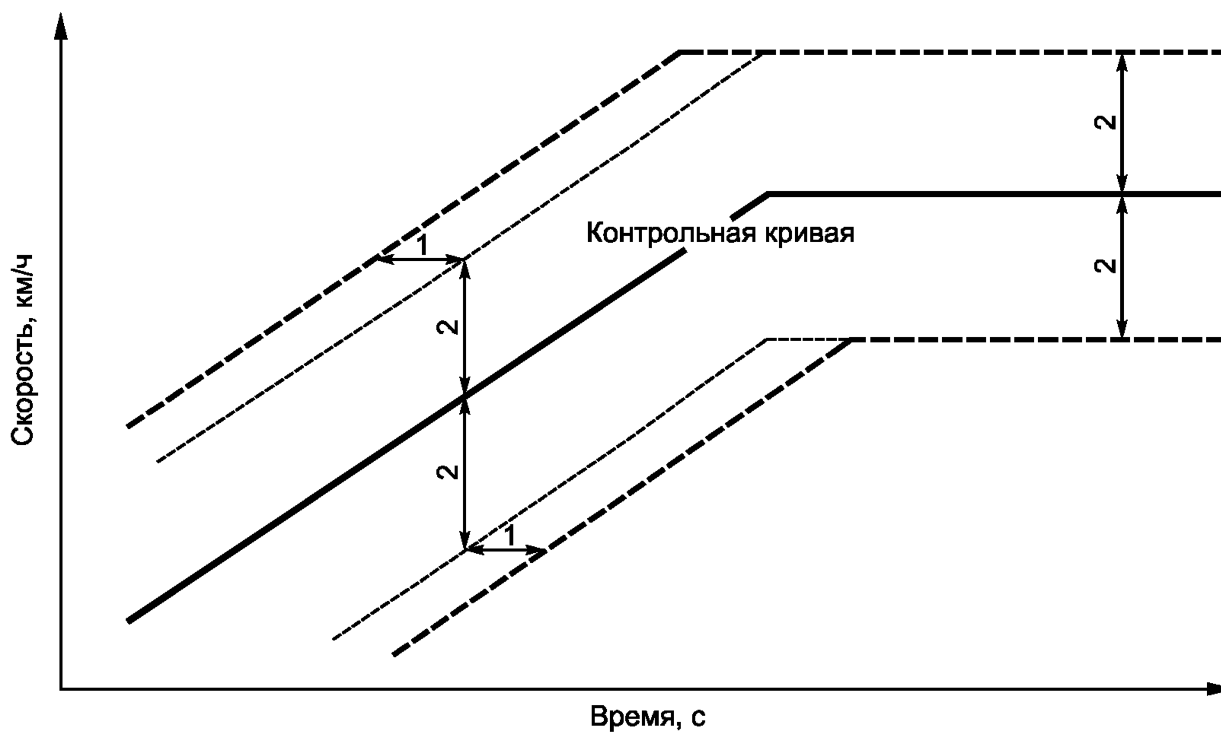
Рисунок 4 — Допустимое отклонение скорости
