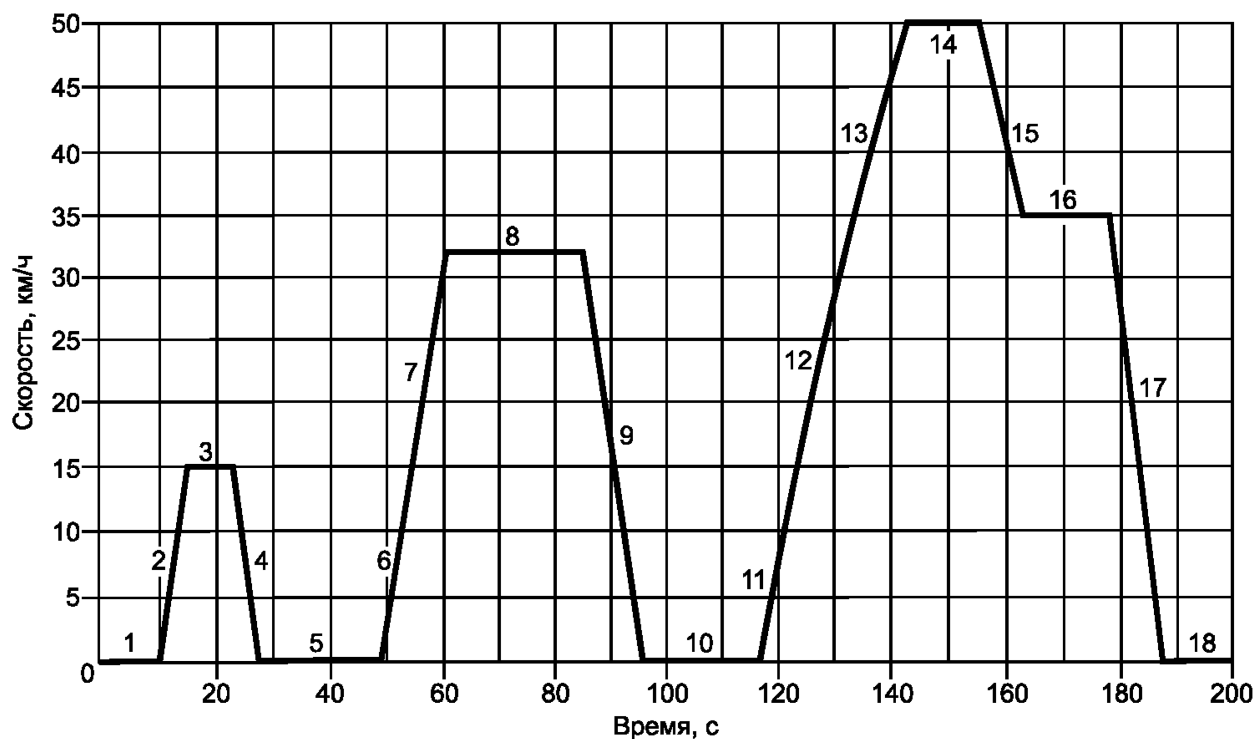
Рисунок 2 — Простой городской цикл (195 с)
