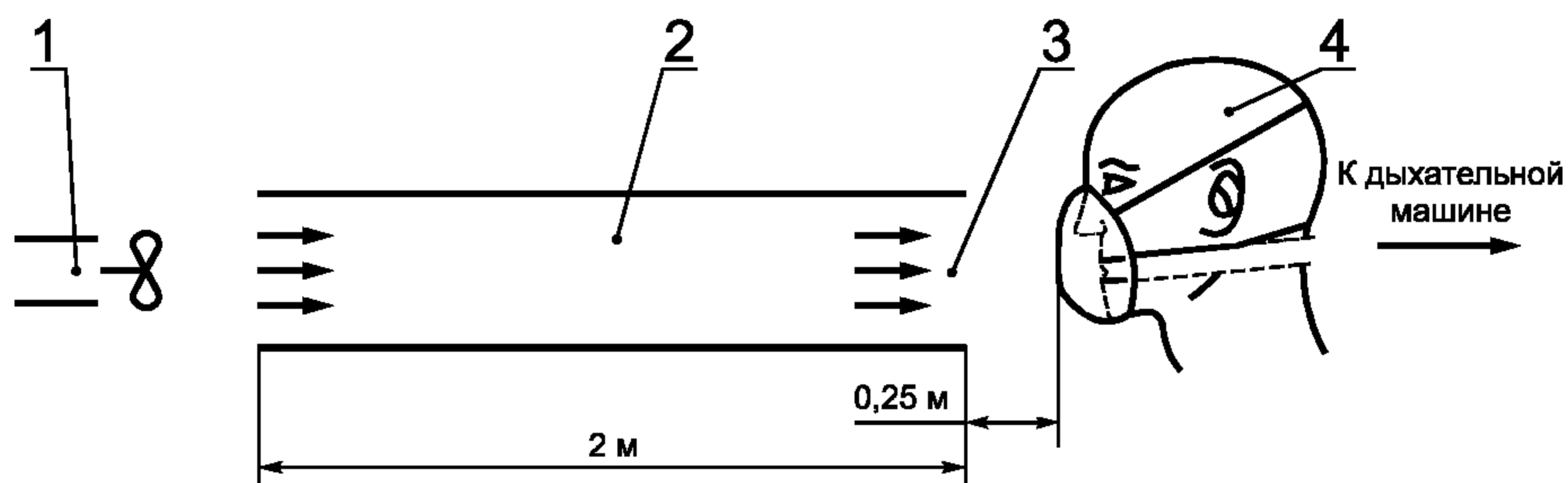
1 — вентилятор; 2 — трубопровод; 3 — датчик воздушного потока; 4 — голова манекена
