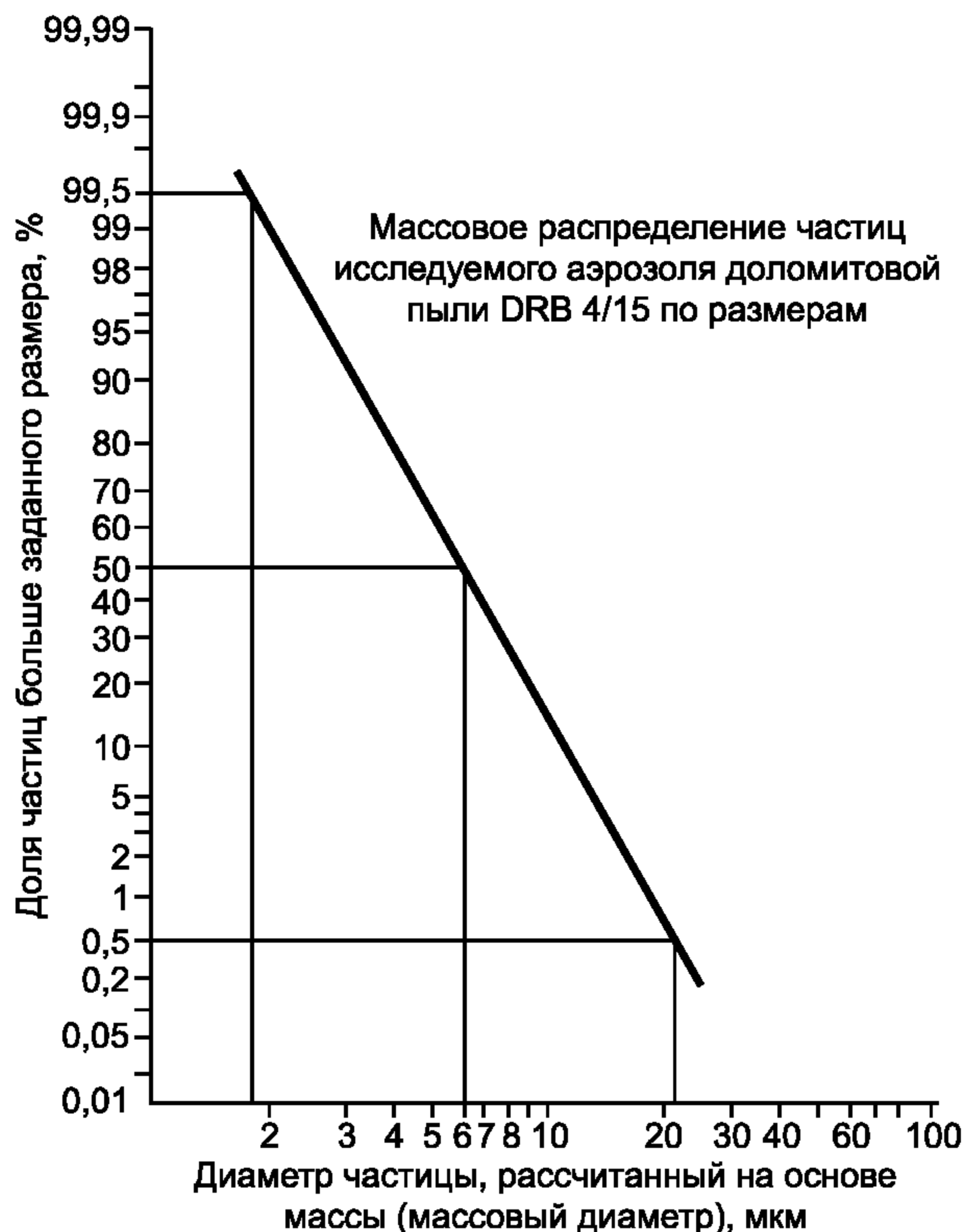
Рисунок 11 — Распределение частиц доломитовой пыли по размерам
