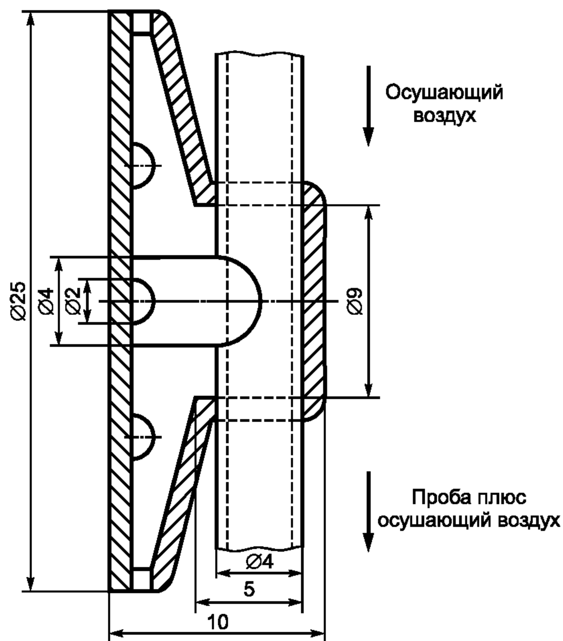
Рисунок 5 — Пробоотборник
