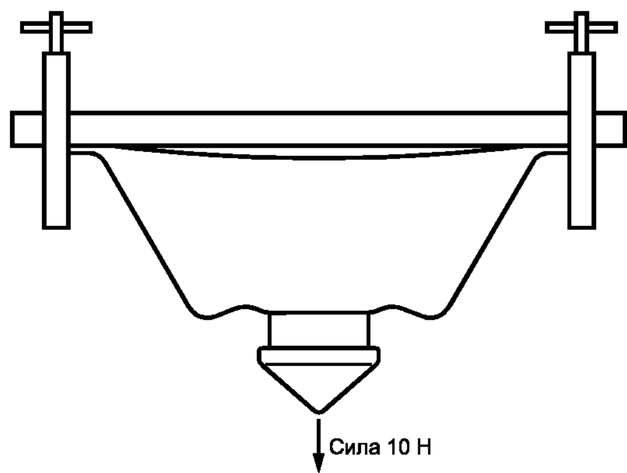
Рисунок 9 — Зажимное устройство для фильтрующей полумаски
