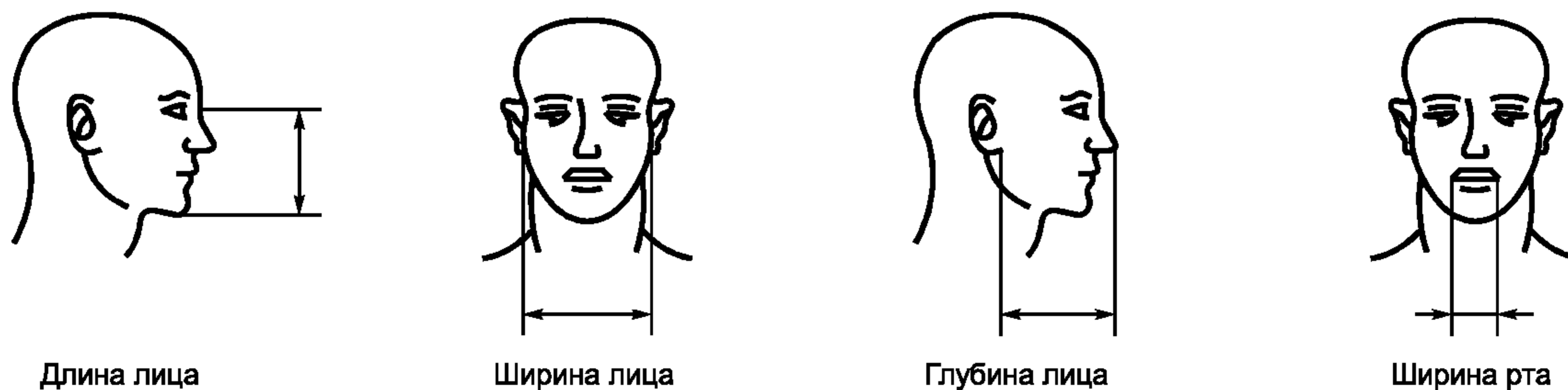
Рисунок 2 — Параметры лица
