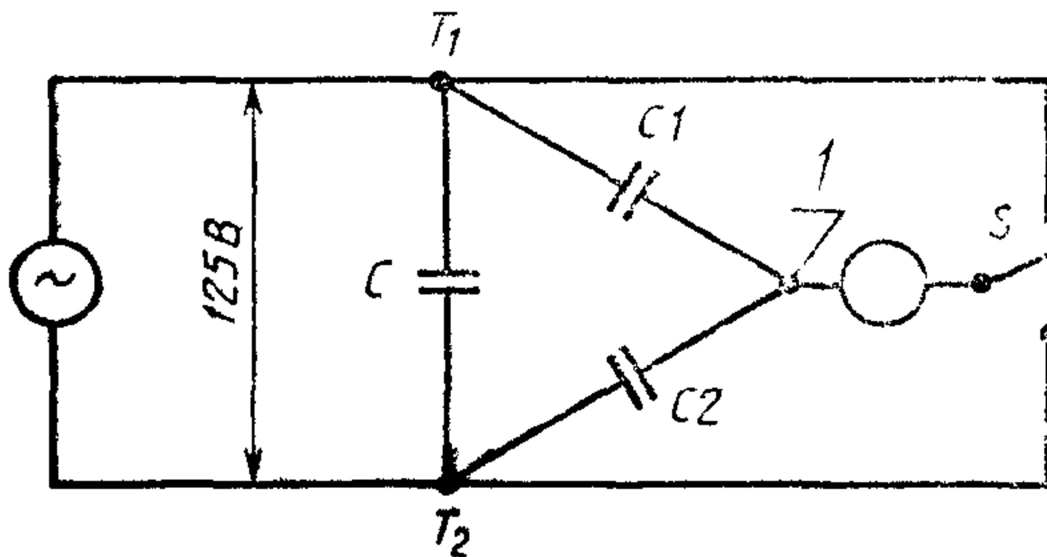
1 — корпус, T_1 и T_2 — выводы конденсатора. C — емкость конденсатора; C_1 и C_2 — паразитные емкости между каждым из электродов и корпусом. S — выключатель, A — микроамперметр
