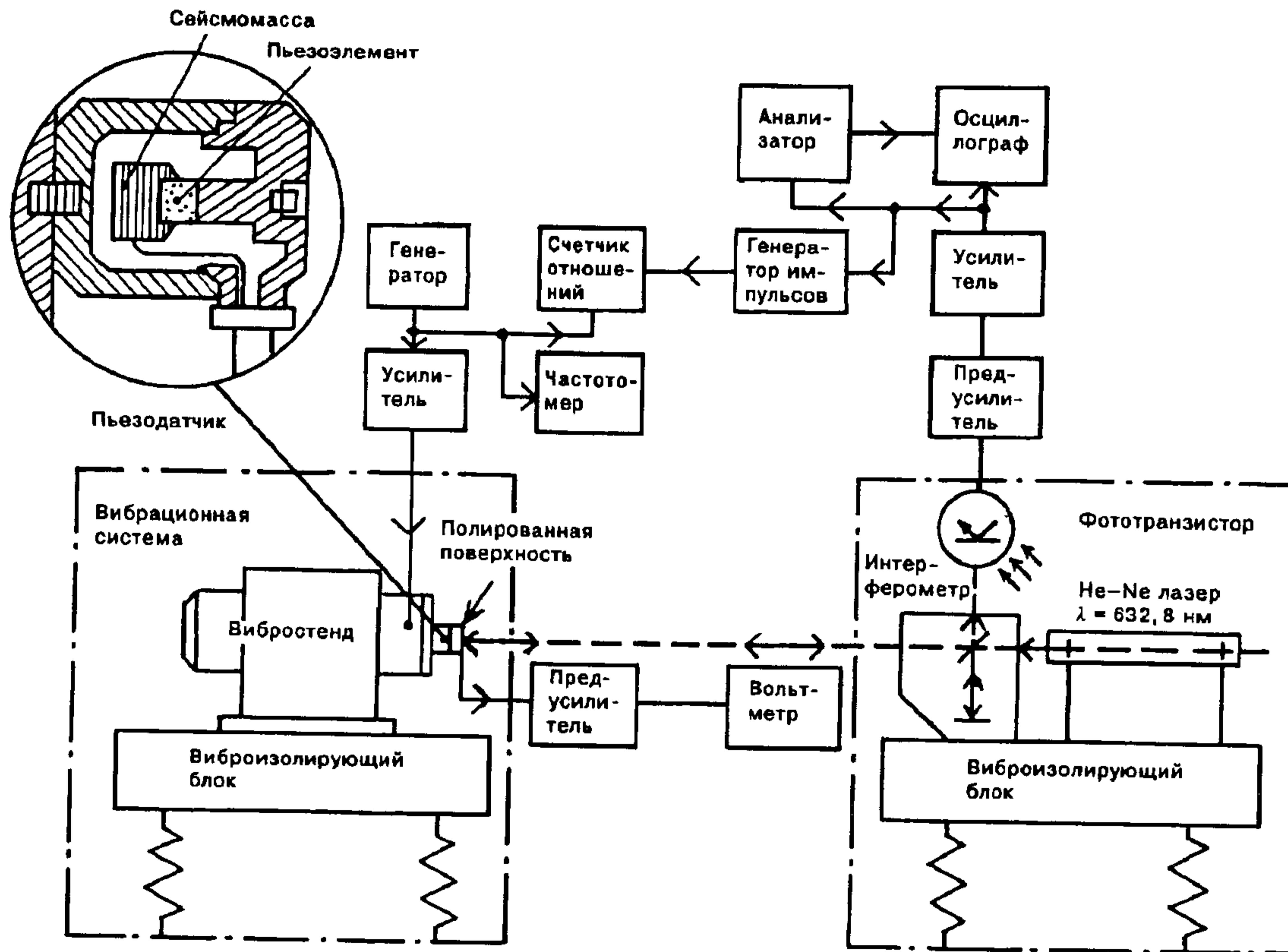
Рисунок 2 — Пример измерительной системы с использованием интерферометра
