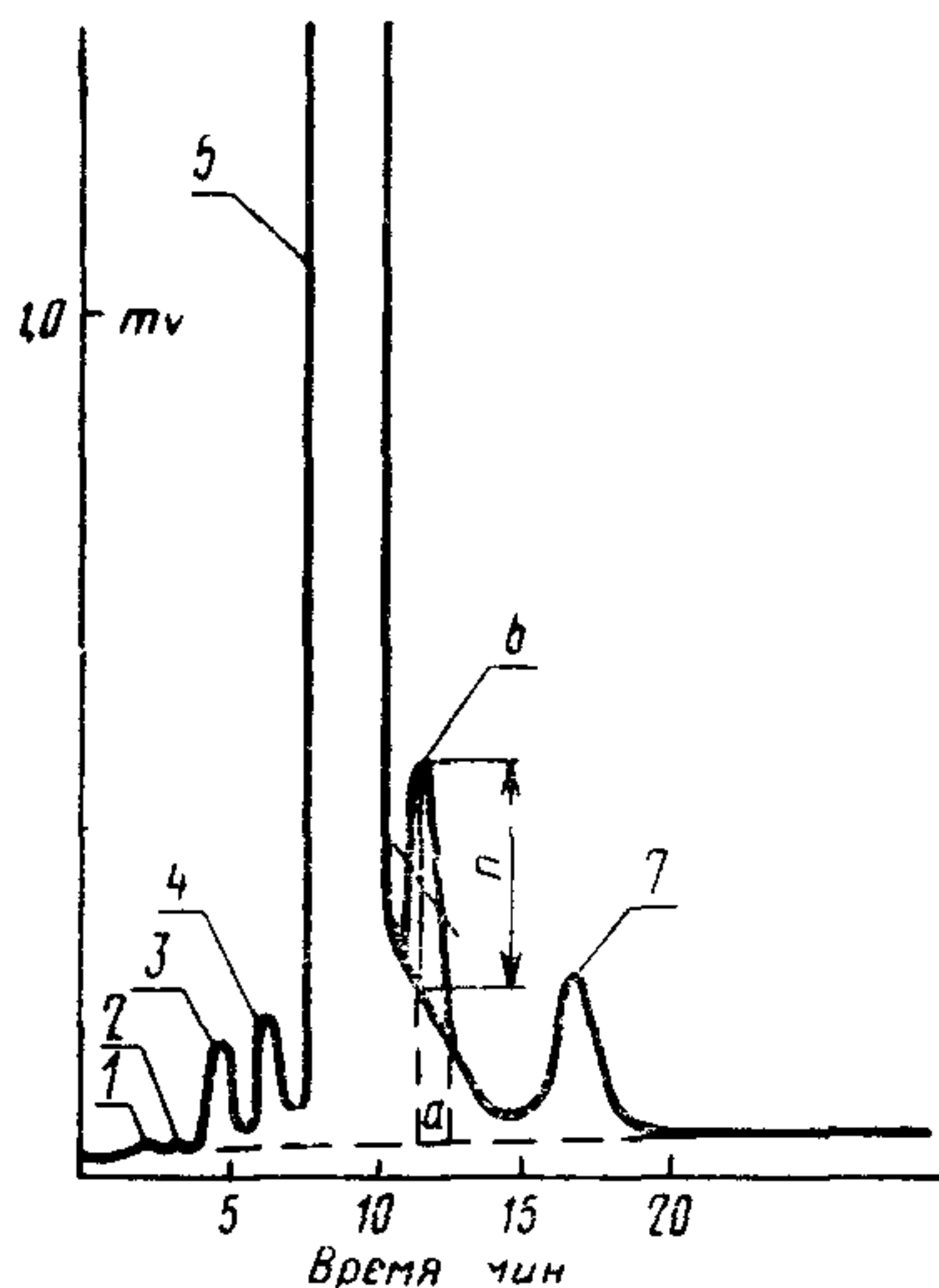
Типовая хроматограмма технического изобутилового спирта
