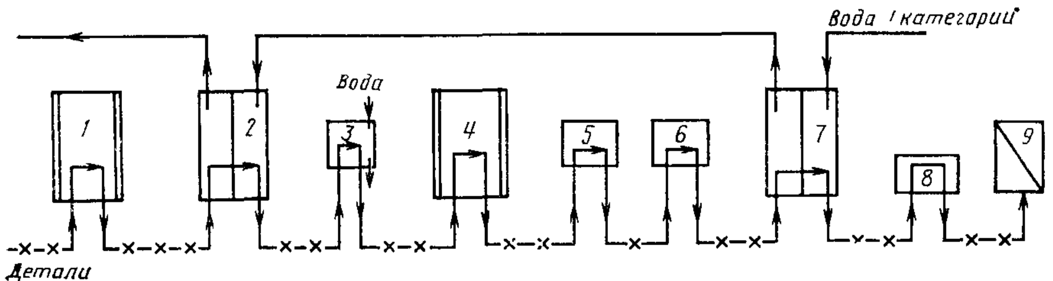
1 — ванна активации; 2, 7 — ванны промывки; 3 — ванна финишной промывки водой III категории (непроточная или циркулирующая); 4 — ванна нанесения покрытий драгметаллами; 5, 6 — ванны-уловители с водой III категории; 8 — обдув сжатым воздухом или центрифугирование; 9 — термосушка
