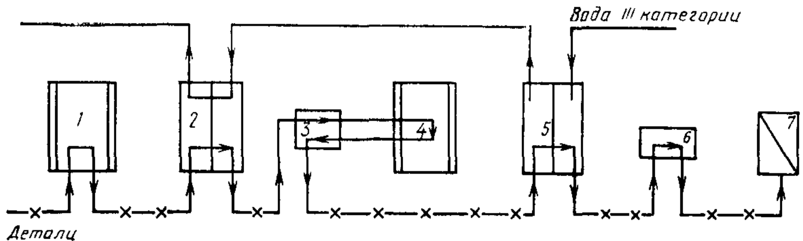
1 — ванна активации; 2, 5 — ванны промывки; 3 — ванны улавливания с водой III категории; 4 — ванна нанесения покрытий; 6 — обдув сжатым воздухом или центрифугирование; 7 — сушка (термосушка)
