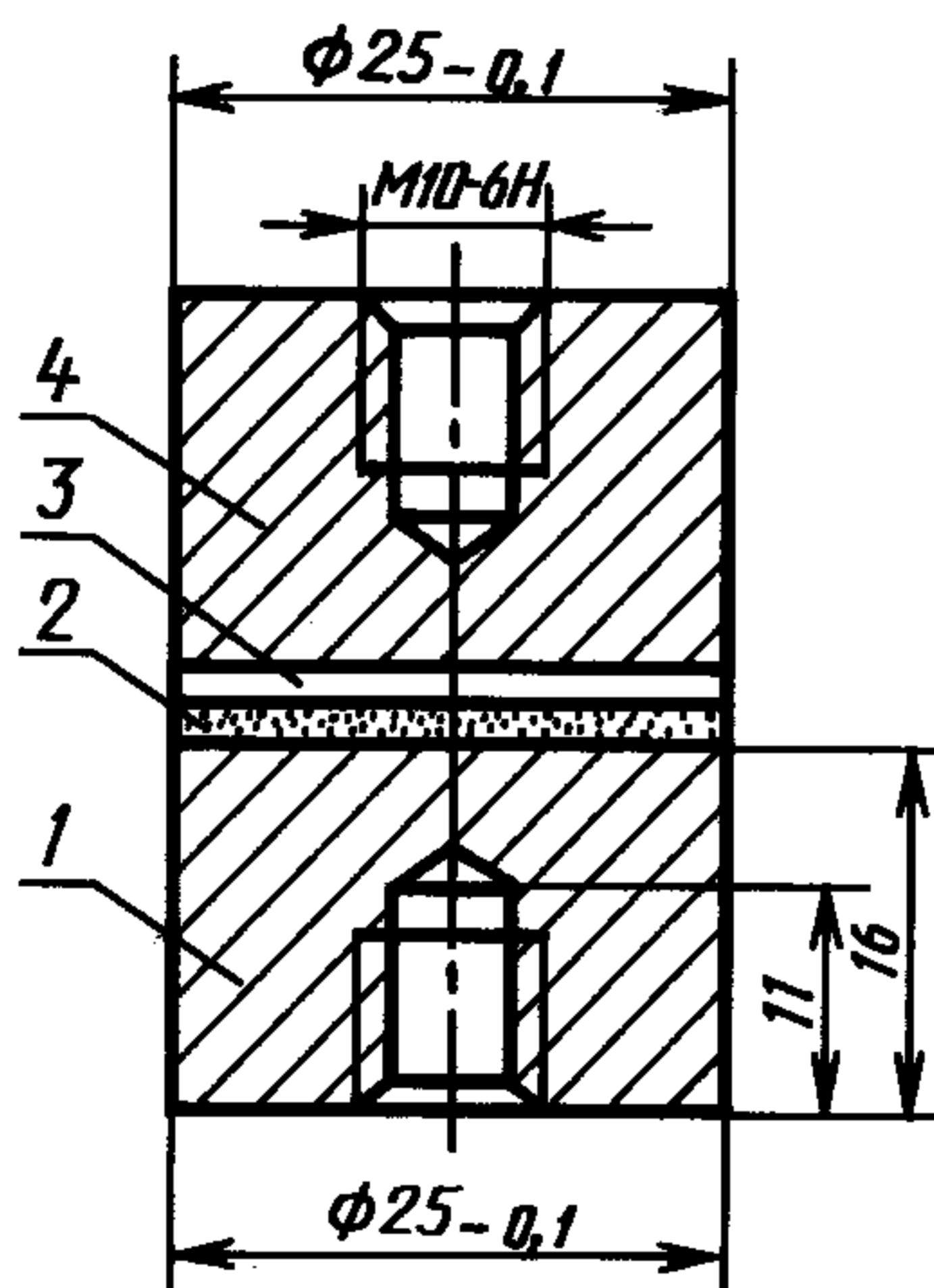
1 — образец; 2 — покрытие; 3 — клеевая прослойка; 4 — контрообразец
