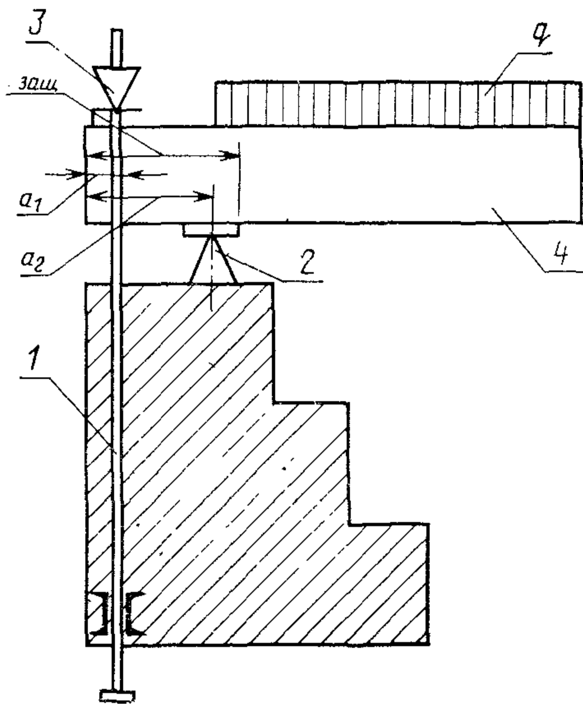
Схема испытания конструкций, работающих как консоль
