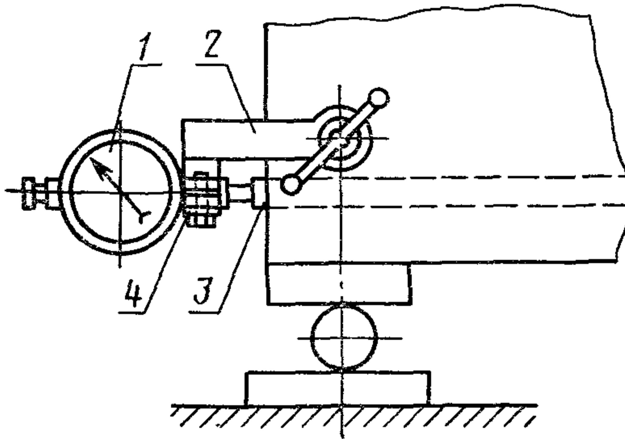
Схема измерения смещения концов арматуры индикаторами
