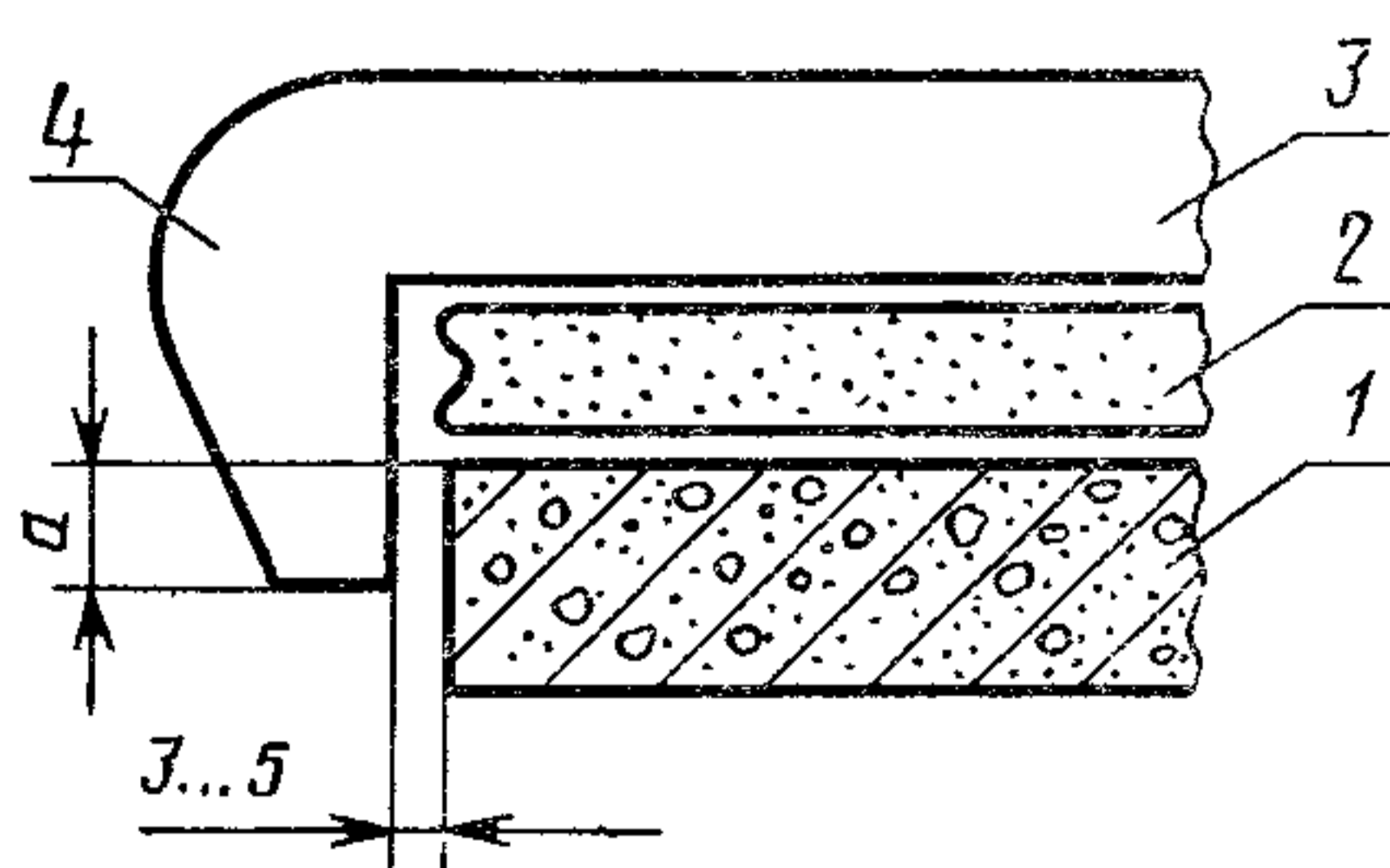
Схема испытания конструкций сжатым воздухом
