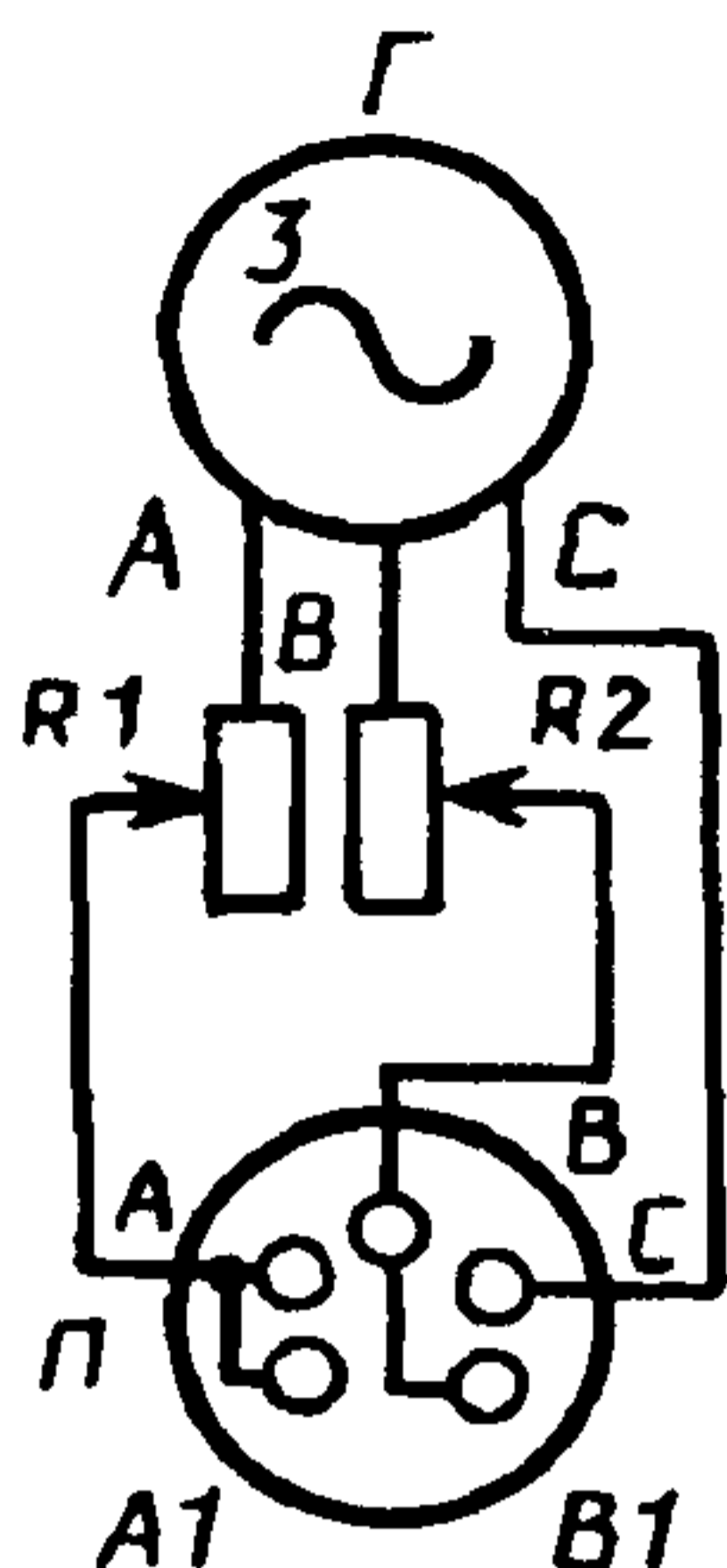
Г — генератор трехфазного напряжения; R1, R2 — переменные резисторы; П — проверяемый синхроскоп.
