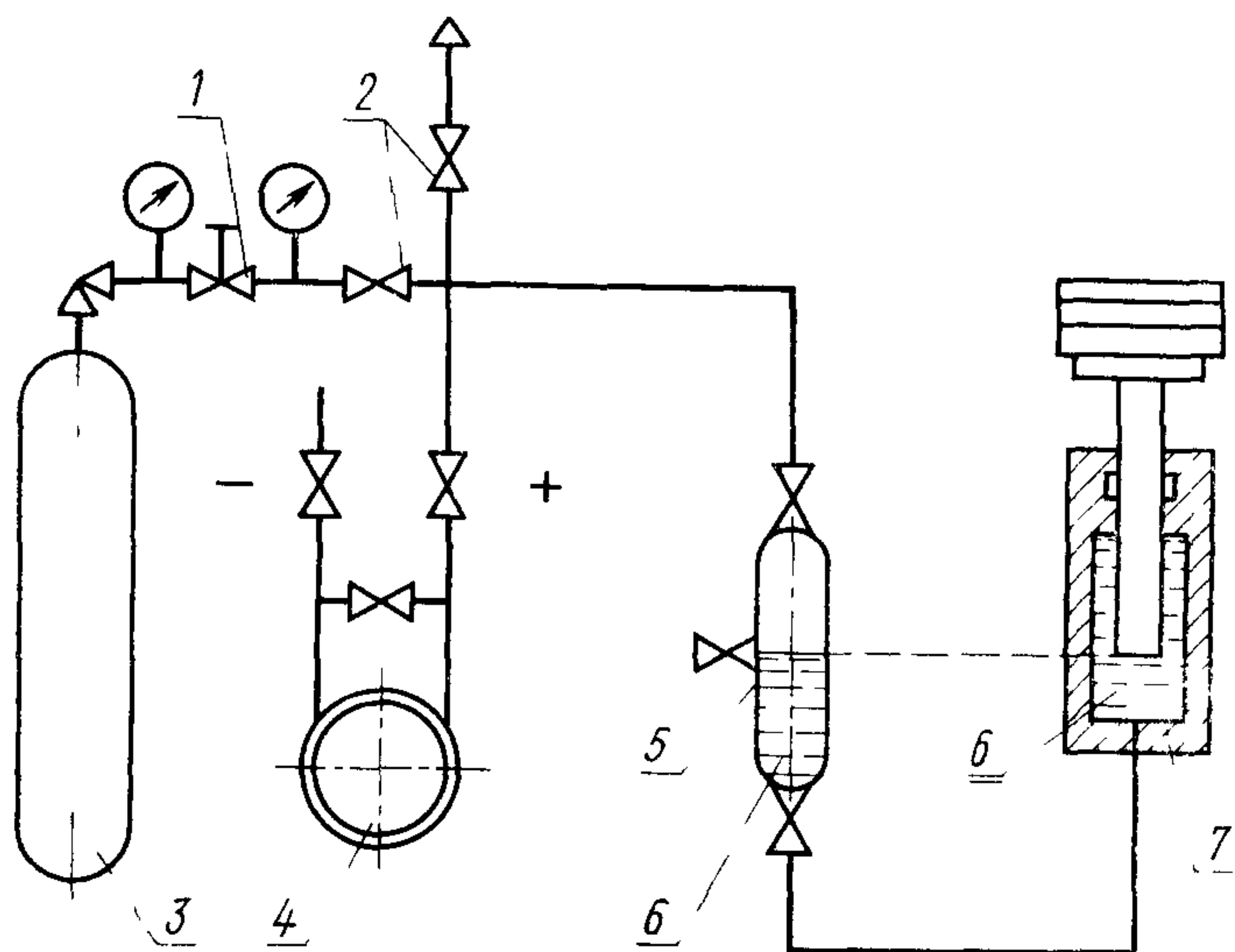
1—редуктор; 2—запорный вентиль; 3—баллон со сжатым азотом, 4—поверяемый преобразователь; 5—разделительный сосуд; 6—рабочая жидкость; 7—грузопоршневой манометр
