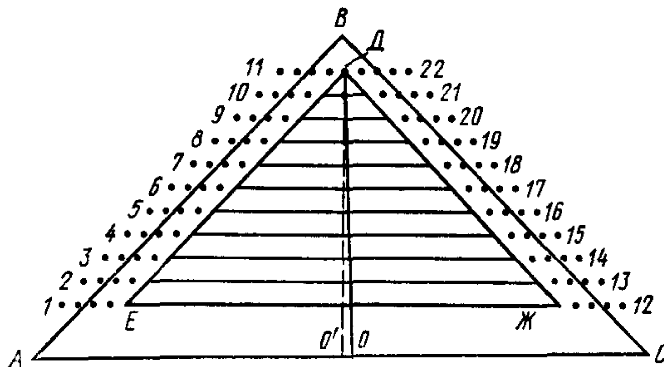
Схема отбора из конической насыпи
