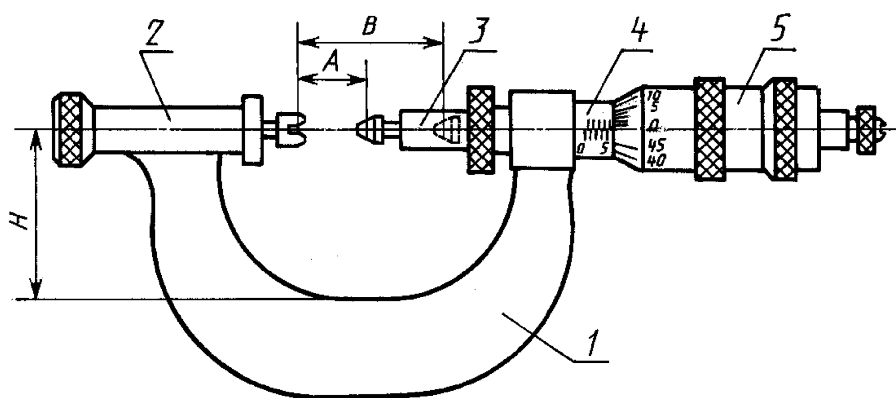
Микрометры типов МВМ, МВТ, МВП
