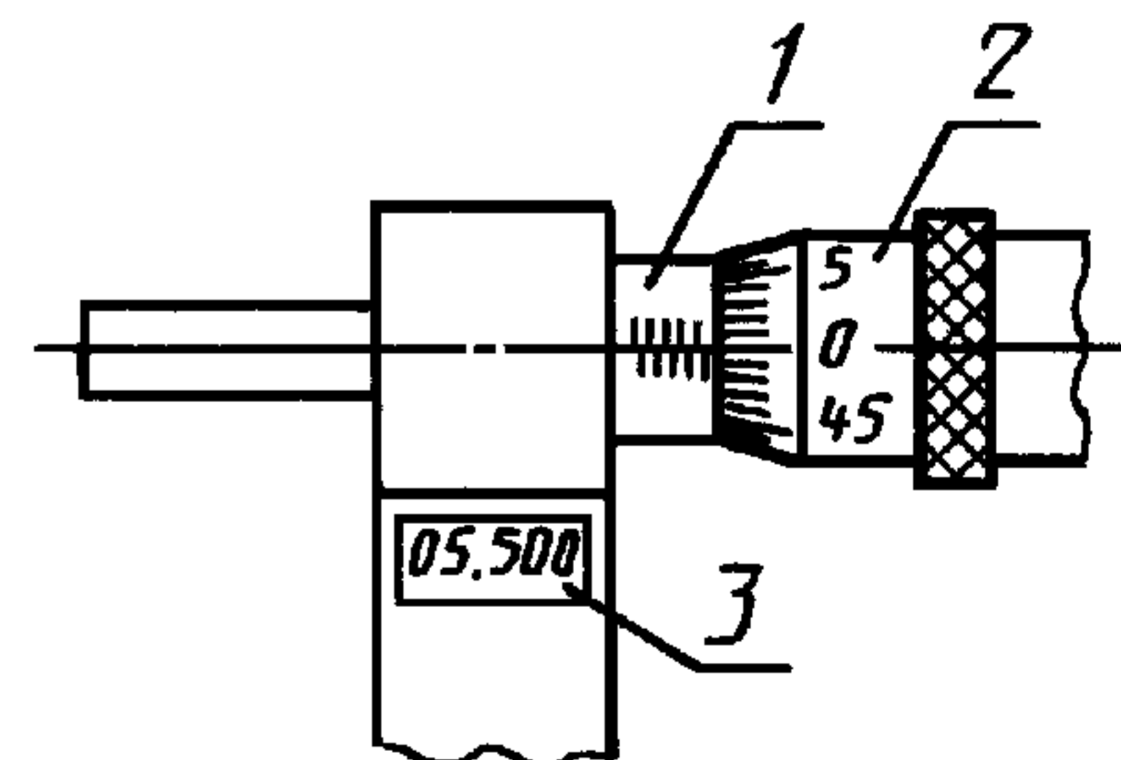
Цифровое устройство микрометров типов МВМЦ, МВТЦ, МВПЦ
