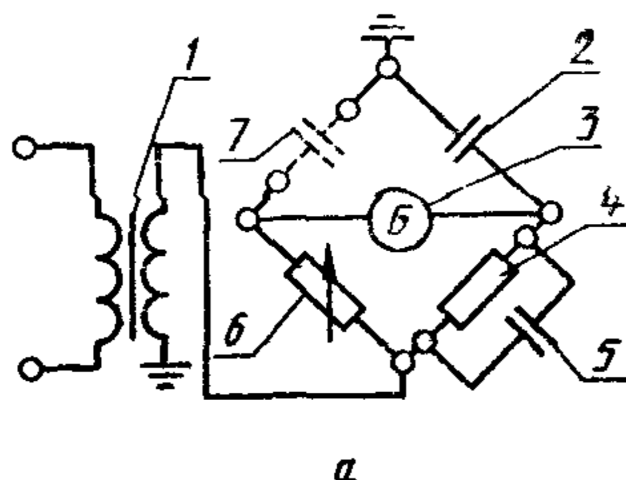
Схема с заземленной диагональю
