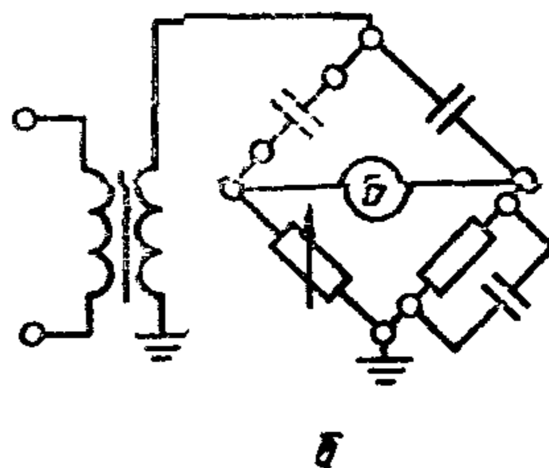
Схема с заземленной диагональю
