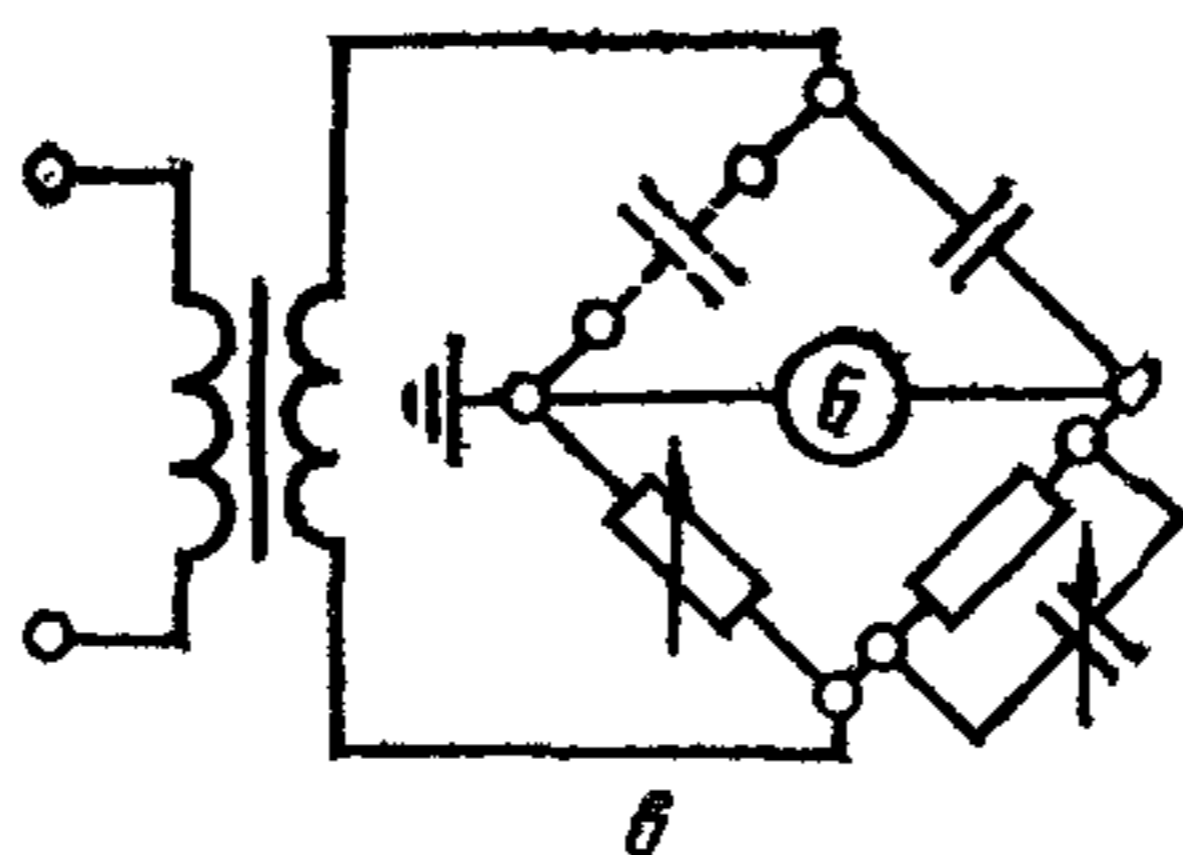
Схема с заземленной диагональю
