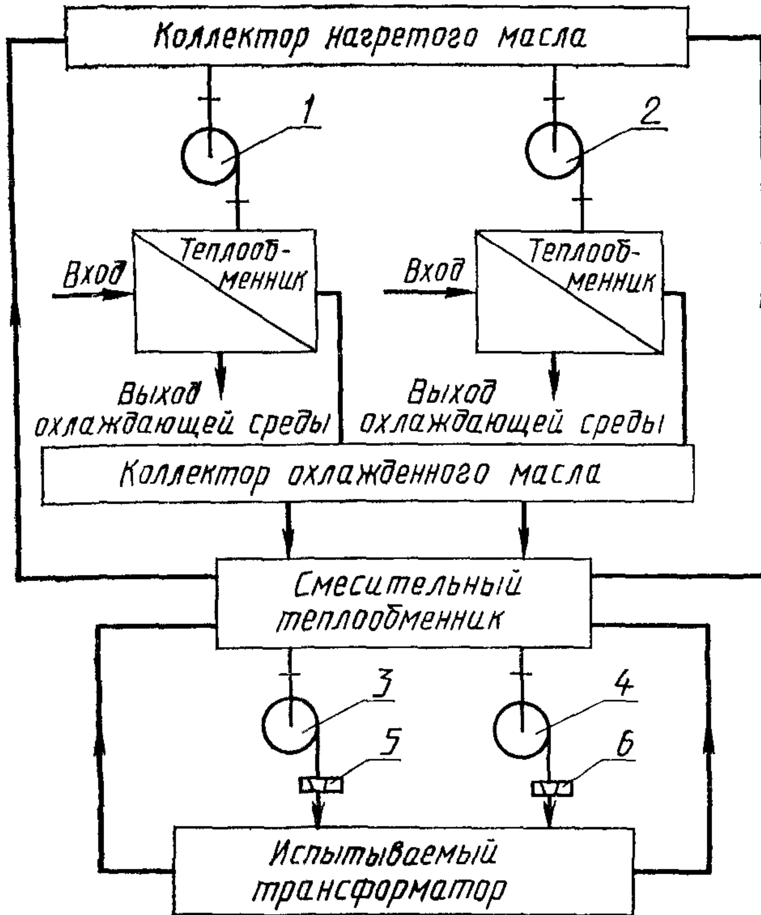
1, 2 — насосы испытательной системы охлаждения; 3, 4 — насосы, обеспечивающие циркуляцию масла; 5, 6 — измерительные диафрагмы
