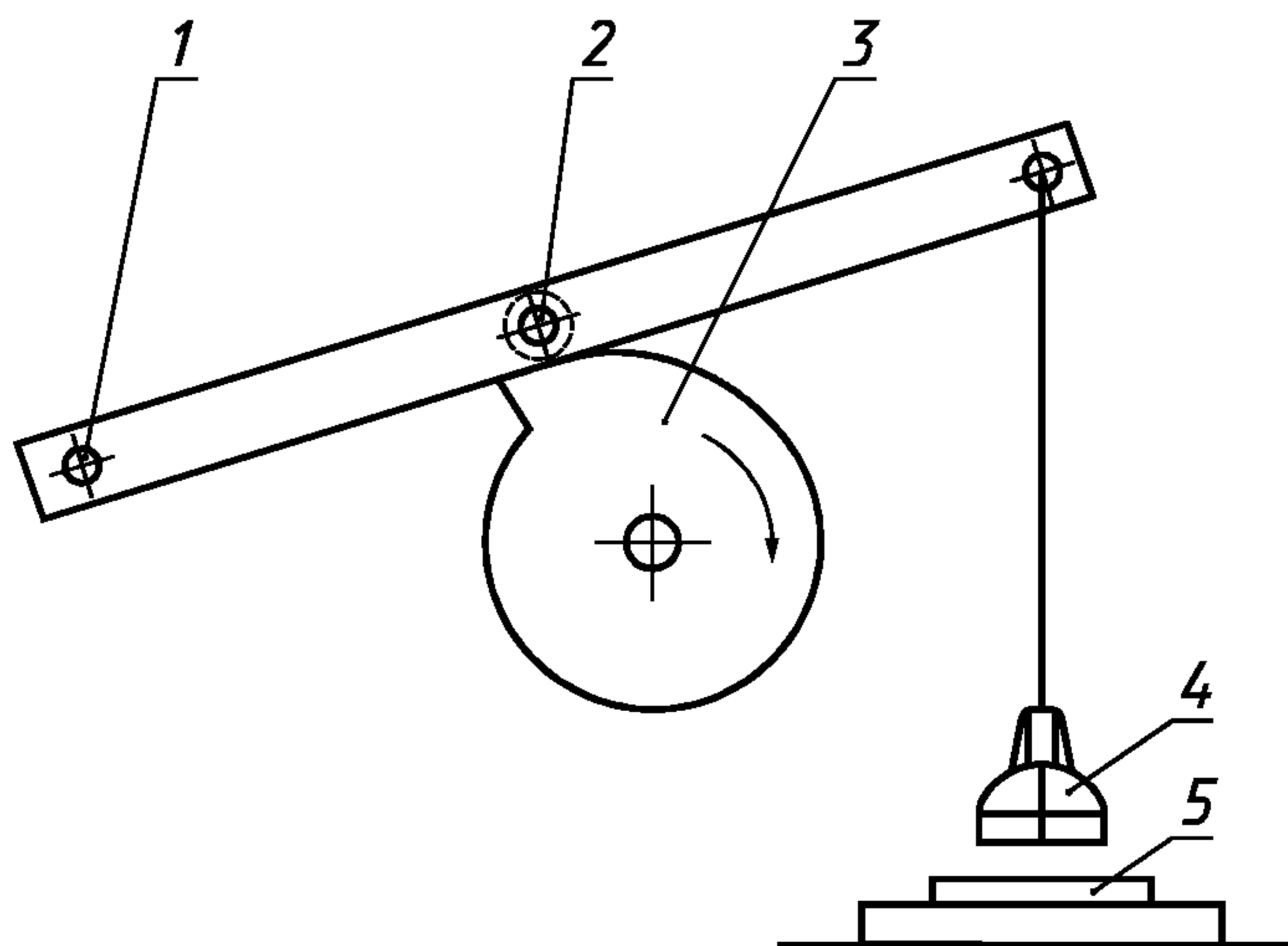
Схема установки проверки механической прочности
