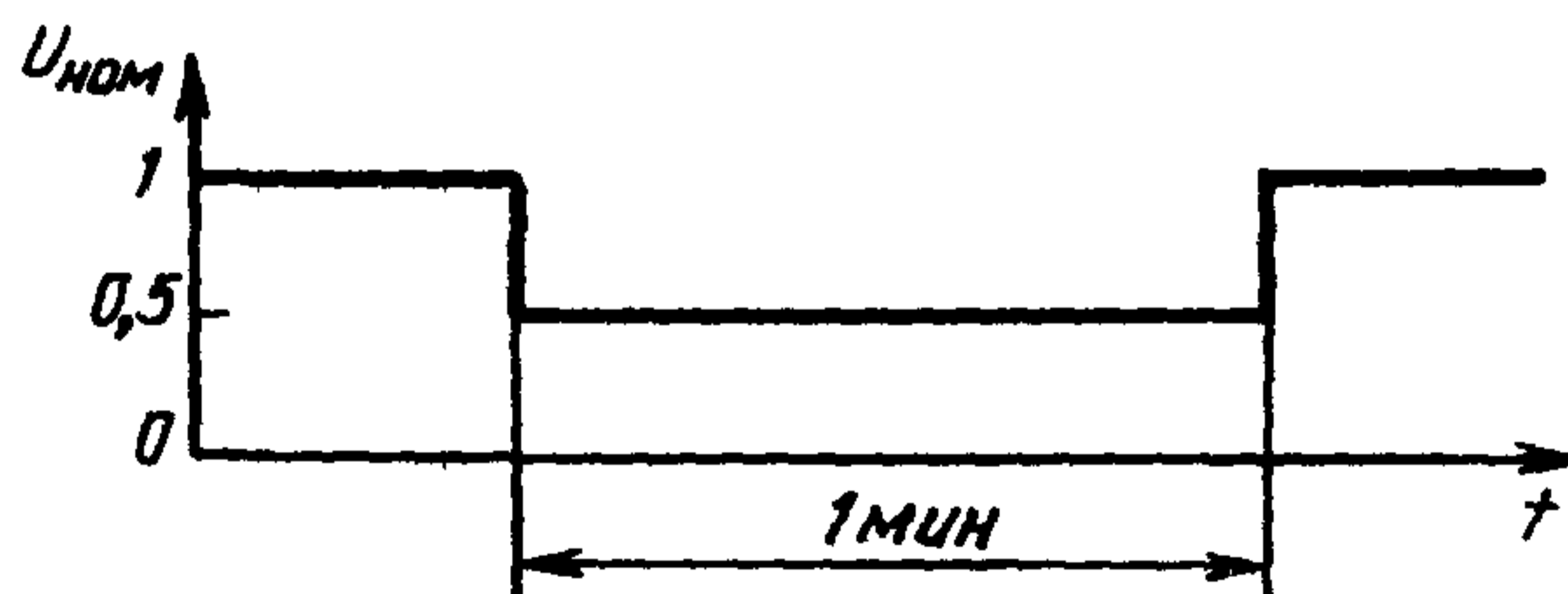
Рисунок 3 — Провалы напряжения \Delta U = 50\%
