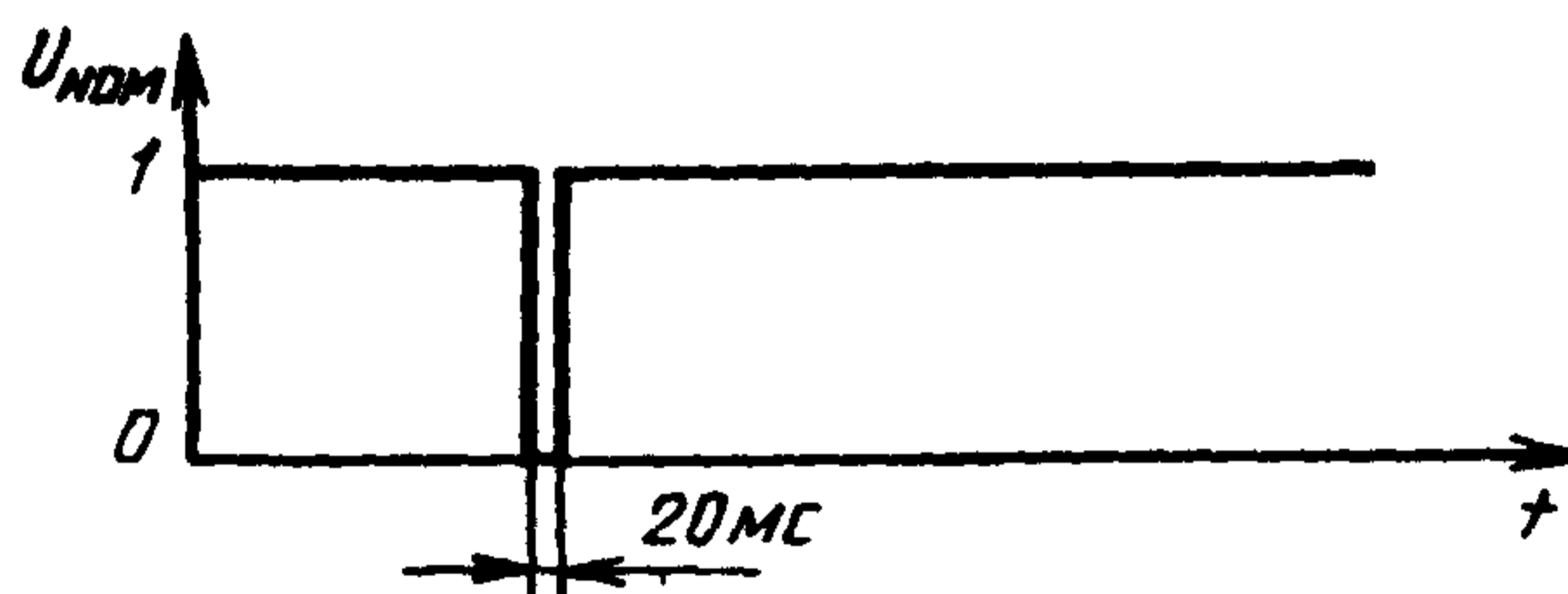
Рисунок 2 — Прерывания напряжения \Delta U = 100\% , 20 мс
