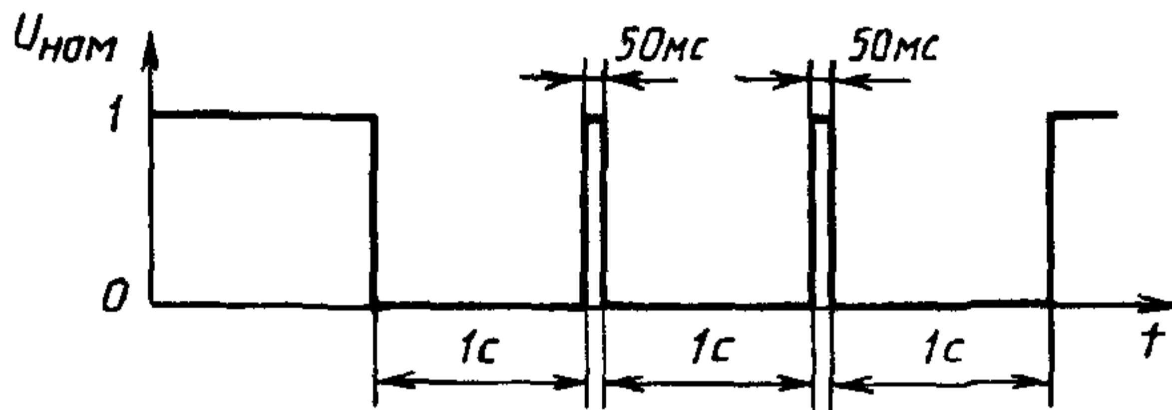
Рисунок 1 — Прерывания напряжения \Delta U=100\% , 1 с
