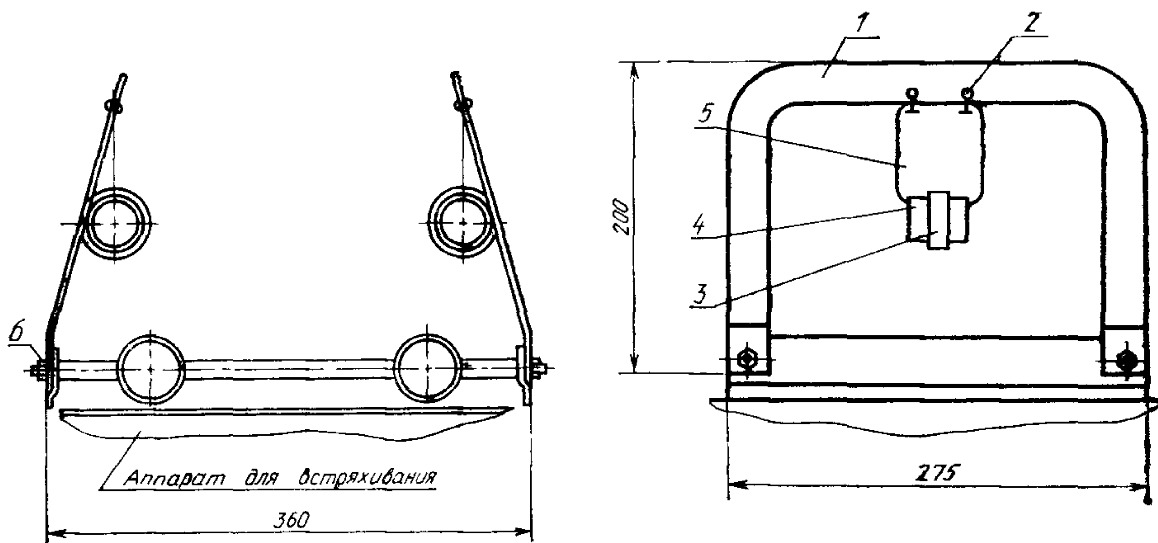
1—стойка, 2, 3—кольца, 4—груз; 5—проволока; 6—гайка
