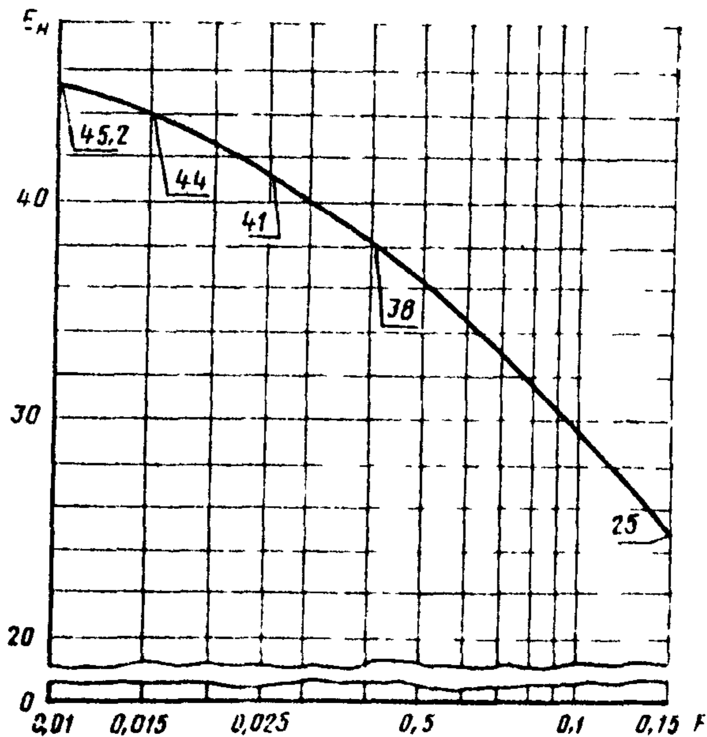
E_{н} — напряженность поля радиопомех, дБ, F — частота, МГц
