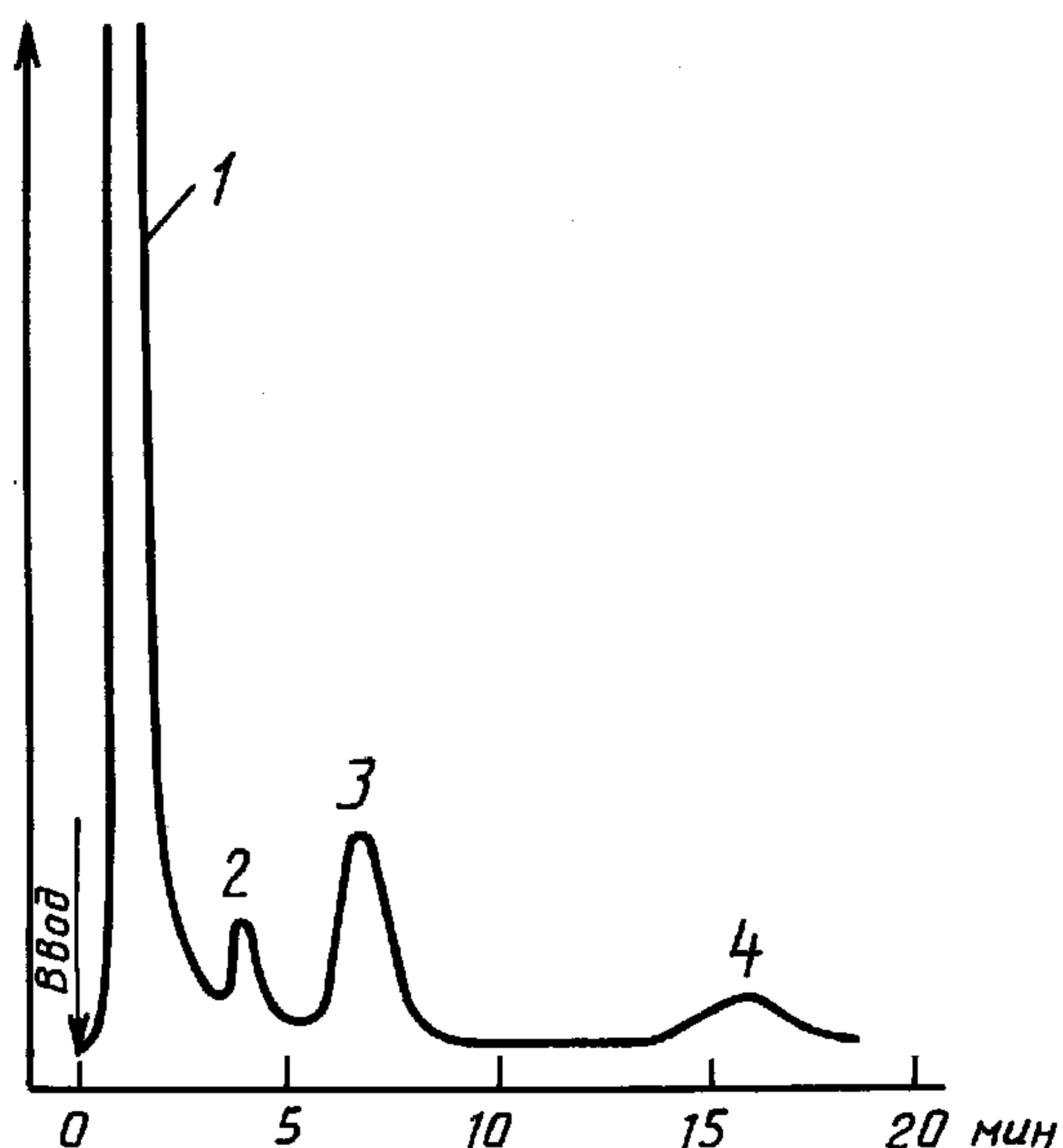
Типовая хроматограмма этиленгликоля с использованием колонки I
