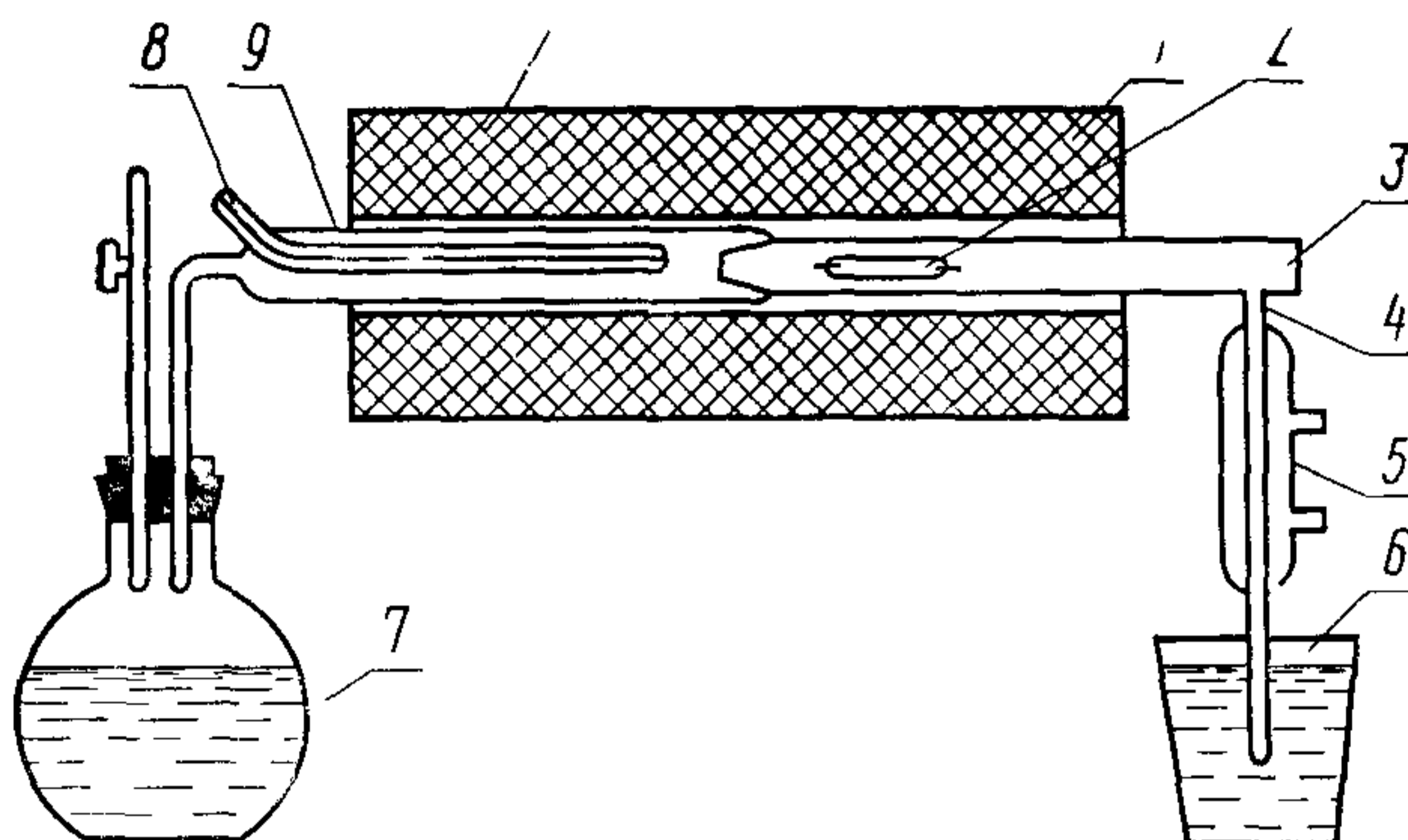
Схема пирогидролитической установки
