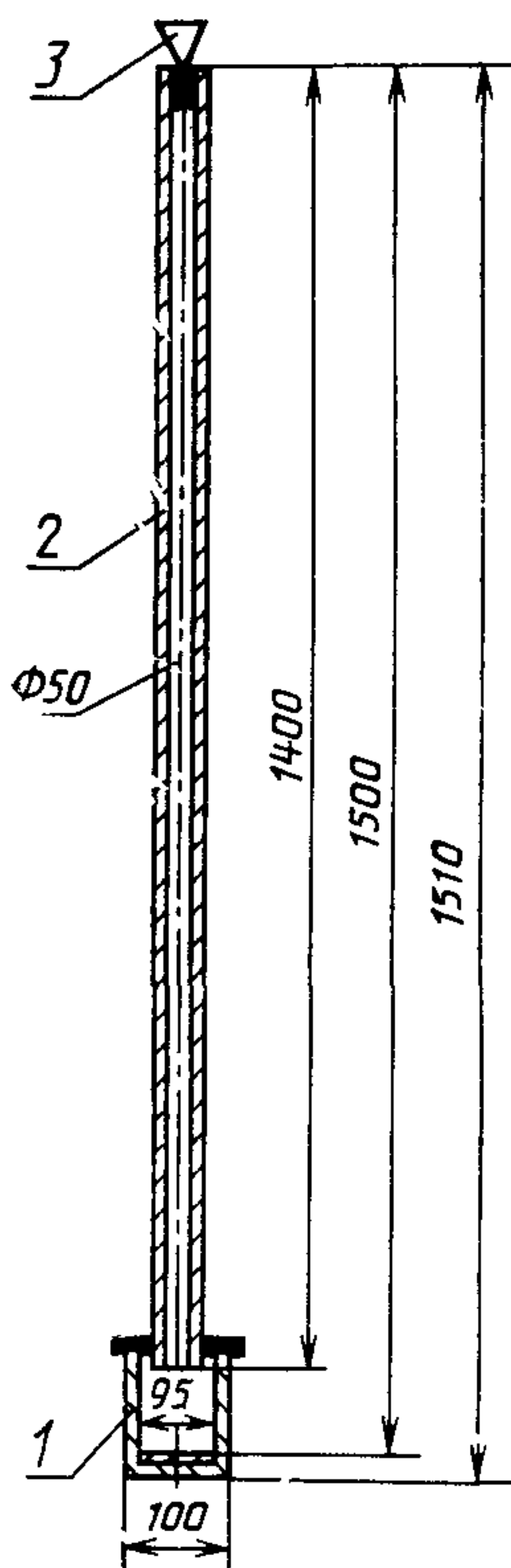
1—приемный стакан 2— труба, 3—воронка
