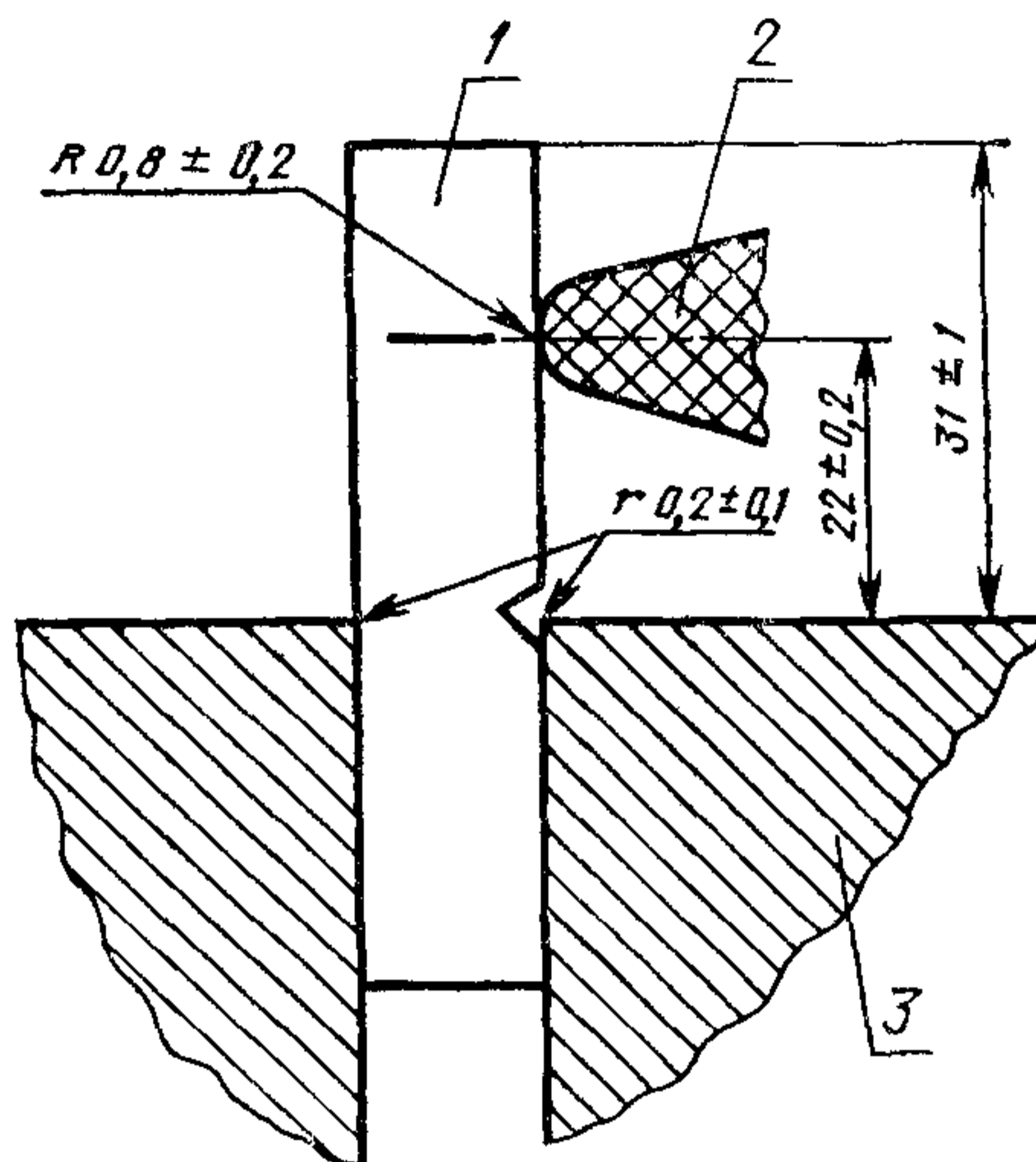
1 — образец; 2 — маятник; 3 — зажим
