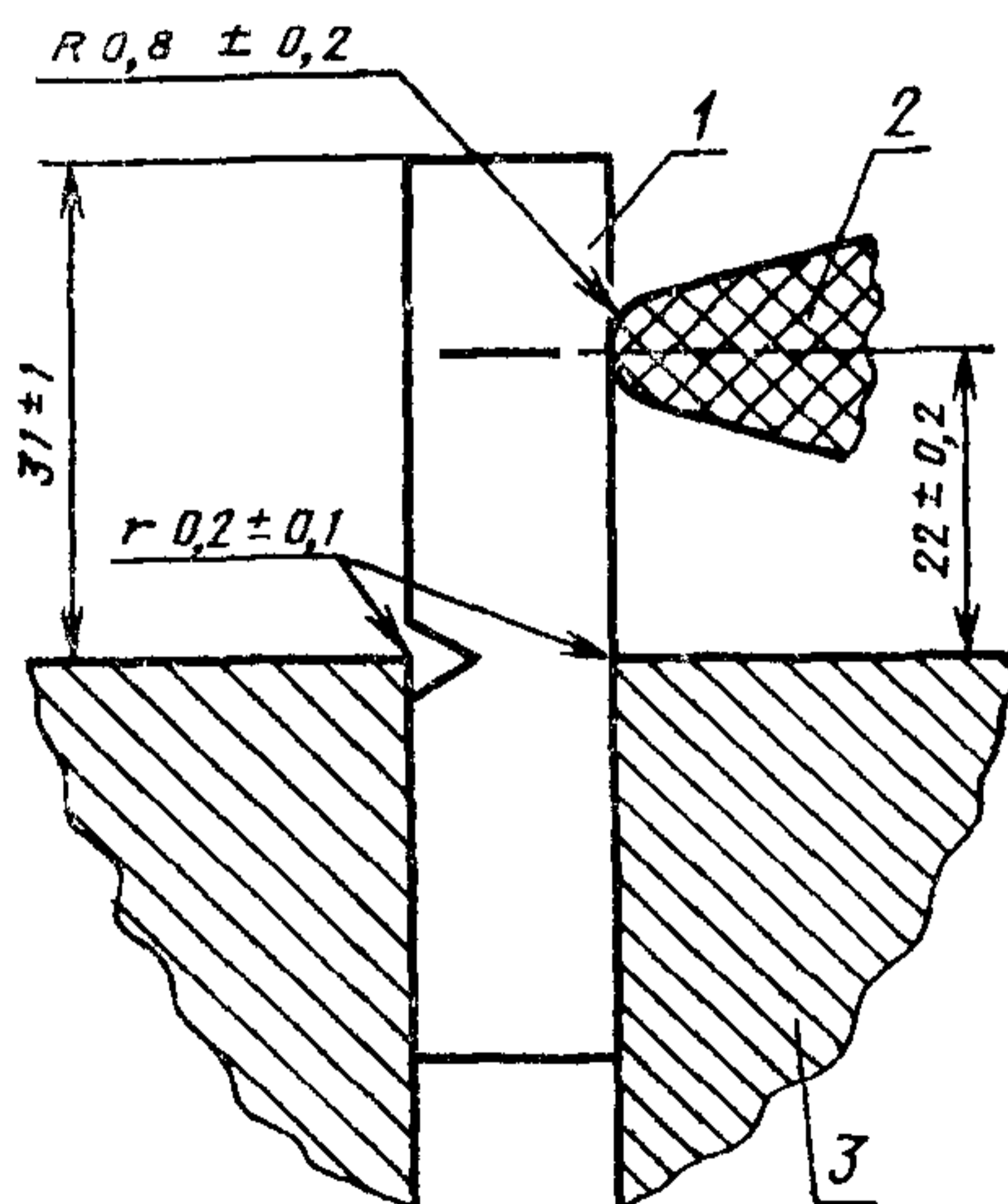
1 — образец; 2 — маятник; 3 — зажим
