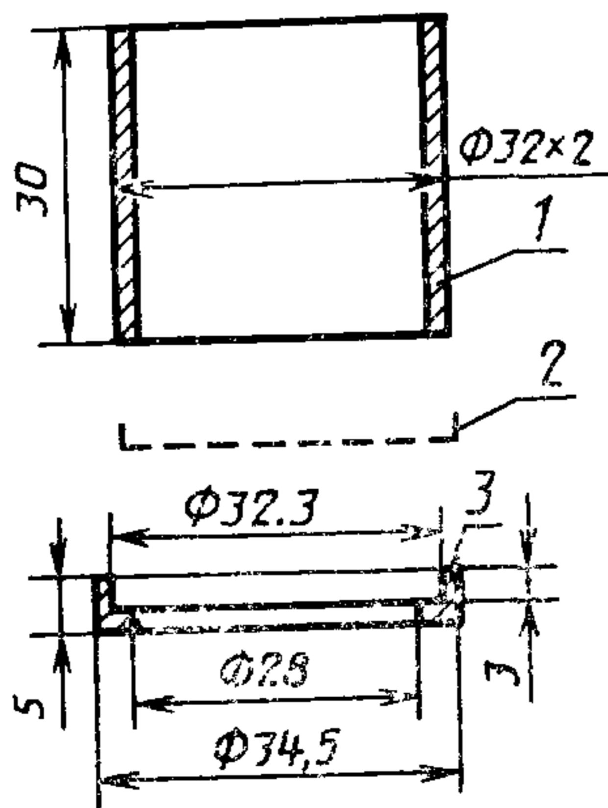
1—трубка; 2—фильтр; 3—зажимное кольцо
