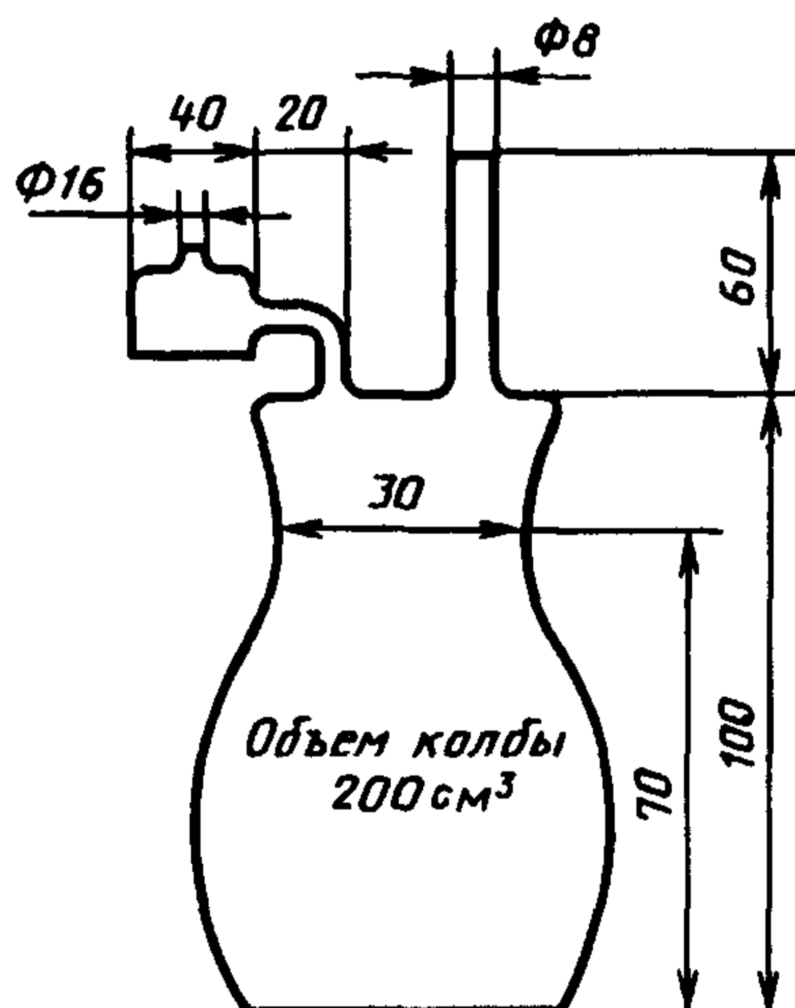
Реакционная колба
