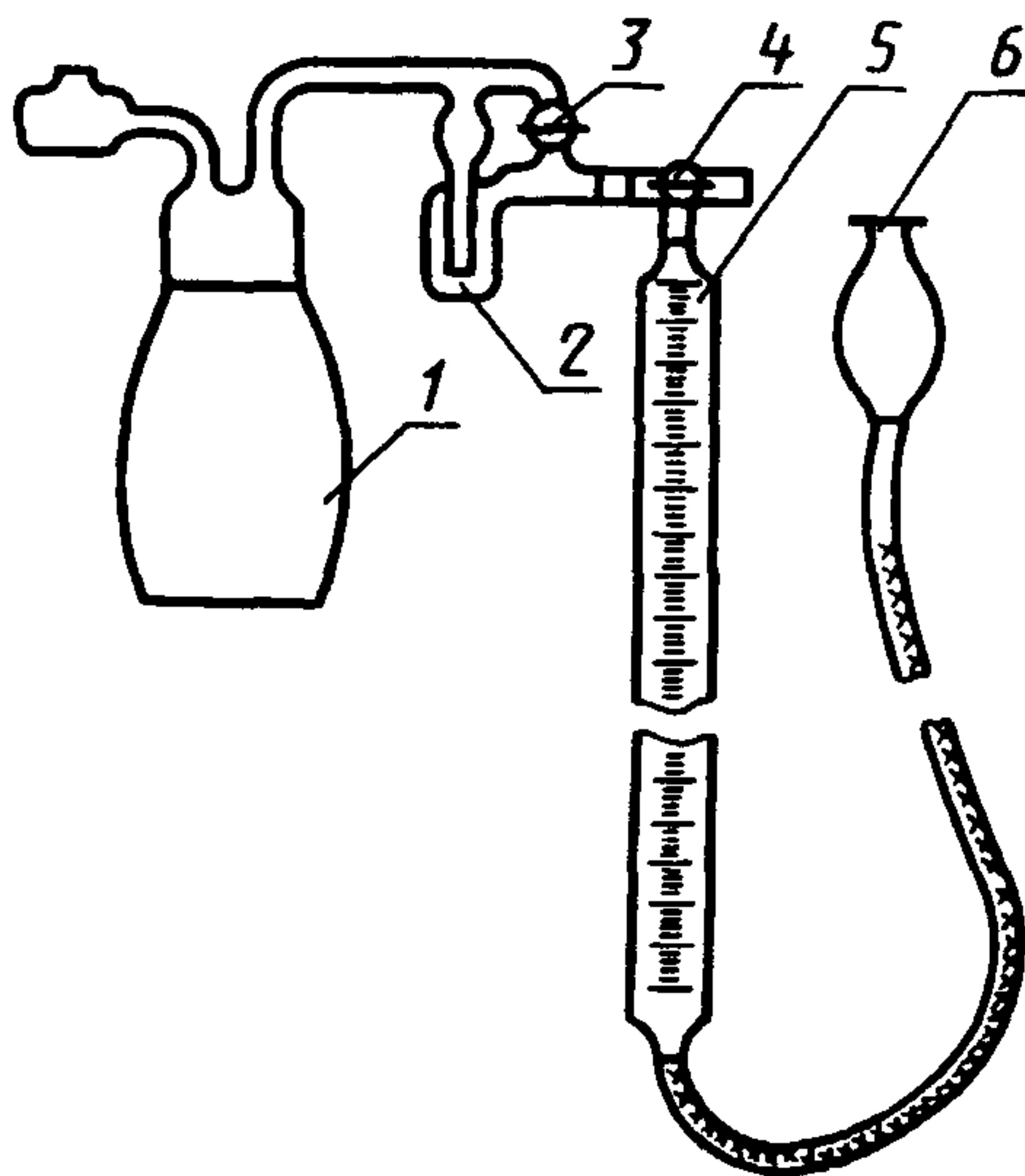
Прибор для определения массовой доли воды
