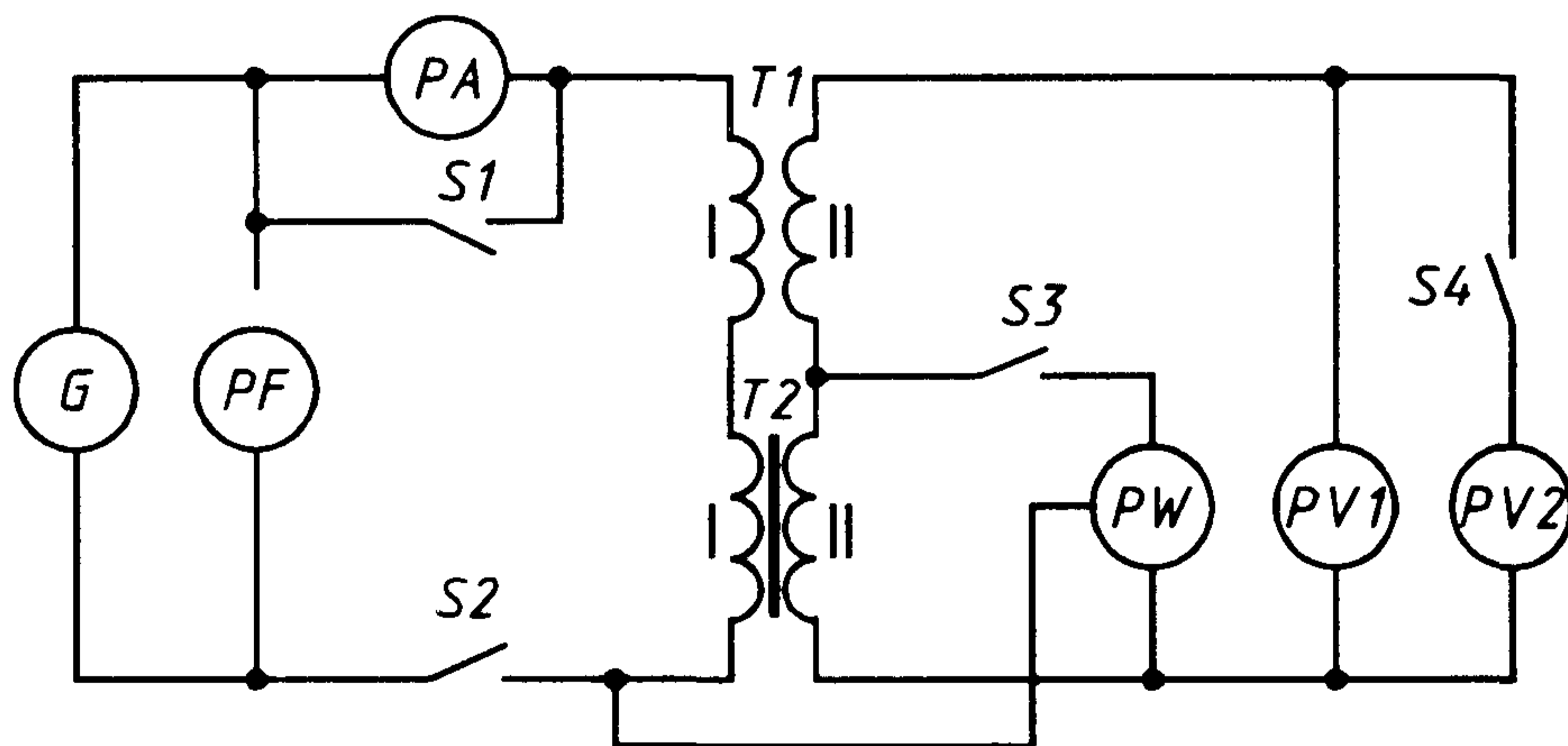
Рисунок 1 — Схема для измерений ваттметровым методом
