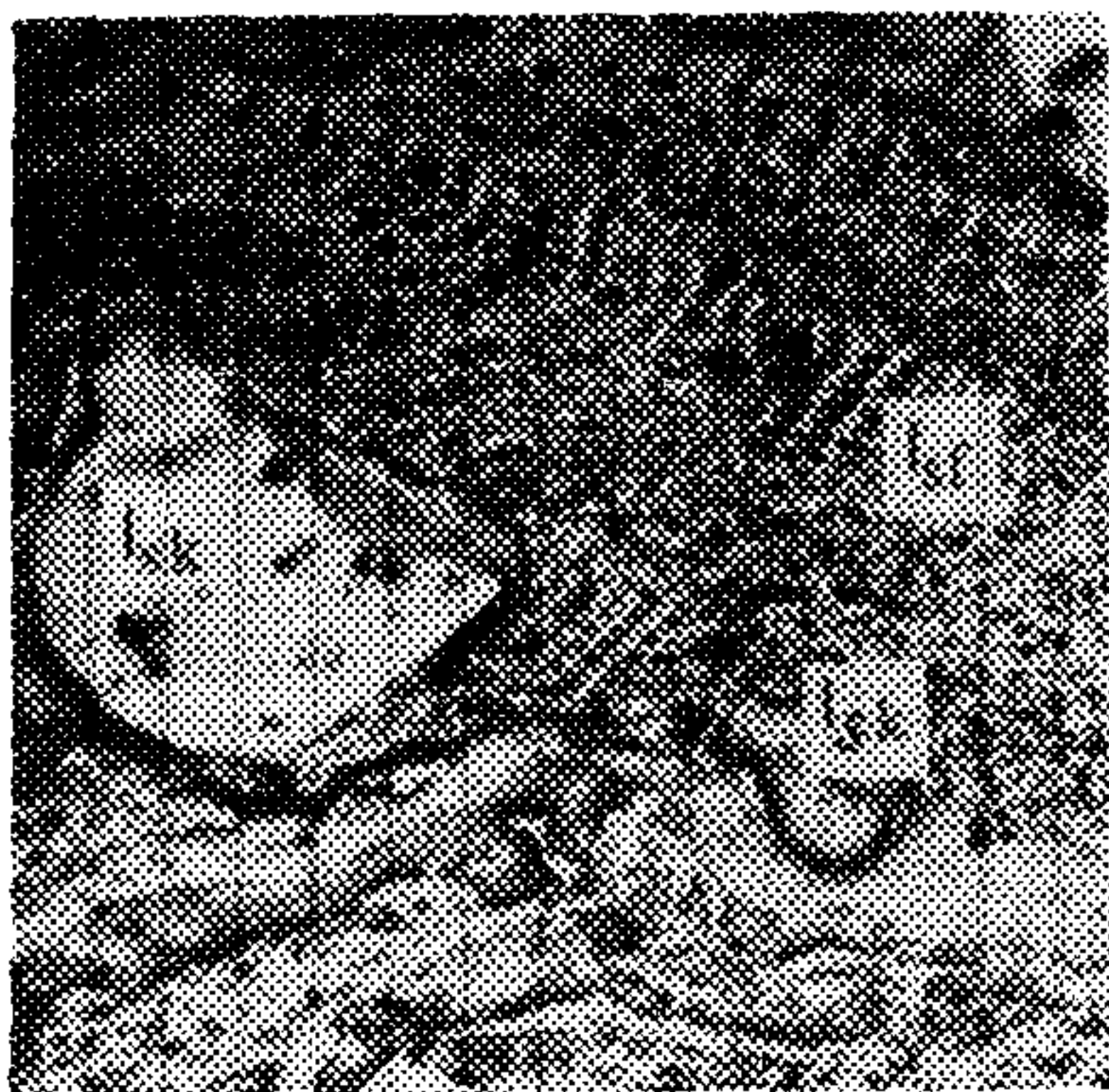
Отраженный свет 100 × I sf — семифюзинит I sk — склеротинит Черт. 7
