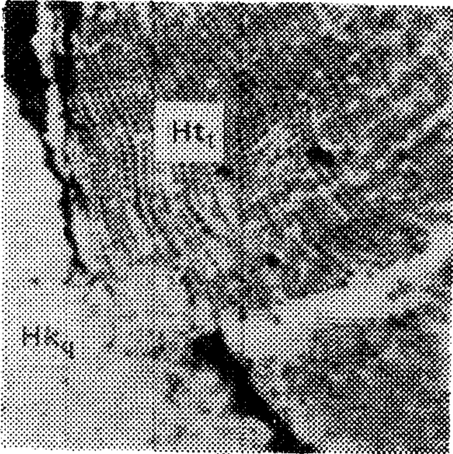
Отраженный свет 100 \times
