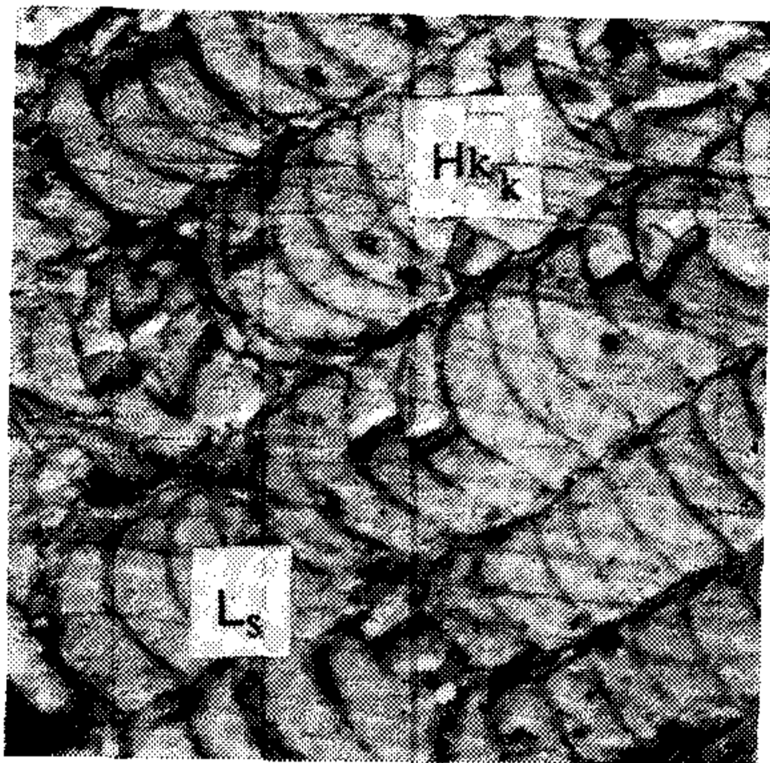
Отраженный свет Масляная иммерсия 400 \times
