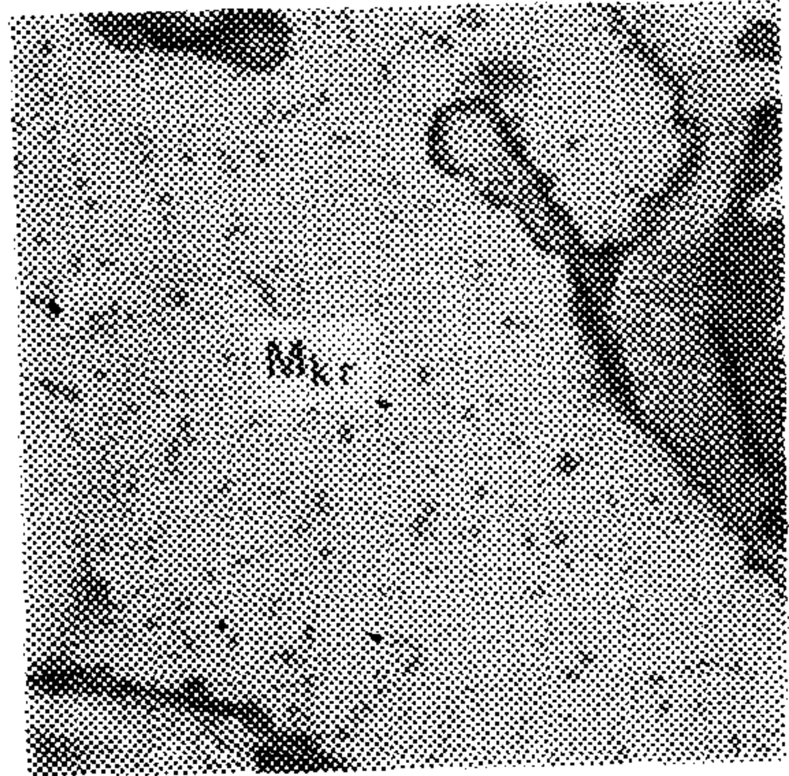
Отраженный свет без иммерсии 200×
