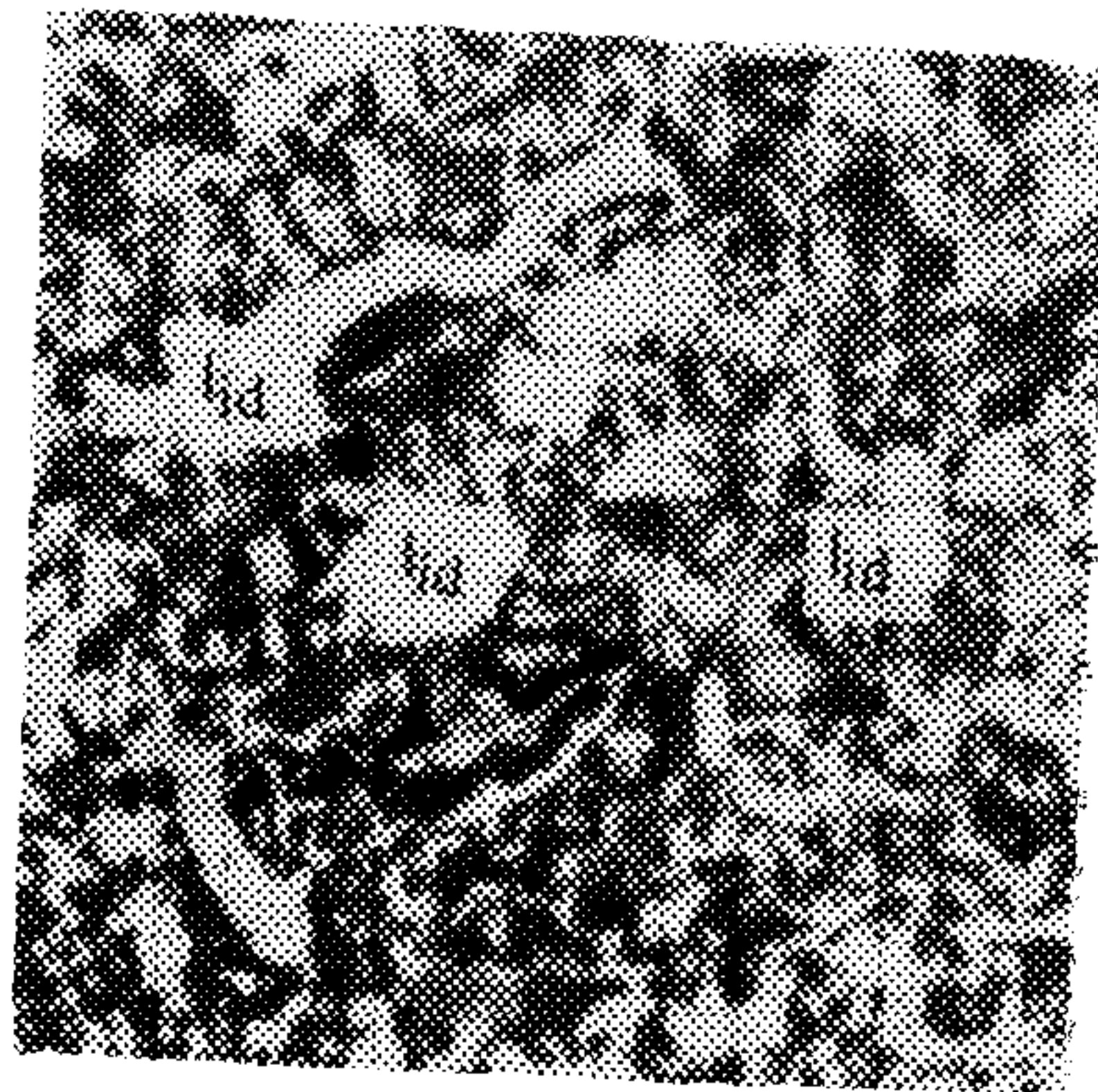
Отраженный свет Масляная иммерсия 500 × I id — инертодетринит Черт. 6
