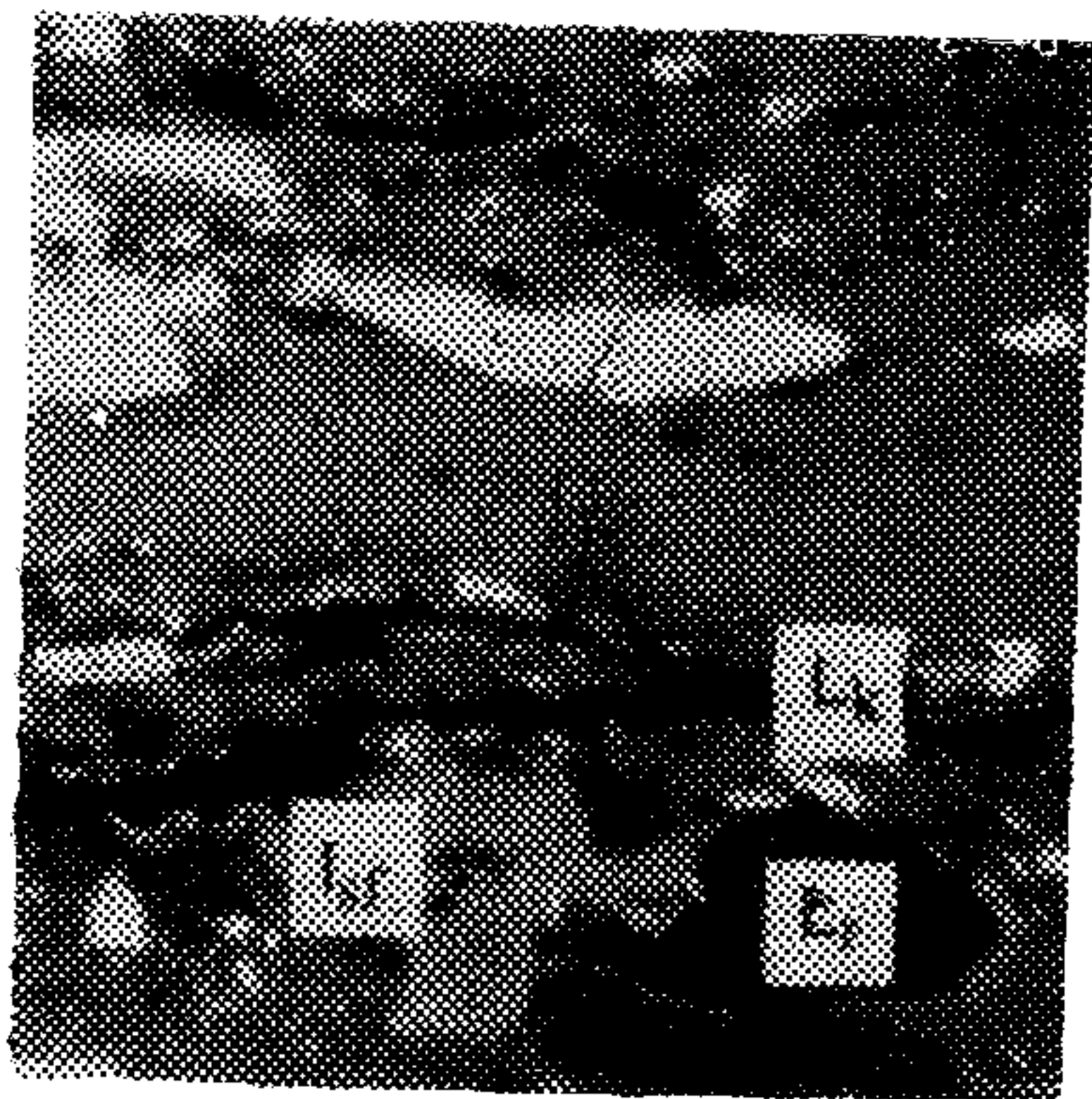
Отраженный свет Масляная иммерсия 600× L_{sf} —семифюзинит L_k —кутинит L_r —резинит Черт. 13
