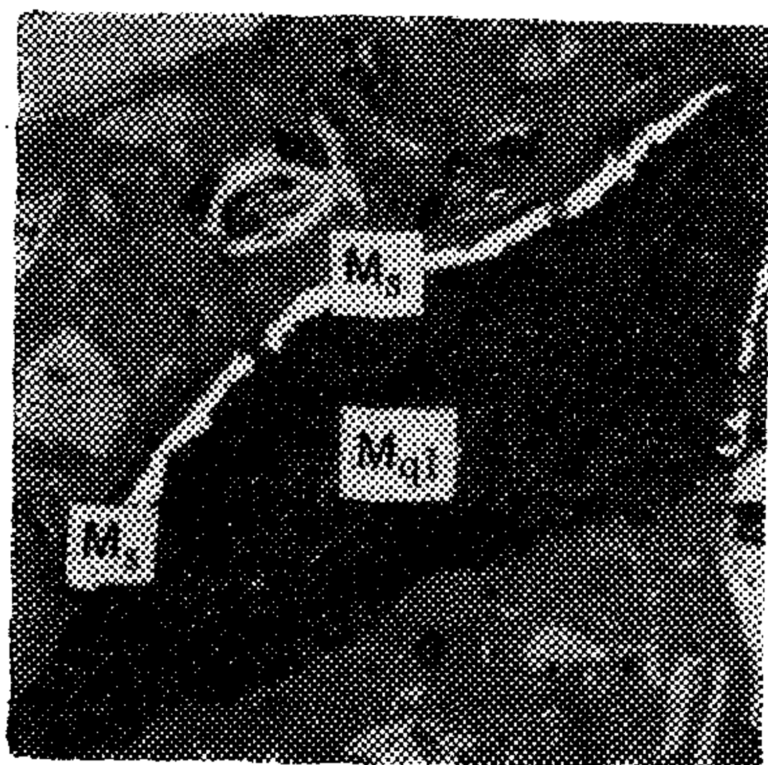
Отраженный свет без иммерсии 200× M_{gl} —глинистые минералы M_s —сульфиды железа Черт. 15
