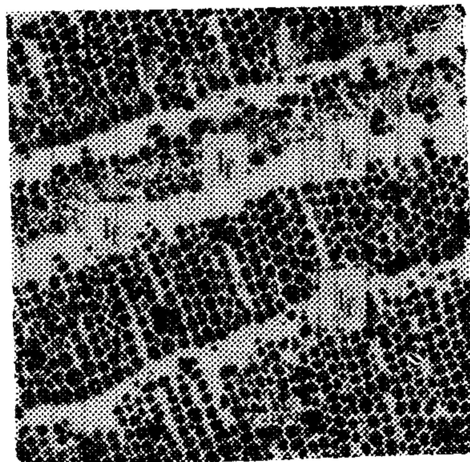
Отраженный свет 100 × I f — фюзинит Черт. 8
