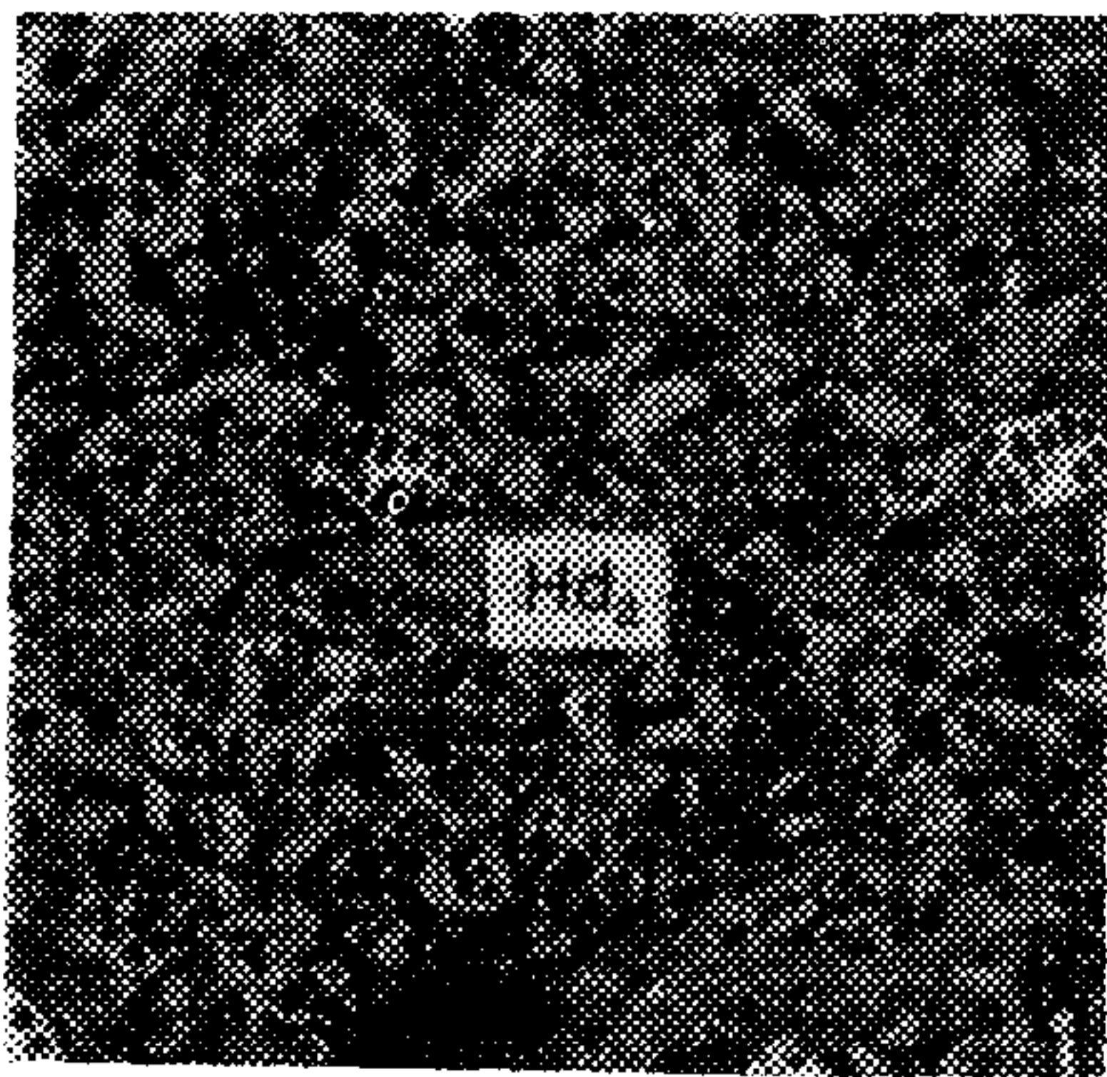
Отраженный свет Масляная иммерсия 400 × Nd a — аттринит Черт. 5
