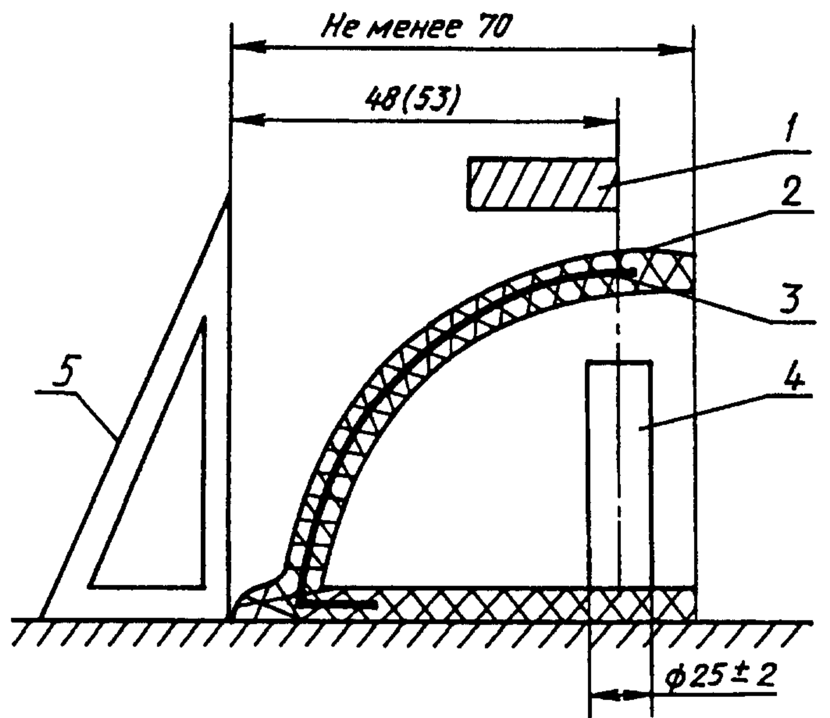
1 — боек; 2 — носок; 3 — ударозащитный подносок; 4 — пластилиновый столбик; 5 — угольник
