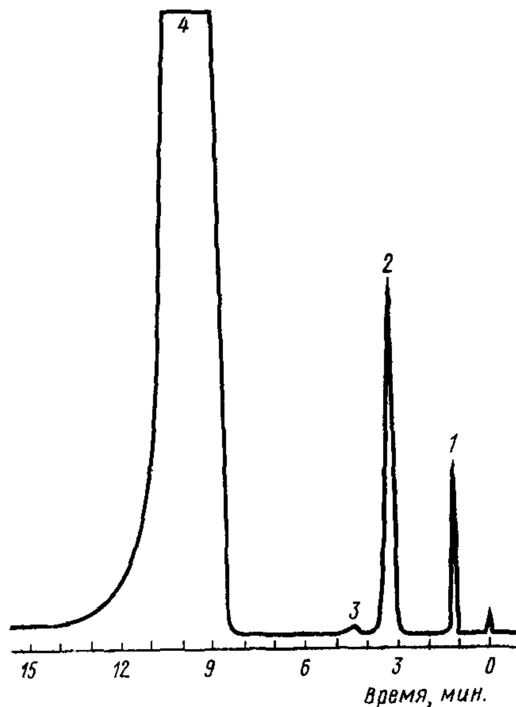
Типовая хроматограмма продукта
