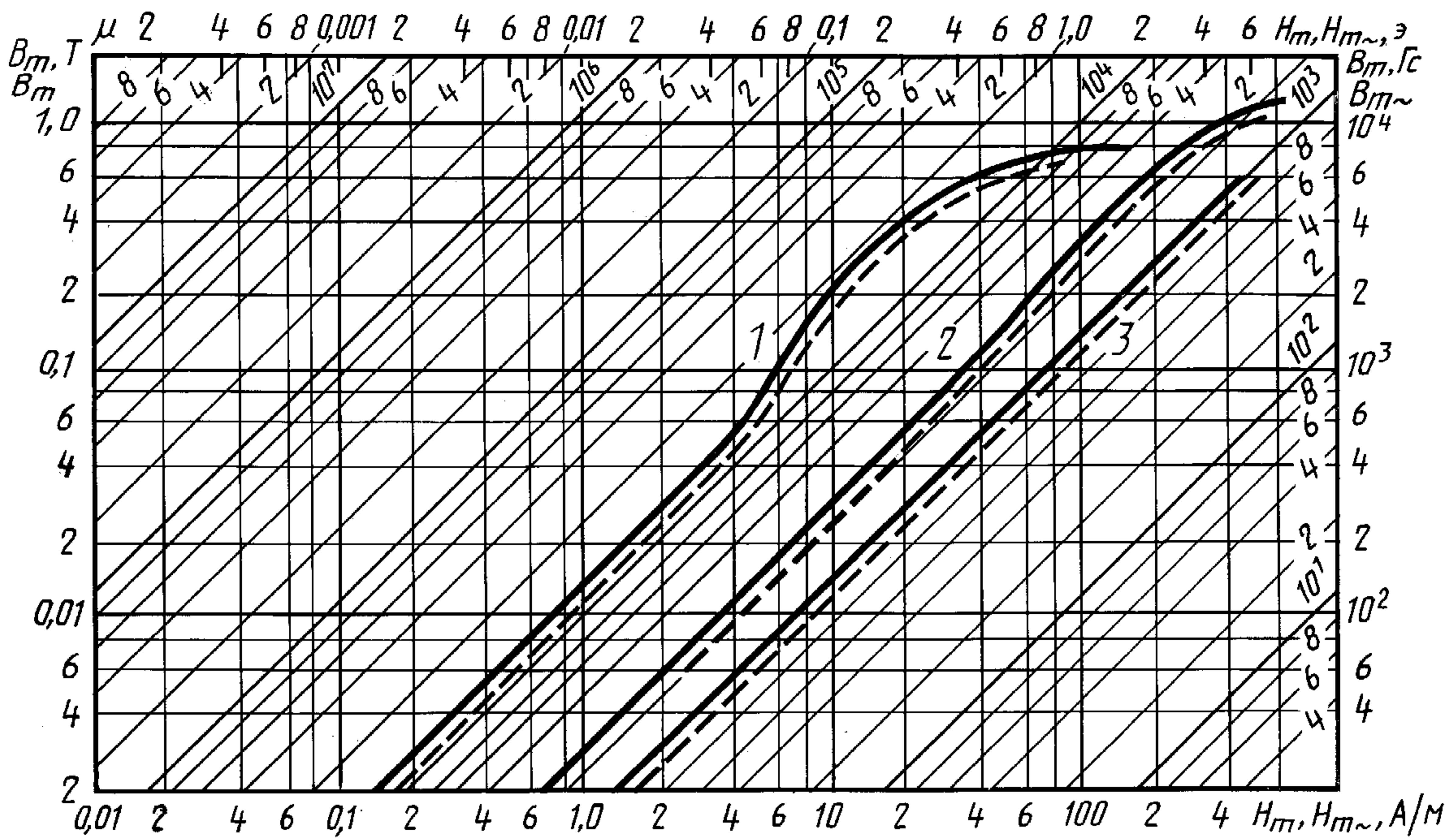
Кривые намагничивания образцов ленты толщиной 0,02 мм из сплавов марок 1—79НЗМ, 2—64Н, 3—47НК.
