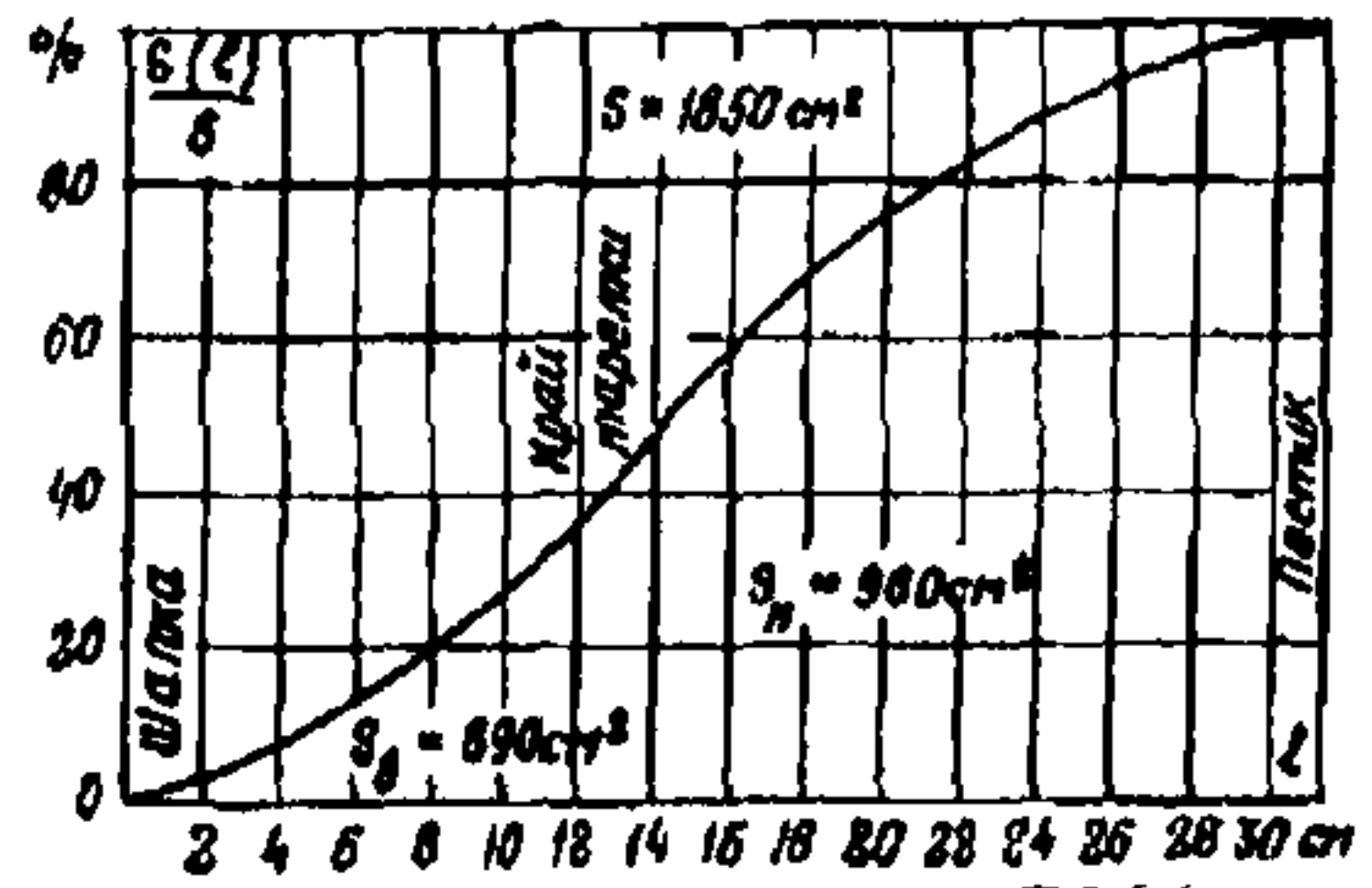
Рис.26. График для определения площади поверхности изолятора ПФ6 (чертеж И-519) и площадей отдельных участков его поверхности
