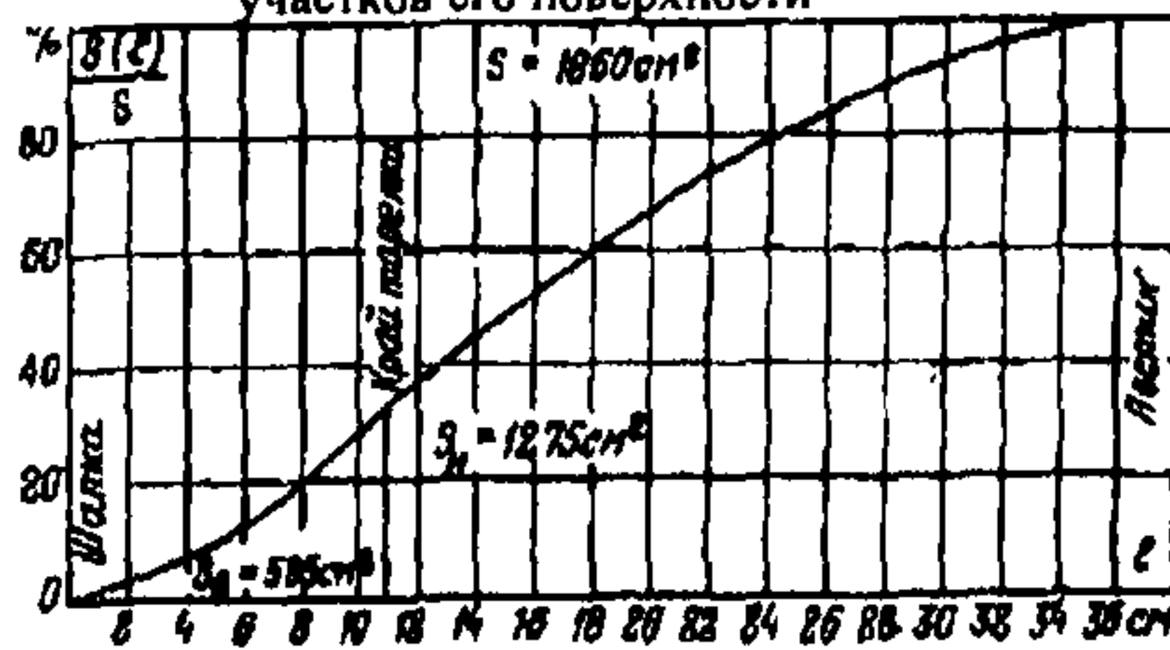
Рис.30. График для определения площади поверхности изолятора ПФ6-И (чертеж И-497) и площадей отдельных участков его поверхности
