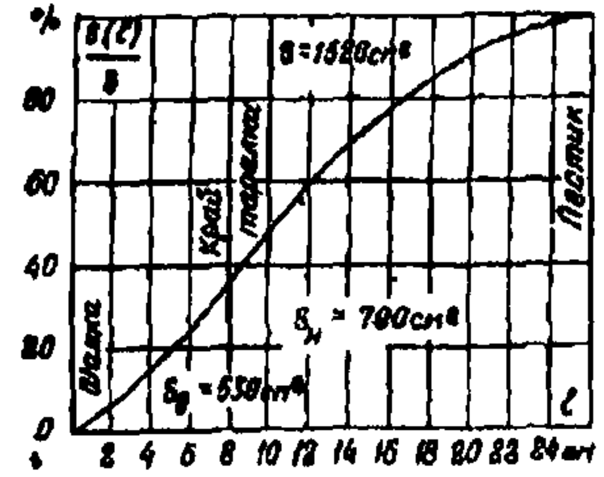
Рис.24. График для определения площади поверхности изолятора ПМ-4,5 (чертеж И-1587А) и площадей отдельных участков его поверхности
