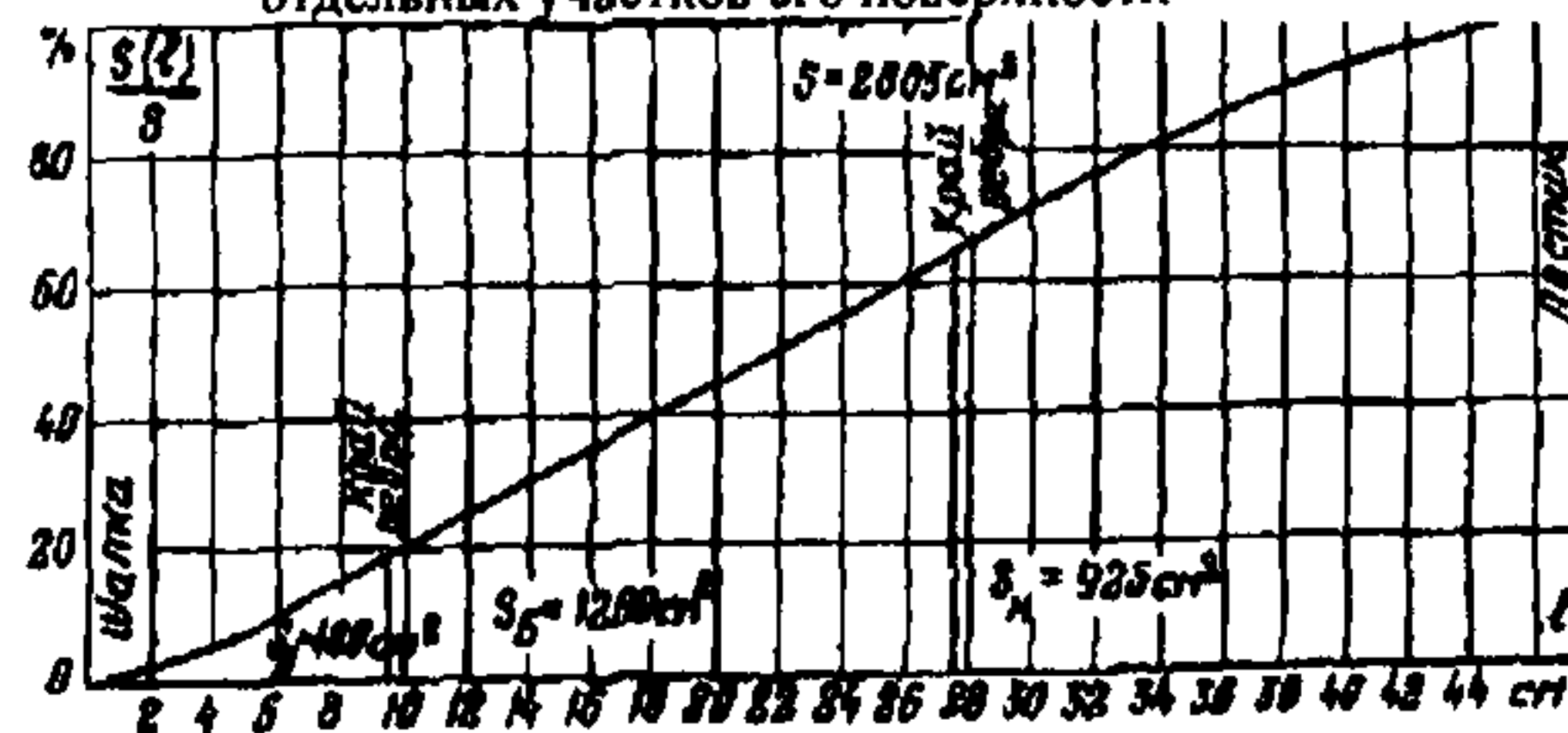
Рис.32. График для определения площади поверхности изолятора ПФ6-Б (чертеж И-3359) и площадей отдельных участков его поверхности
