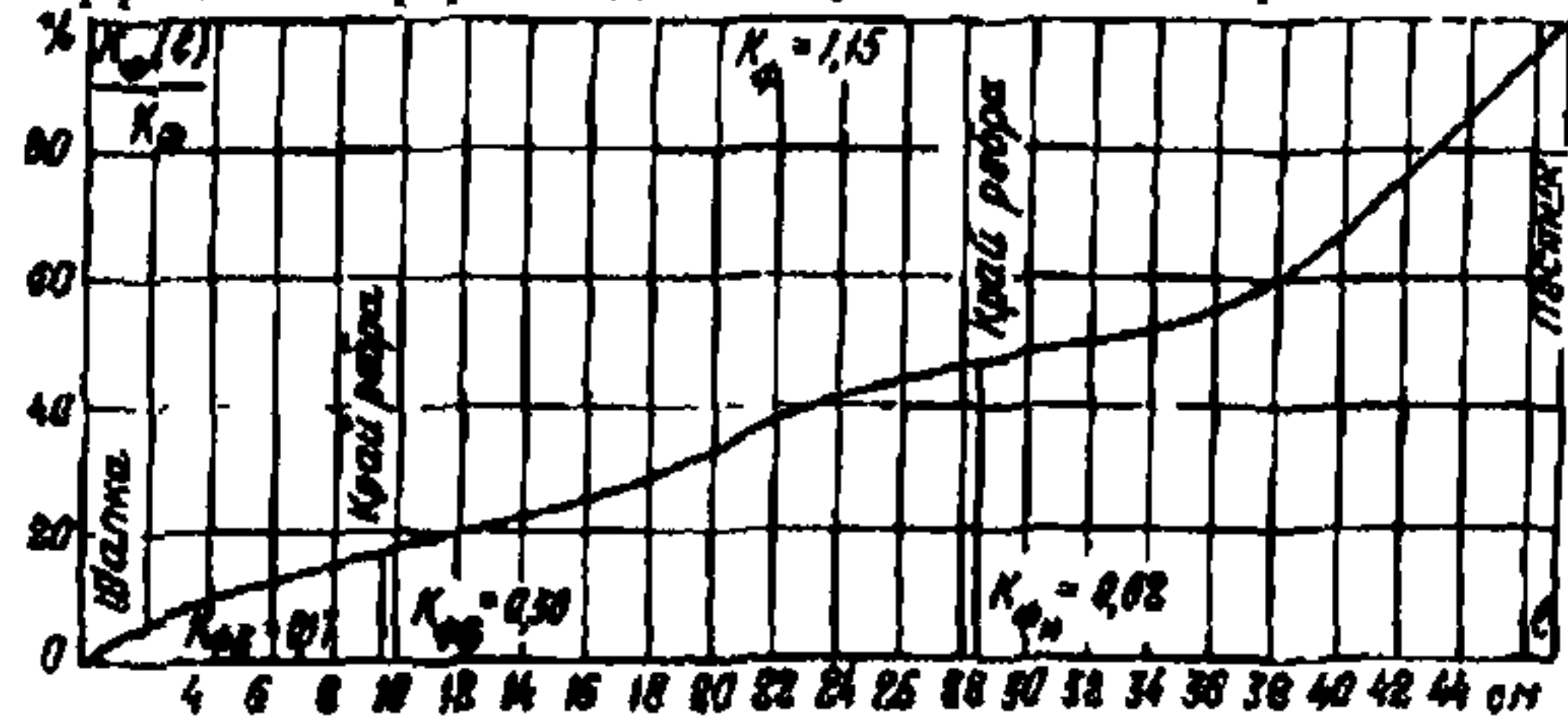
Рис. 17. График для определения коэффициента форм изолятора NS-2 (чертеж И-324) и коэффициентов формы
