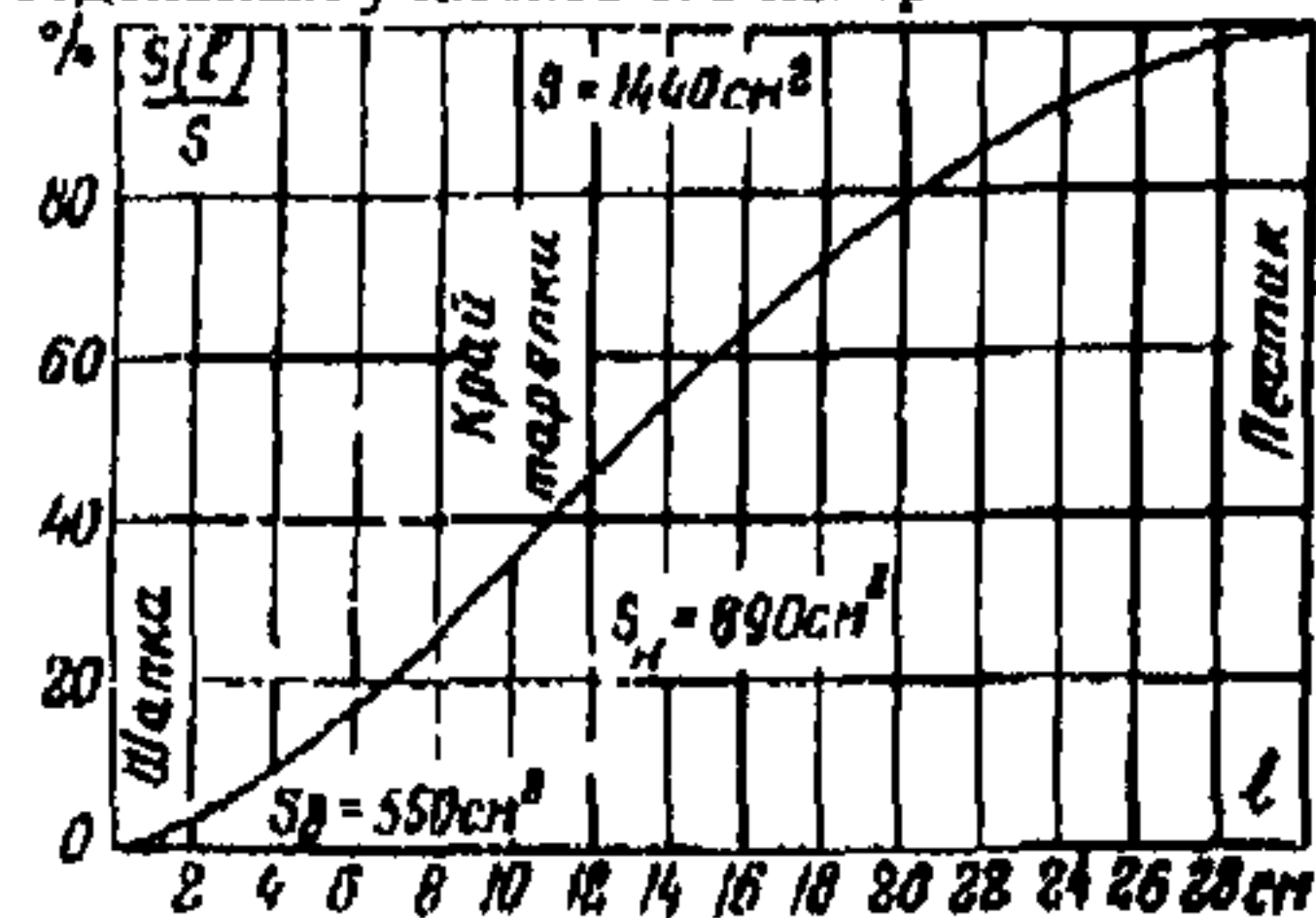
Рис.36. График для определения площади поверхности изолятора ПС6-Б (чертеж И-459) и площадей отдельных участков его поверхности
