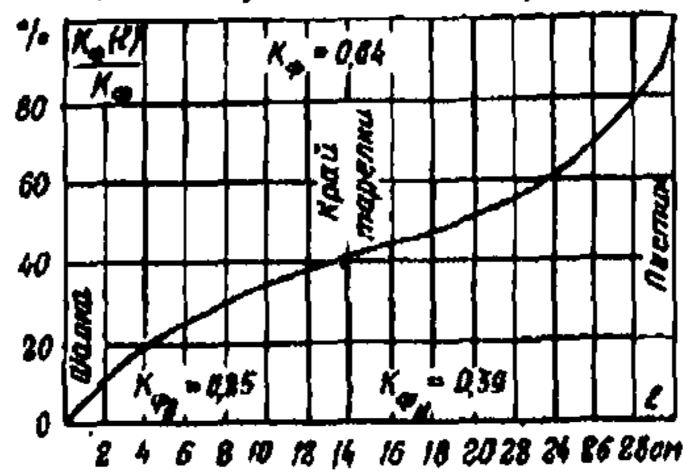
Рис.20. График для определения коэффициент формы изолятора ПС6-1 (чертеж И-428) и коэффициентов формы отдельных участков его поверхности
