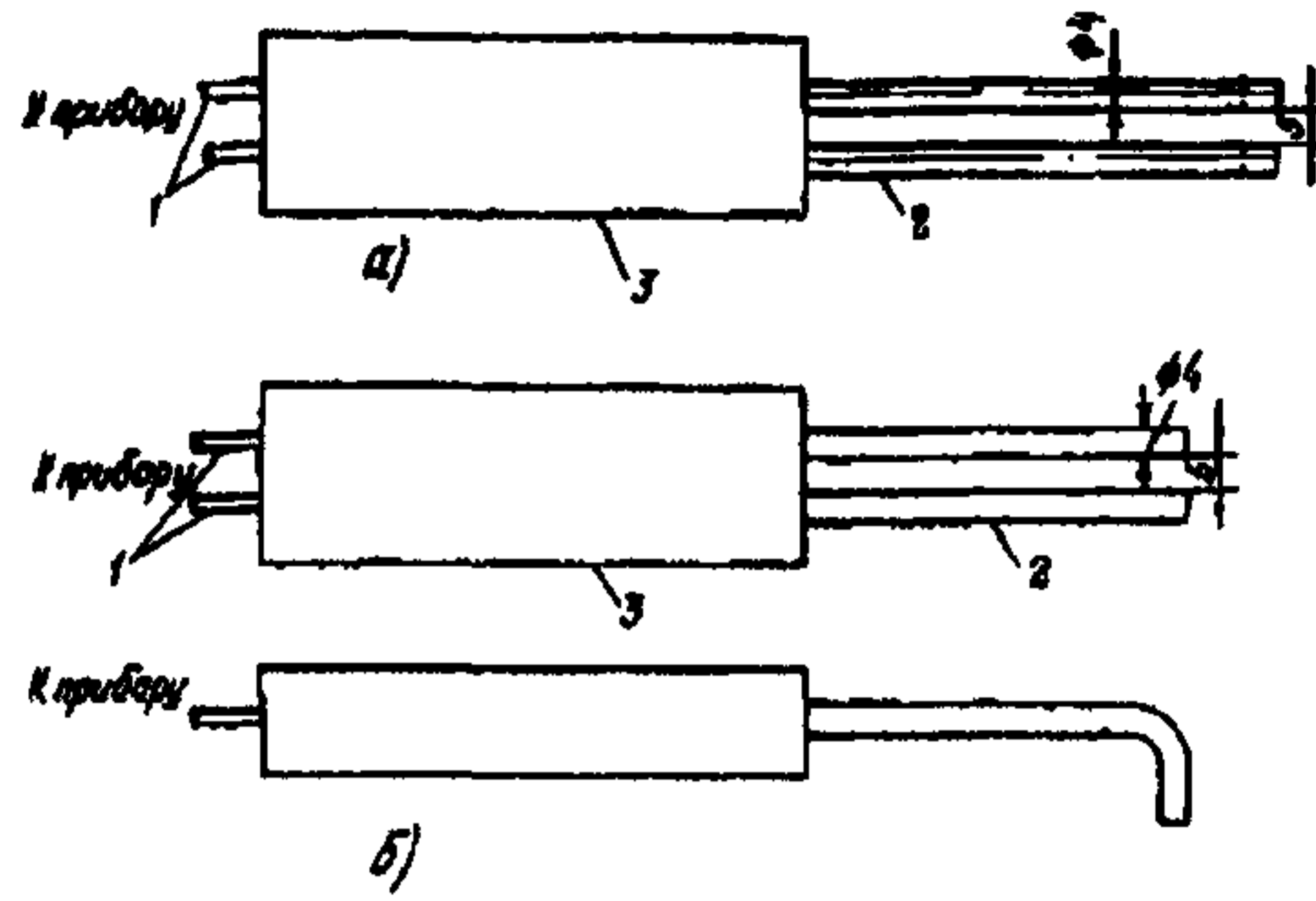
Рис. 1. Эскиз зонда: а - прямые электроды; б - загнутые электроды; 1 - зажимы; 2 - электроды; 3 – изолирующий корпус
