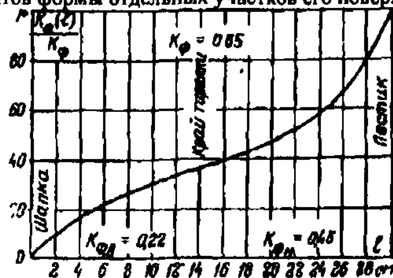
Рис.12. График для определения коэффициента формы изолятора ПФ6-1 (чертеж И-414) и коэффициентов
