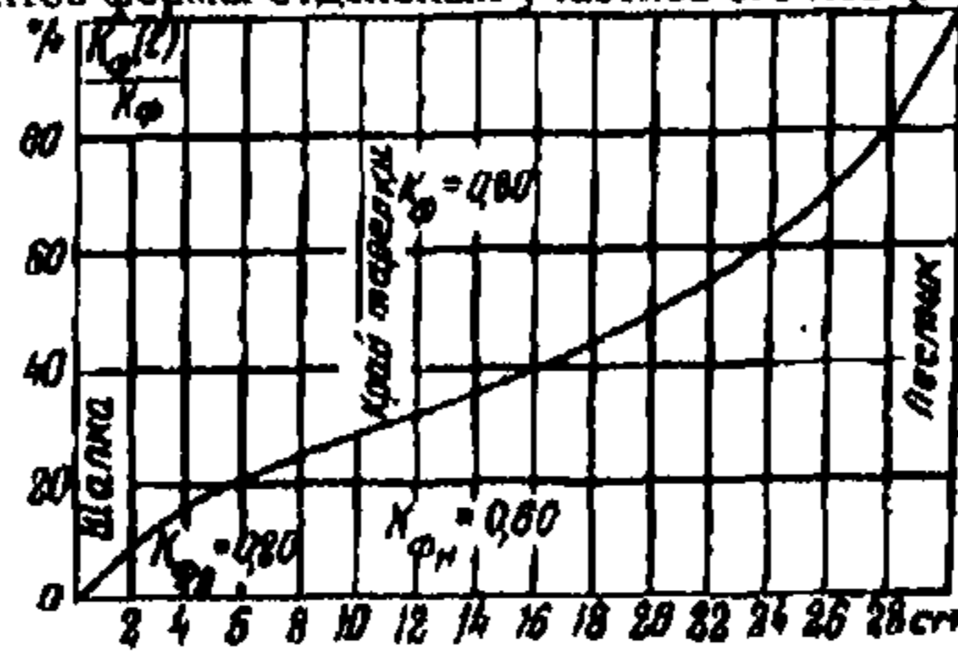
Рис.19. График для определения коэффициента формы изолятора ПС6-Б (чертеж И-459) и коэффициентов формы отдельных участков его поверхности
