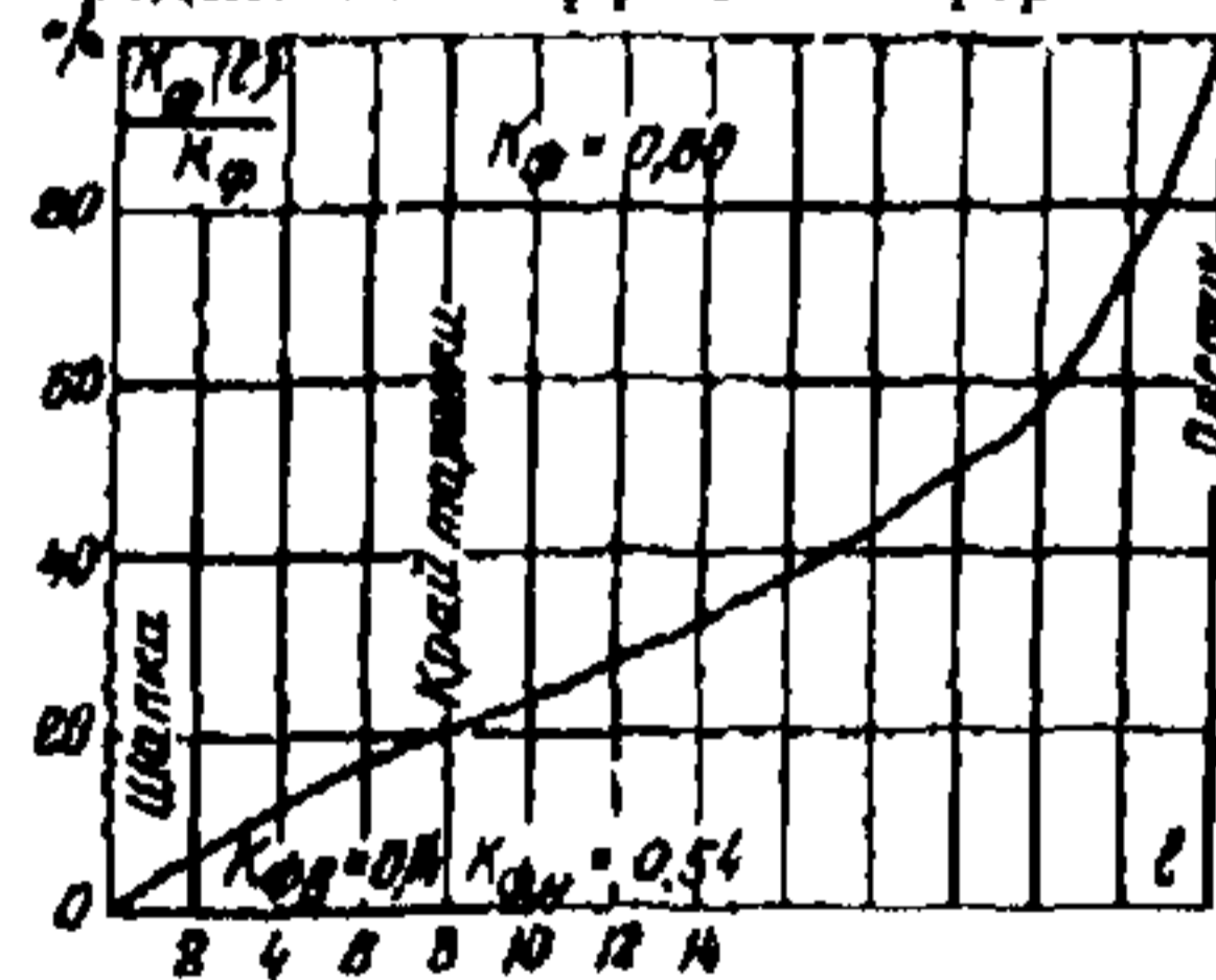
Рис.7. График для определения коэффициента, формы изолятора ПМ-4,5 (чертеж И-1587 СКТЬ 1 треста Электросетьизоляция) и коэффициентов формы отдельных участков его поверхности. Индекс В относится к верху изолятора, индекс н - к низу изолятора
