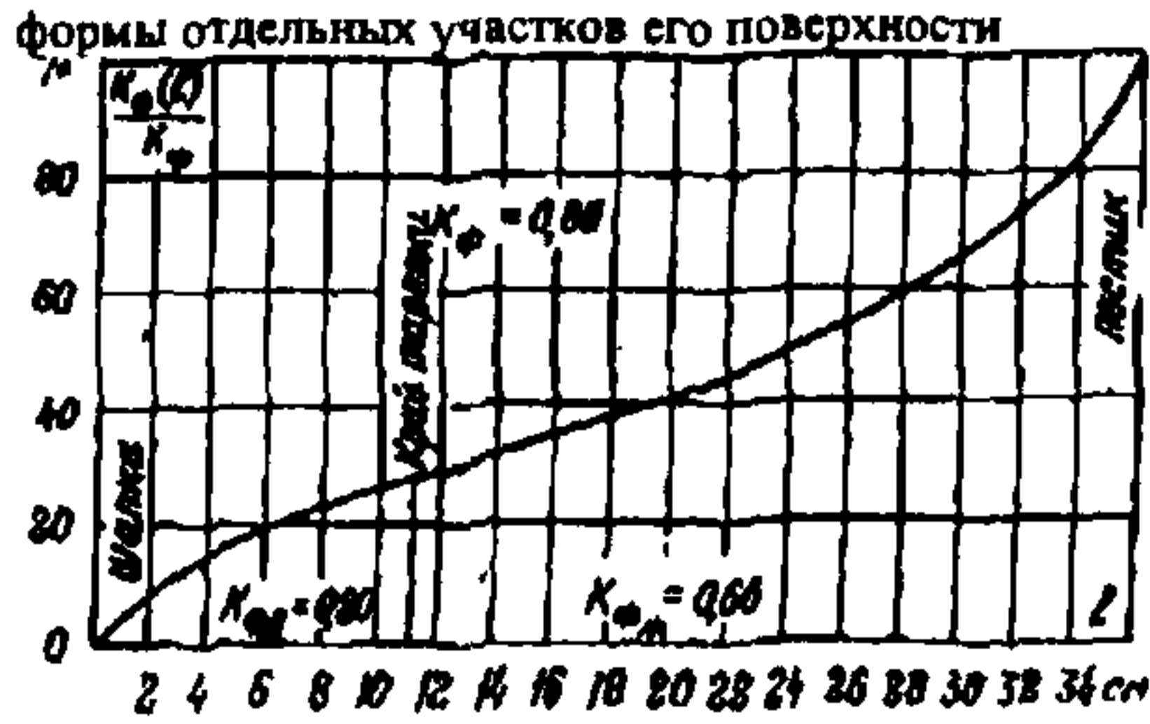
Рис. 13. График для определения коэффициента формы изолятора ПФГ6-1 (чертеж И-497) и коэффициентов формы отдельных участков его поверхности
