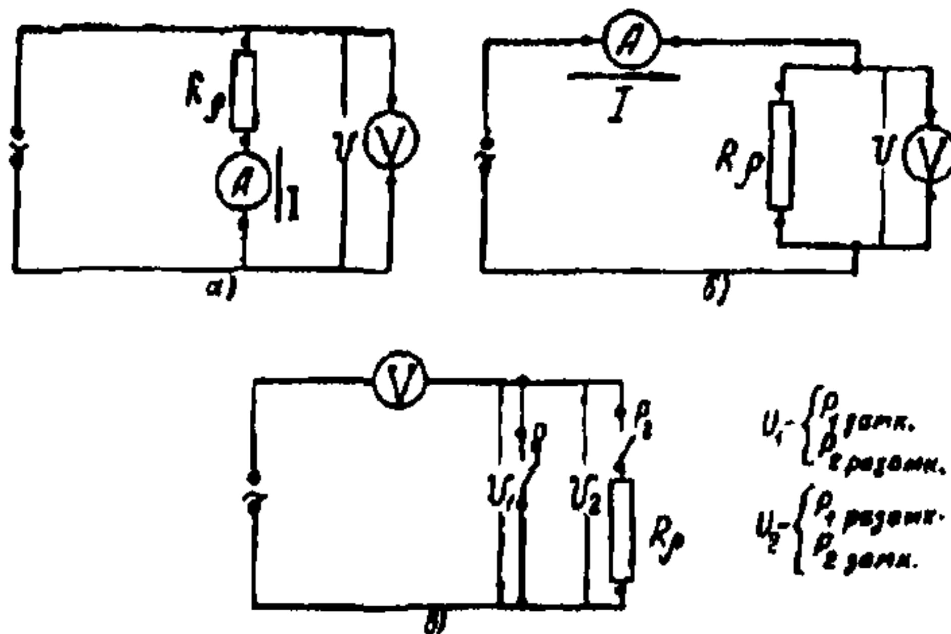
Рис.42. Возможные схемы измерения удельной объемной проводимости:
