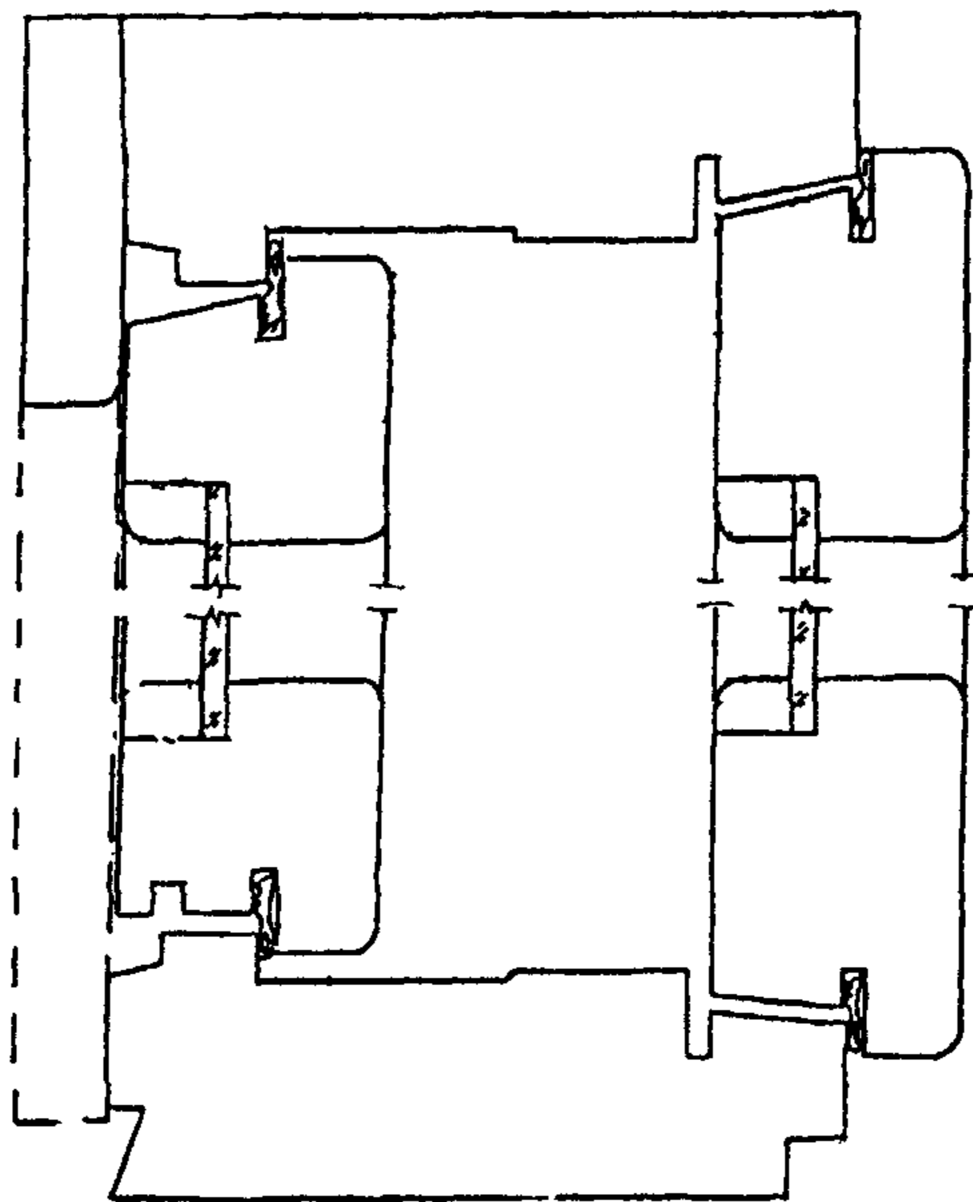
Рисунок 7 – Пример раздельной конструкции оконного блока с двойным остеклением (бруски коробки имеют универсальный профиль, что позволяет устанавливать дополнительную створку и преобразовывать конструкцию в раздельно-спаренную)
