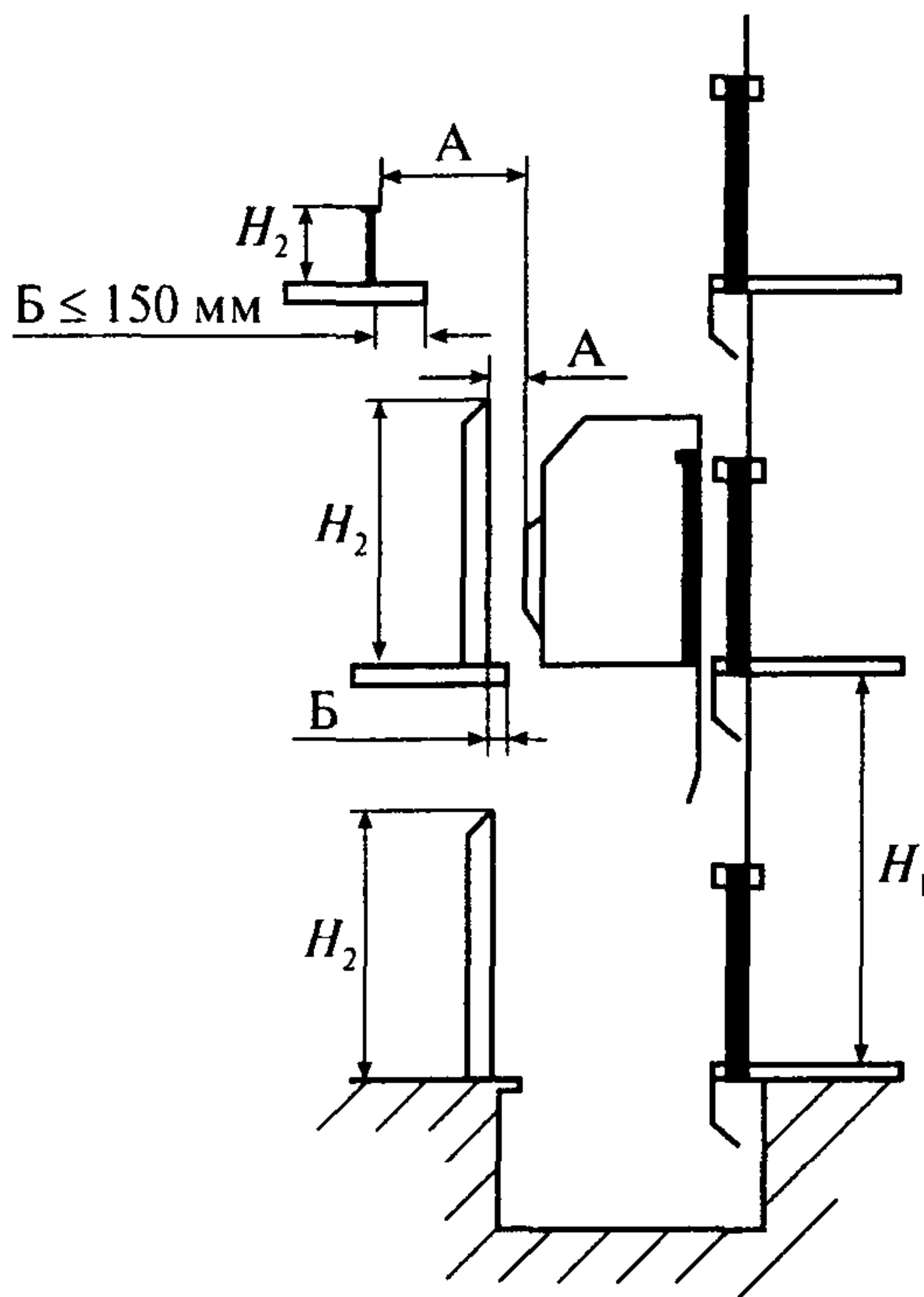
Рис. 1. Расстояние до движущихся элементов лифта:
