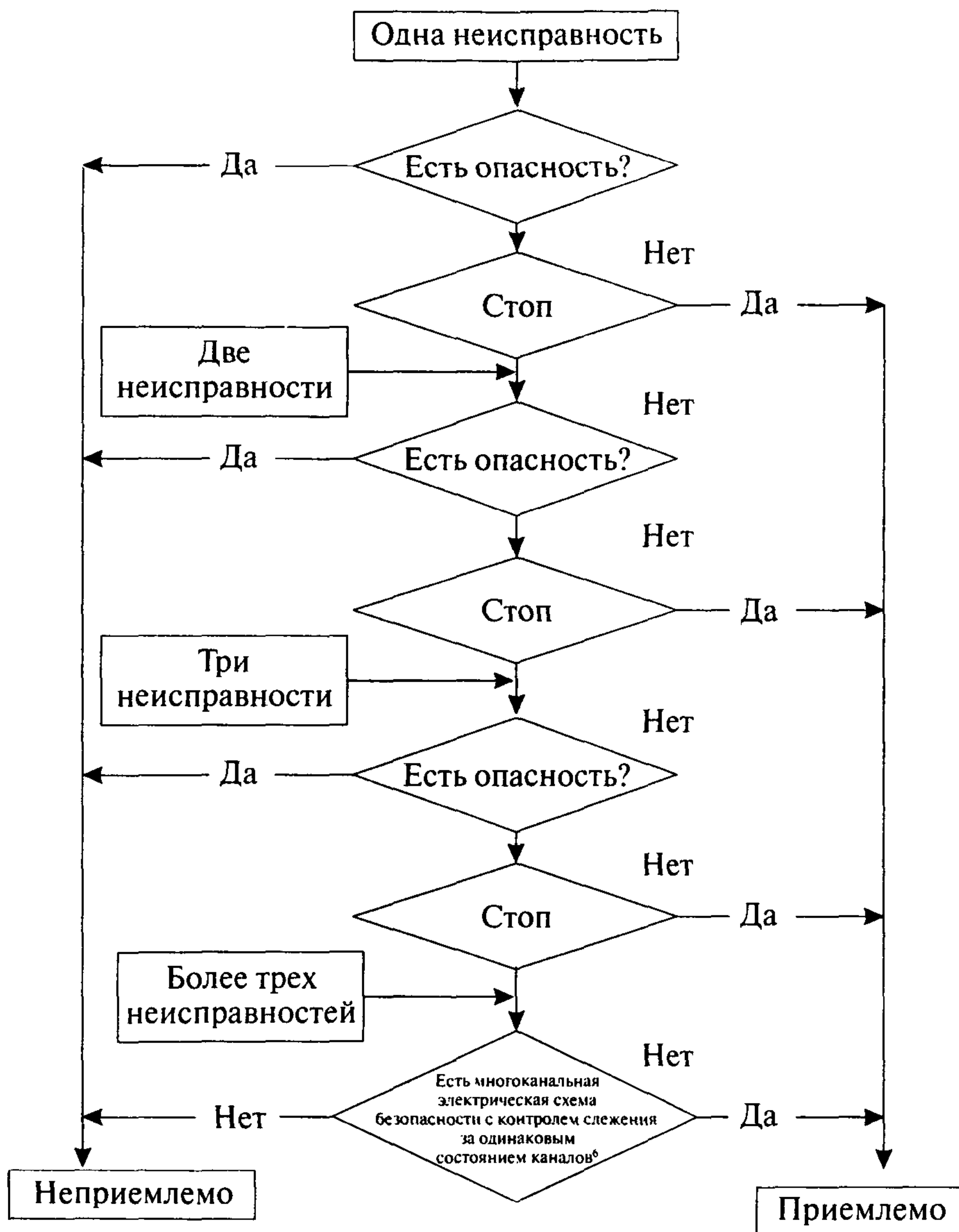
Рис. 6. Блок-схема оценки электрических схем безопасности
