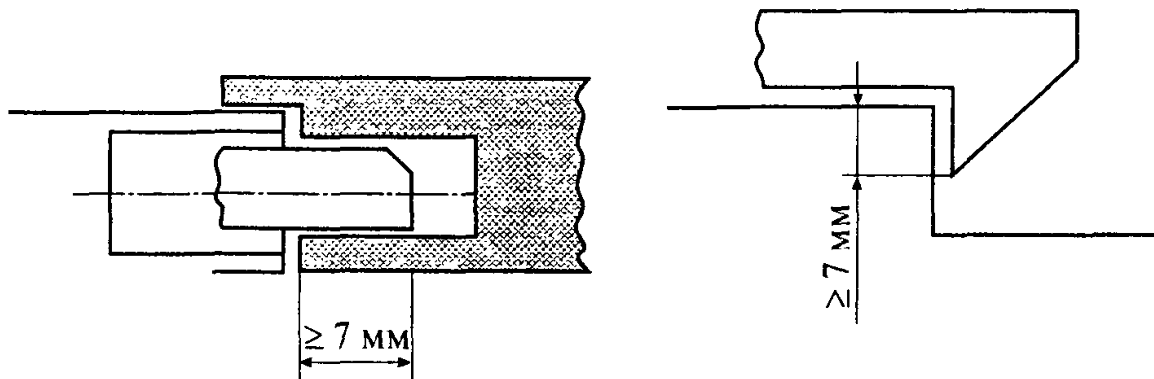
Рис. 5. Запирающее устройство автоматического замка двери шахты
