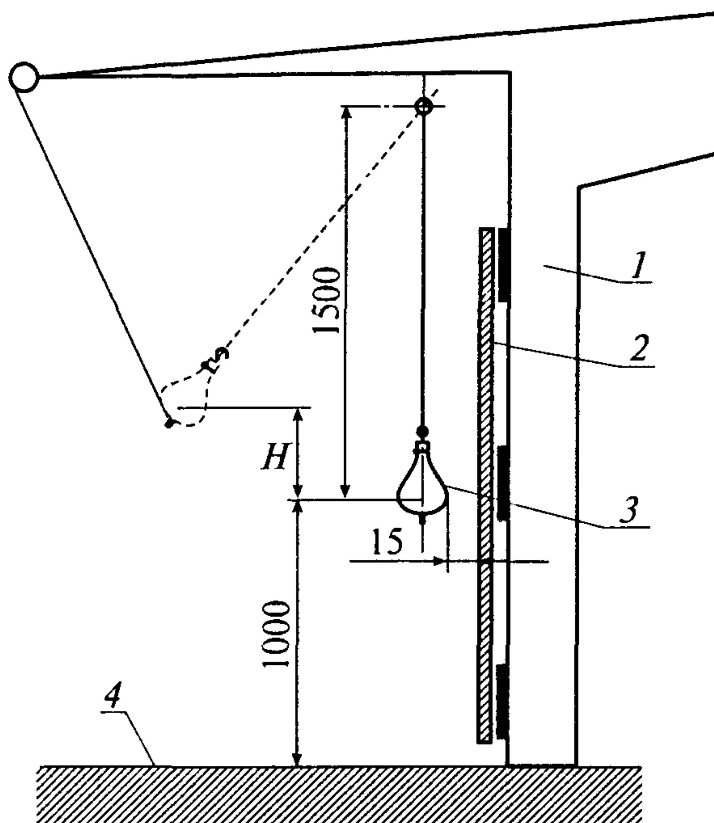
Рис. 3. Высота падения на испытательном стенде:
