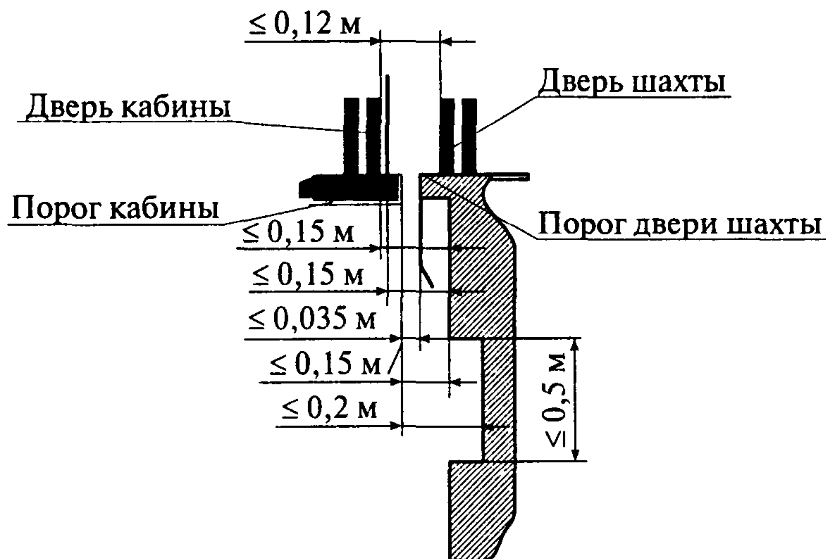
Рис. 3. Расстояния между элементами кабины и шахты
