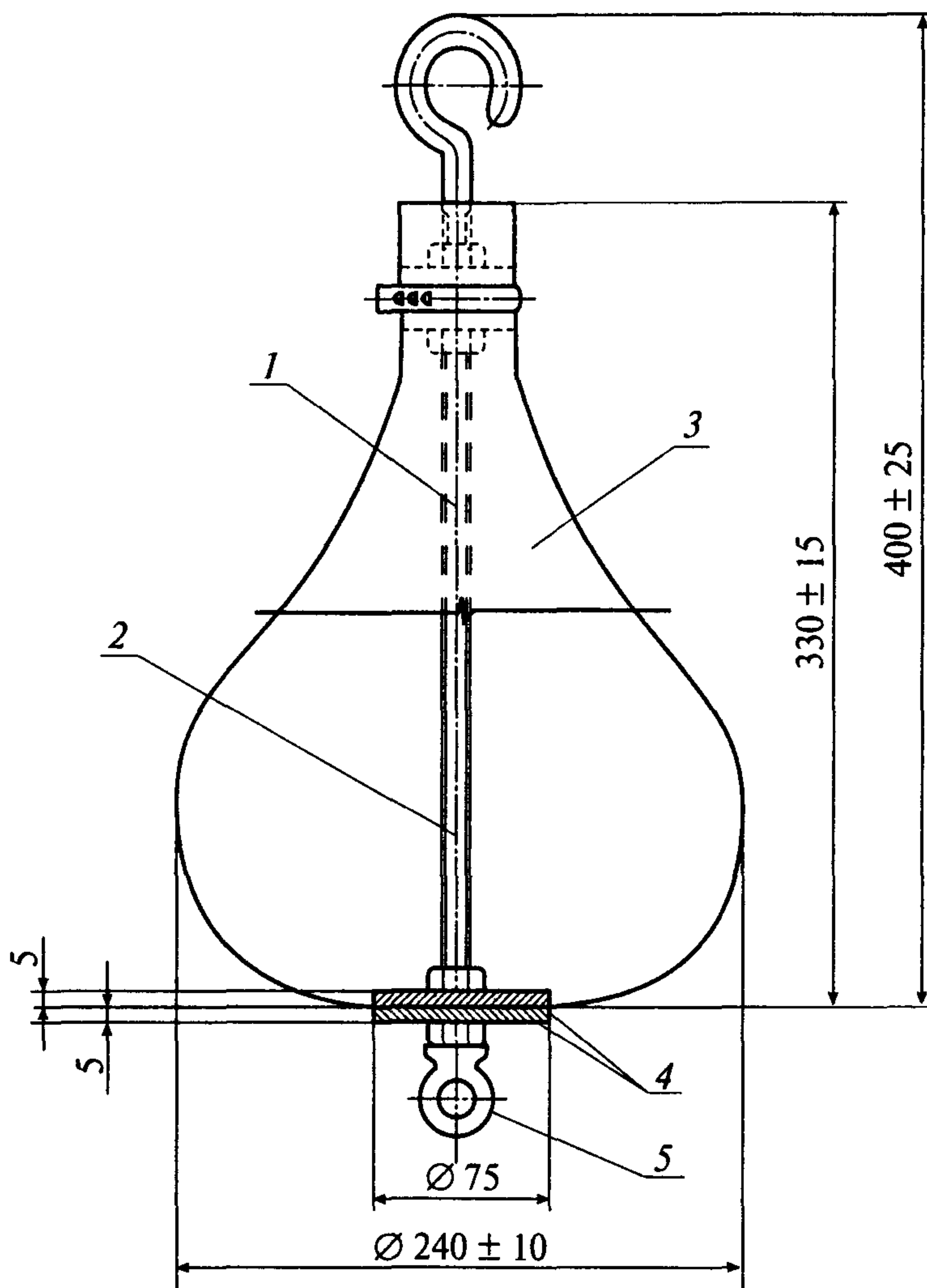
Рис. 2. Маятник для нежесткого удара:
