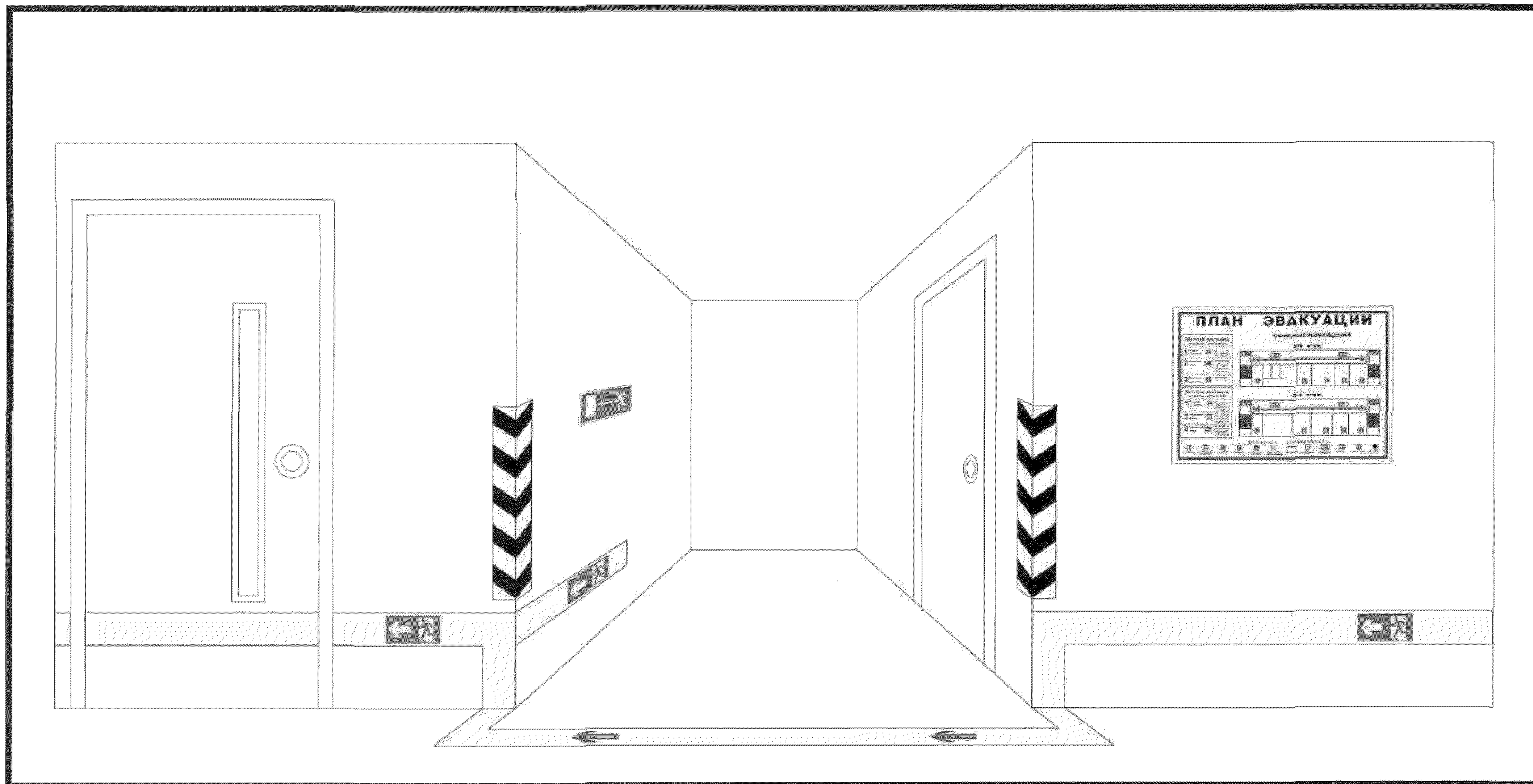
Рисунок Б.4 — Пример обозначения элементами ФЭС коридора при наличии тупика. Направляющая полоса переходит со стены на пол, исключая возможный разрыв в обозначении пути эвакуации, а затем снова переходит на стену
