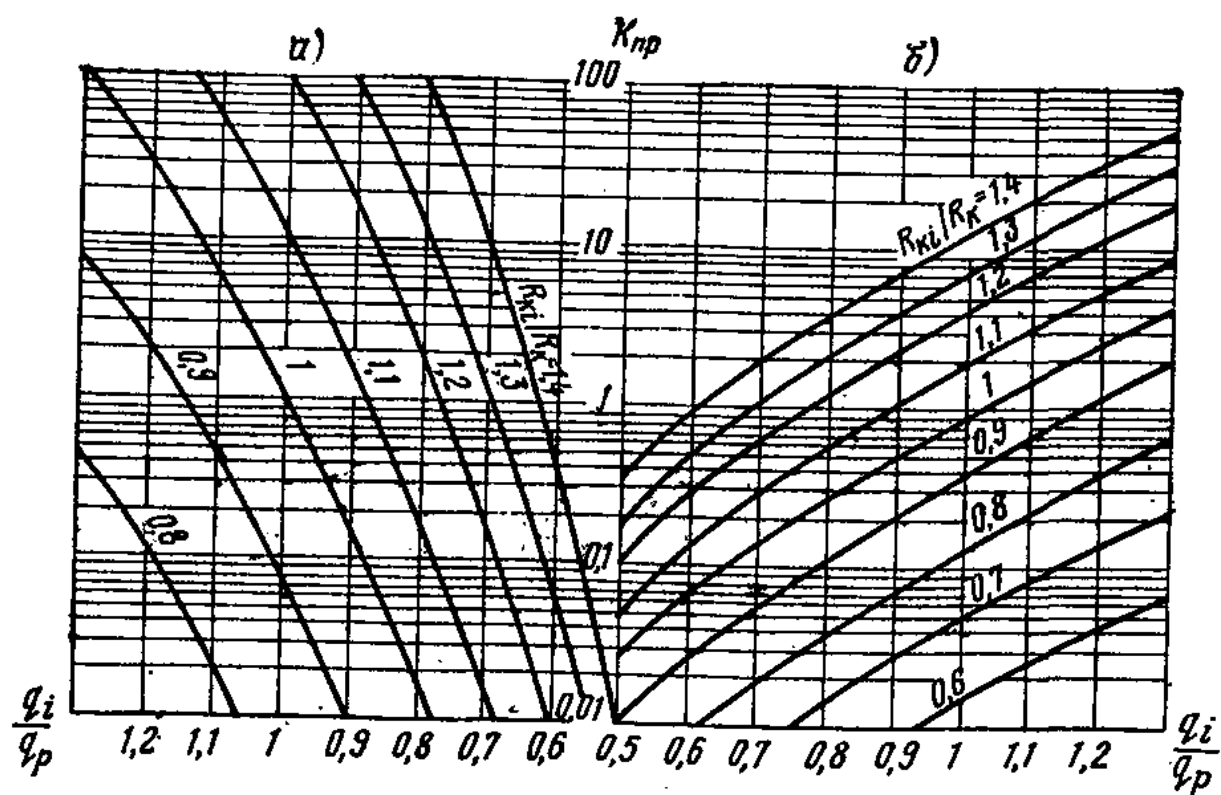
Рис. 22. Номограммы для определения коэффициентов приведения нагрузки к расчетной k_{пр} для нежестких покрытий
