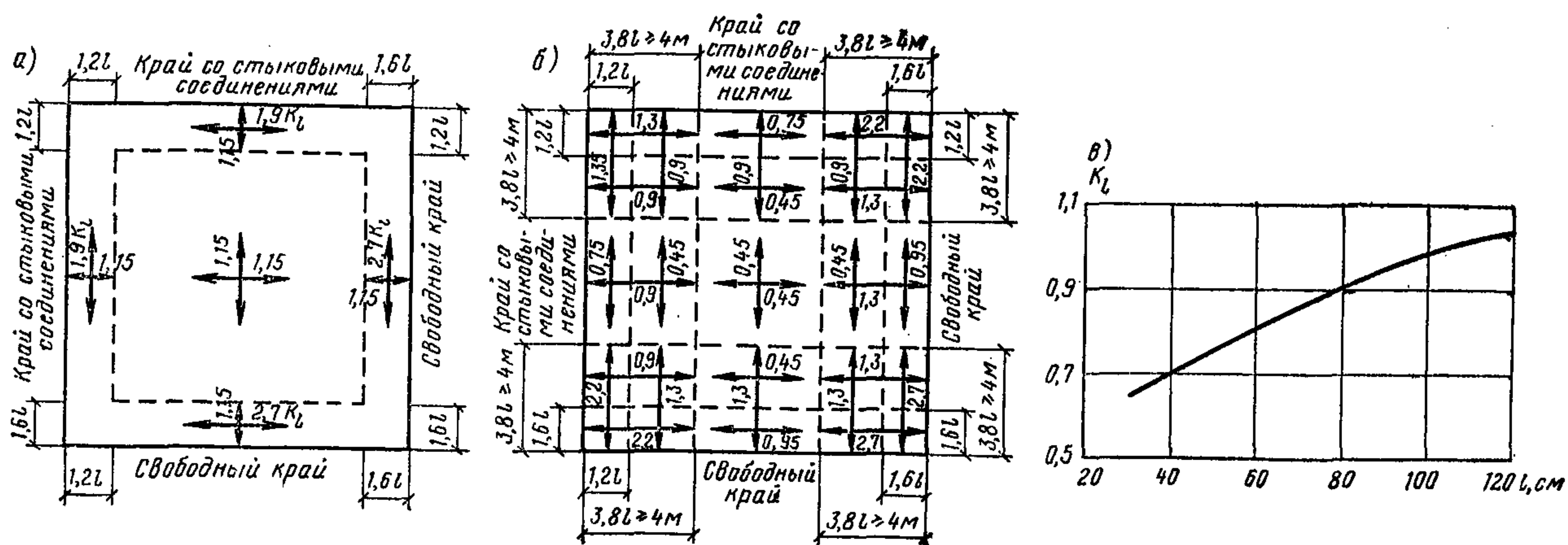
Рис. 14. Значения переходных коэффициентов K
