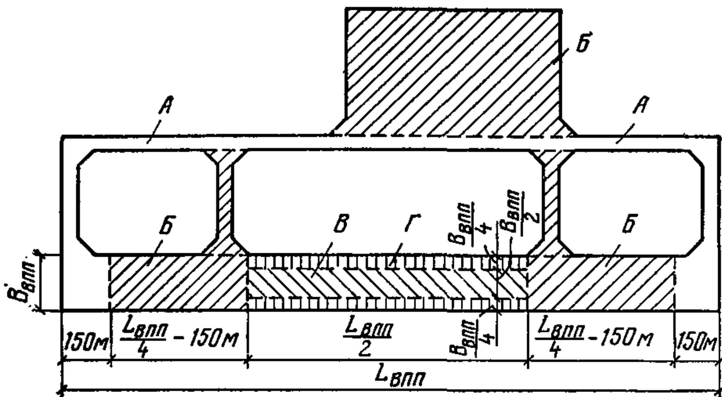
Рис. 2. Схема деления покрытий аэродрома на группы участков
