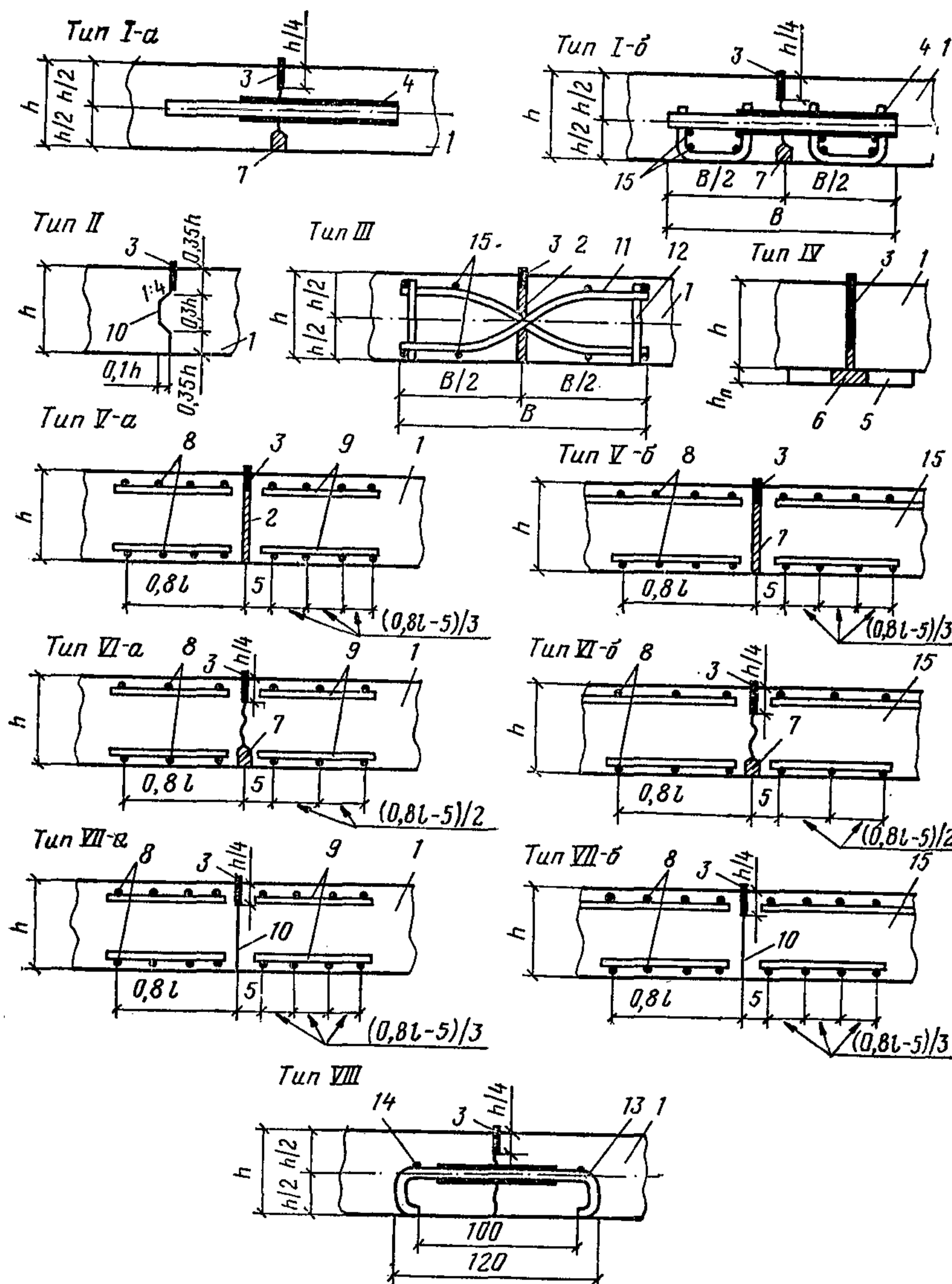
Рис. 3. Схемы конструкций деформационных швов (размеры в см)
