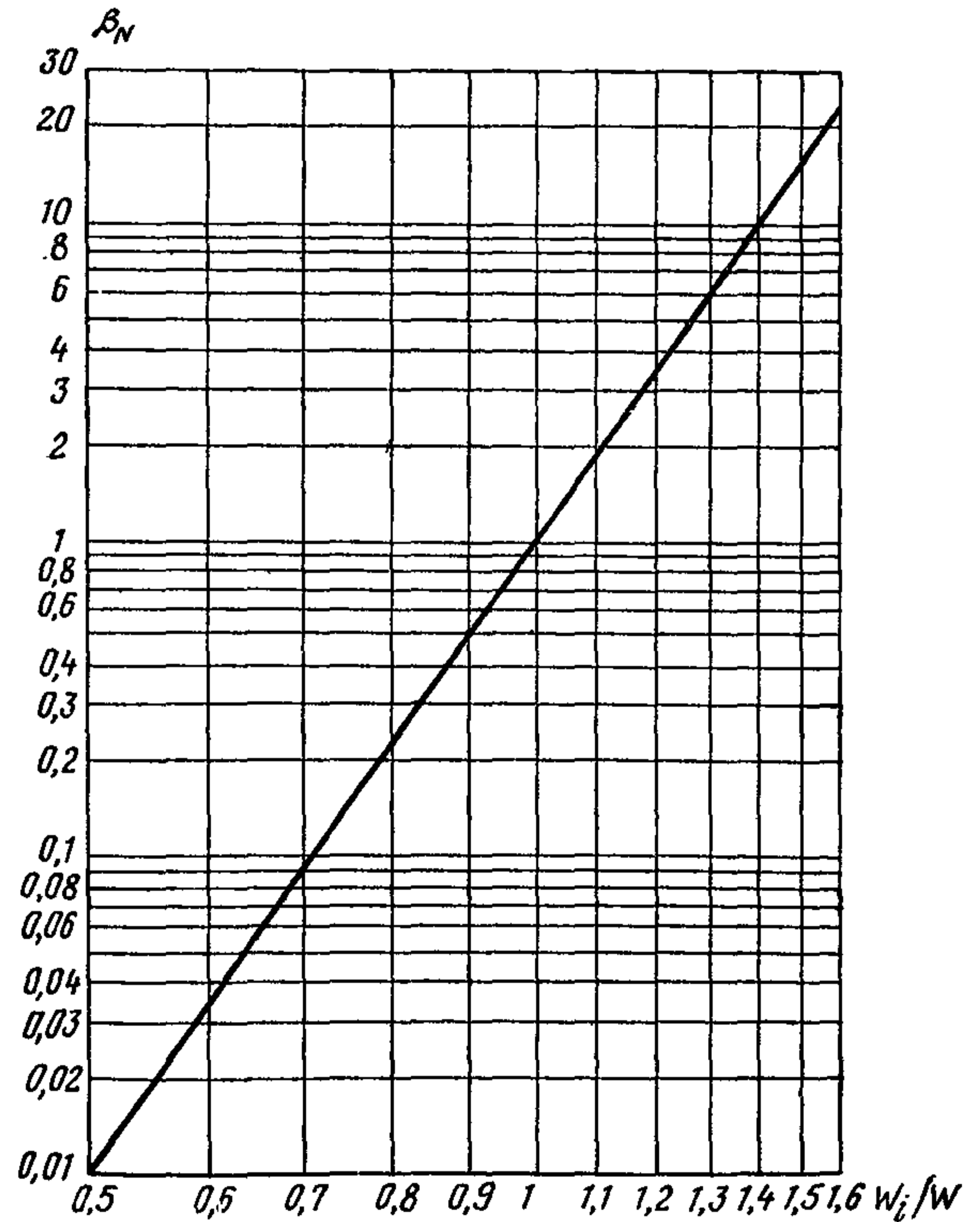
Рис. 19. График для определения коэффициента \beta_N
