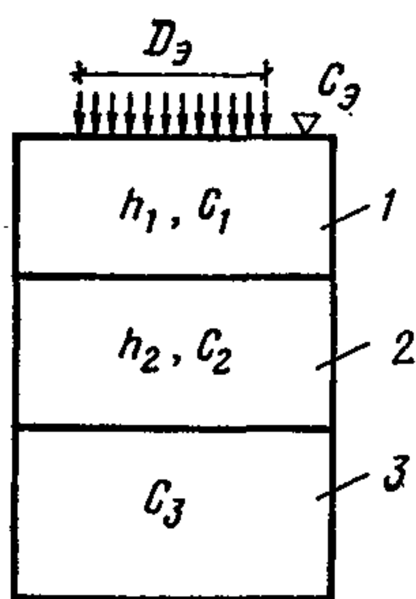
Рис. 6. Расчетная схема слоистого основания для определения эквивалентного коэффициента постели
