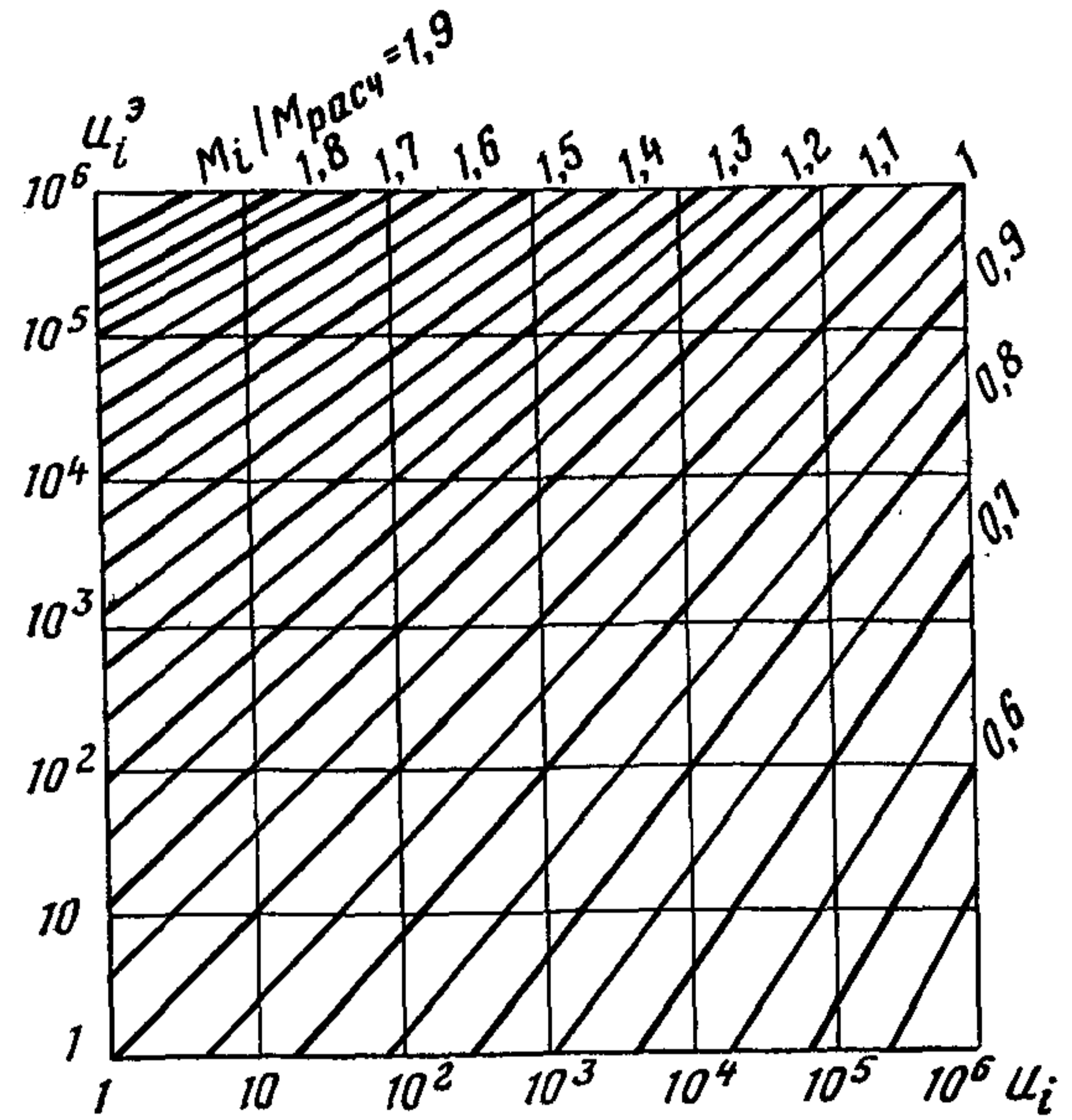
Рис. 18. Номограмма для определения эквивалентного числа приложений нагрузки u_i^э
