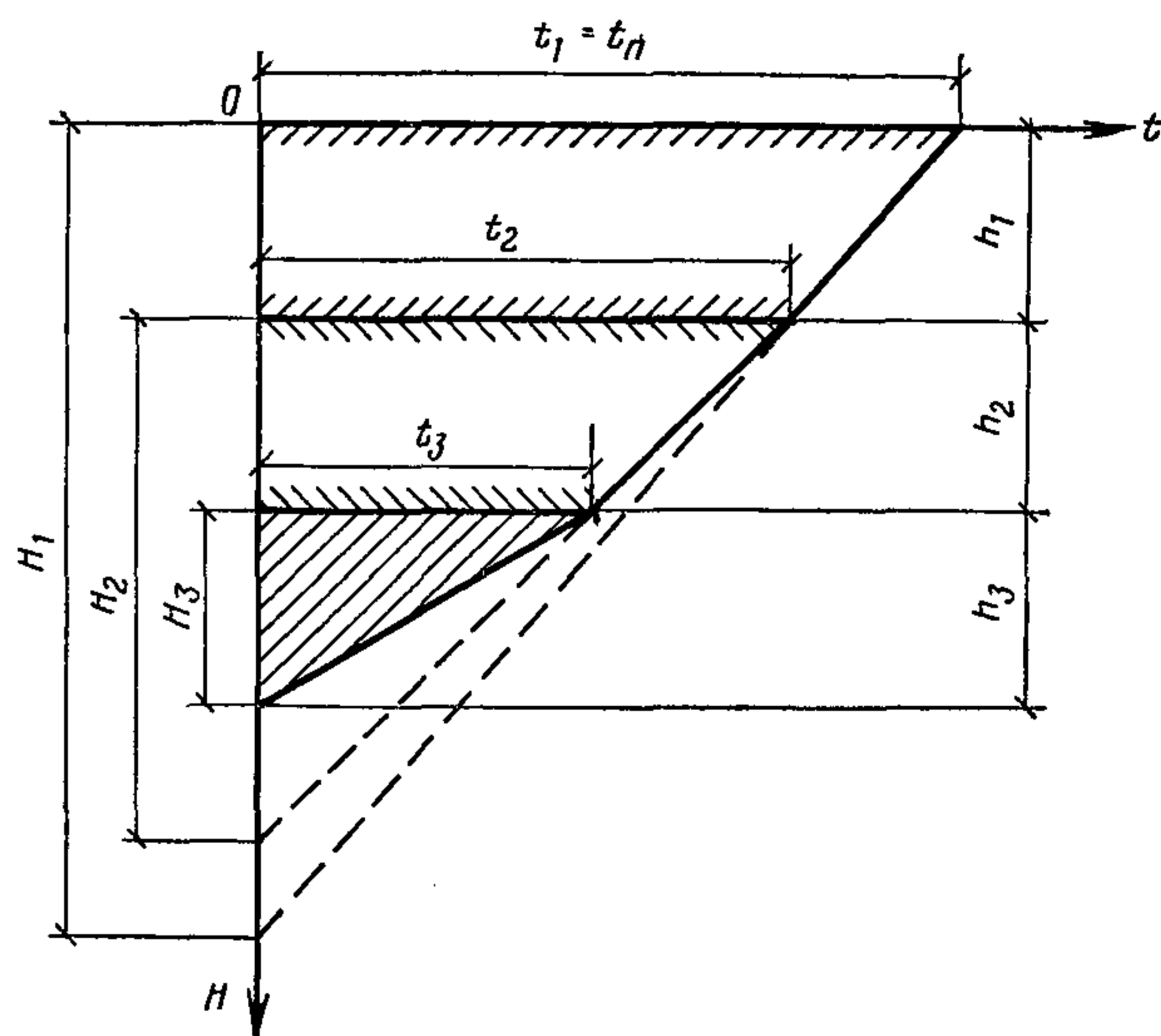
Рис. 10. Расчетная схема распределения температур по глубине многослойного грунтового массива к концу оттаивания
