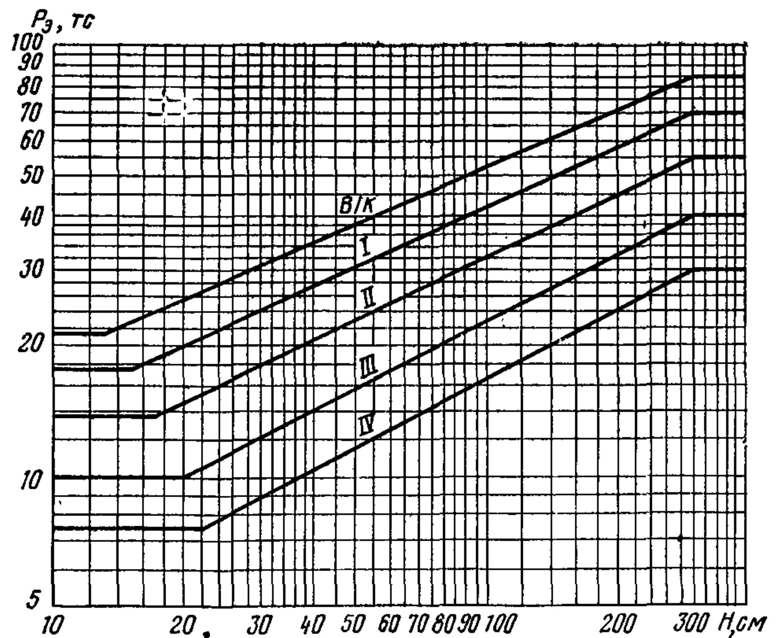
Рис. 7. График для определения эквивалентной одноколевой нагрузки P_0 (I, II, III и IV — категории нормативных нагрузок)
