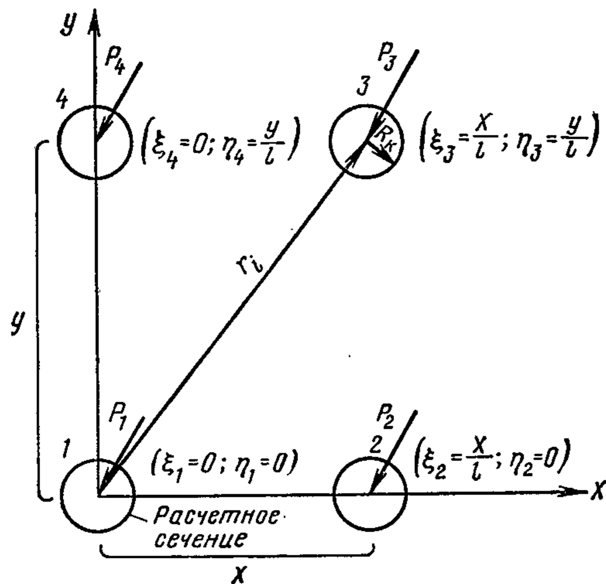
Рис. 4. Расчетная схема параметров загрузки опор воздушного судна
