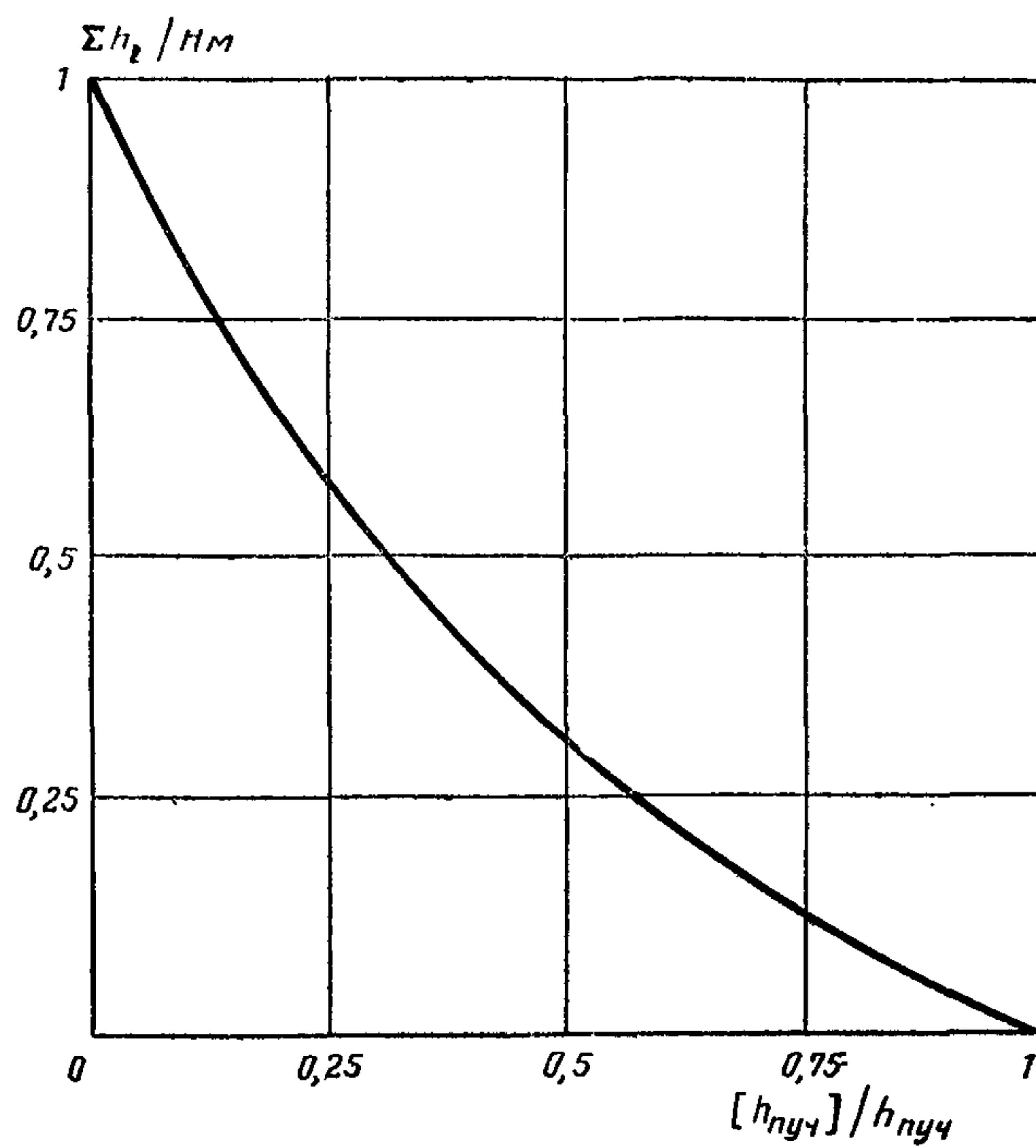
Рис. 13. График для определения общей толщины пучинистого грунта, подлежащего замене непучинистым грунтом
