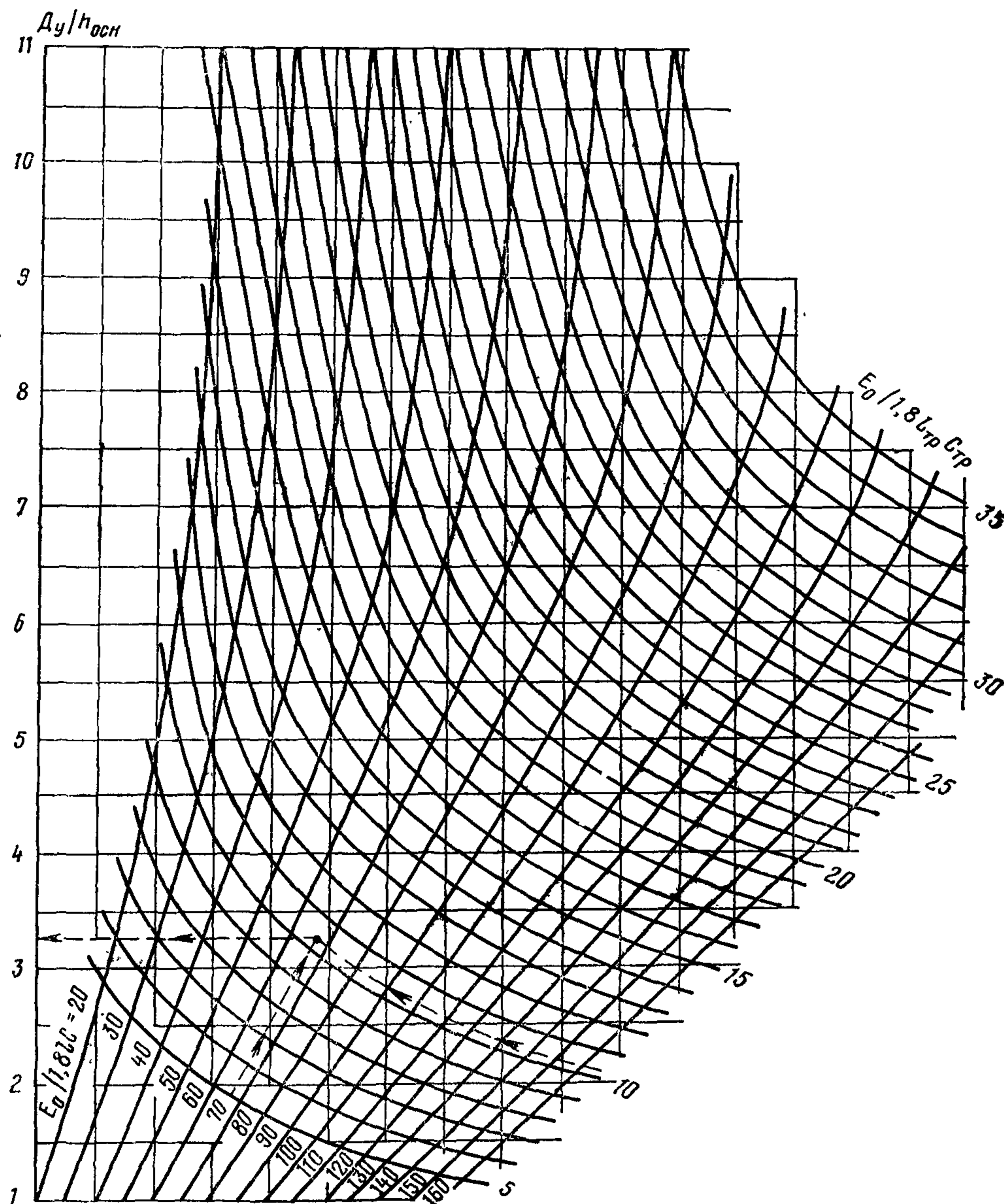
Рис. 26. Номограмма для определения соотношения условного диаметра площади передачи нагрузки на основание D_y и толщины искусственных оснований h_{осн} из материалов, обработанных вяжущими, под железобетонные монолитные и сборные покрытия
