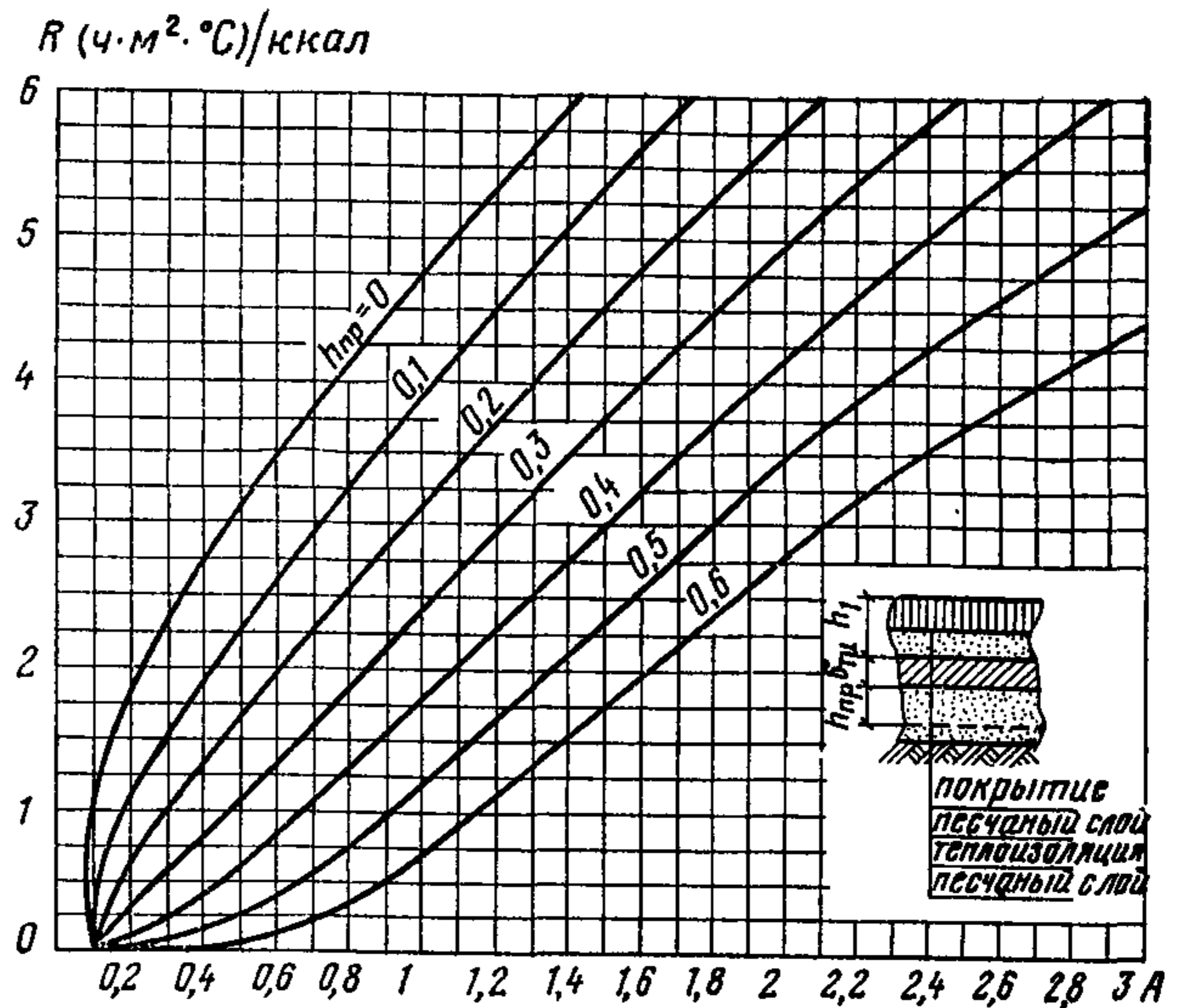
Рис. 11. Номограмма для определения термического сопротивления теплоизоляции R
