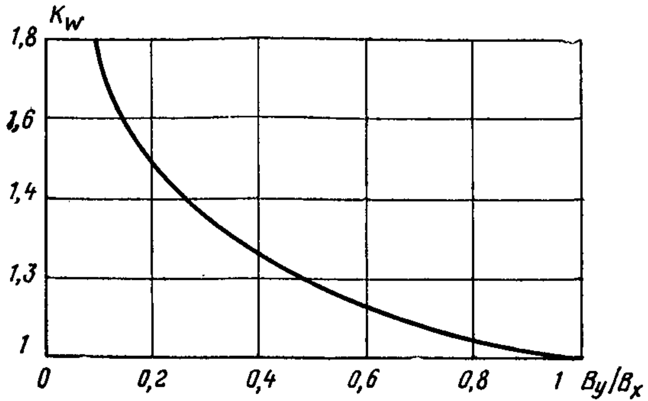
Рис. 20. График для определения коэффициента k_w
