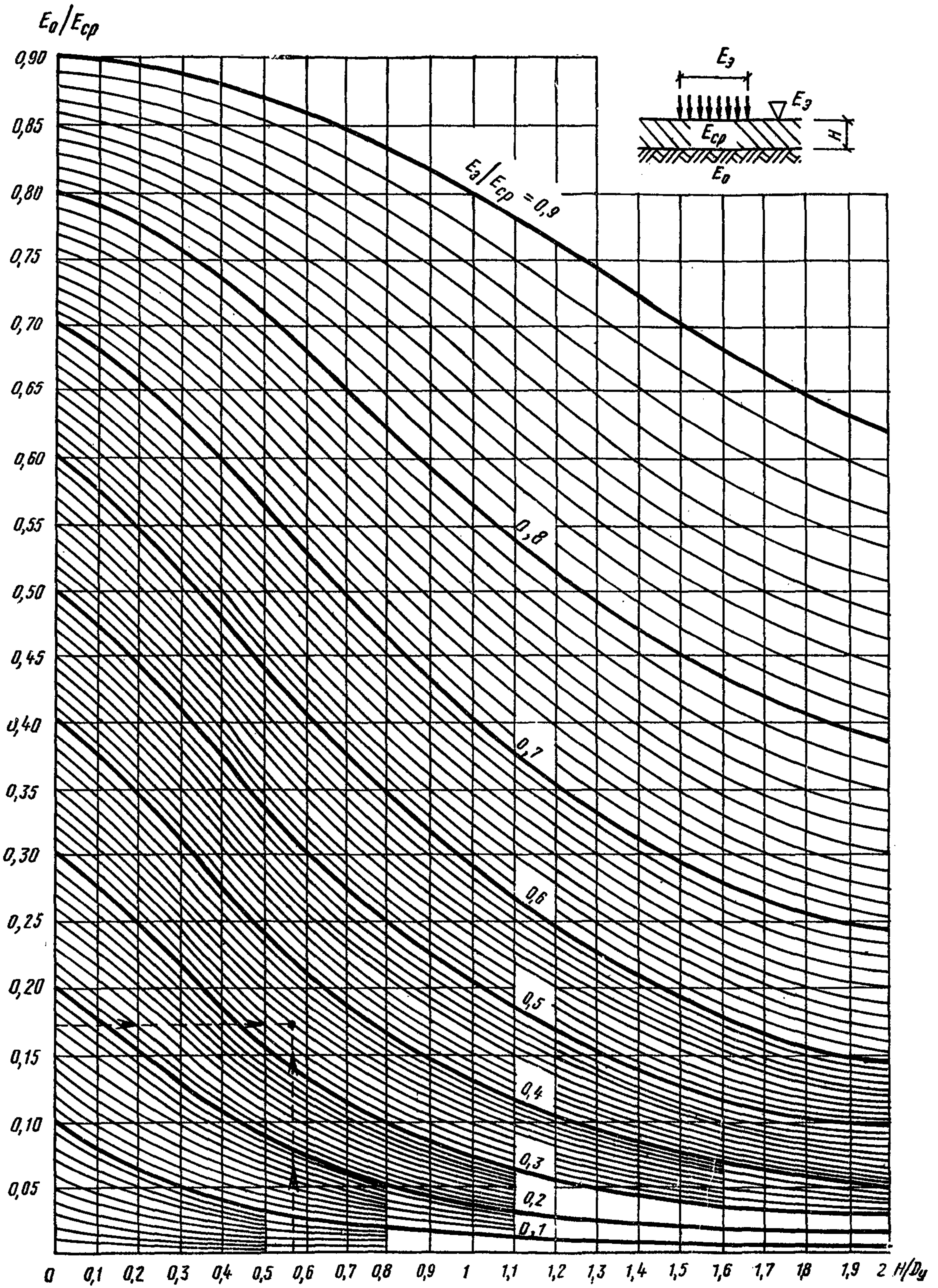
Рис. 8. Номограмма для определения эквивалентного модуля упругости E_e конструкции нежесткого покрытия
