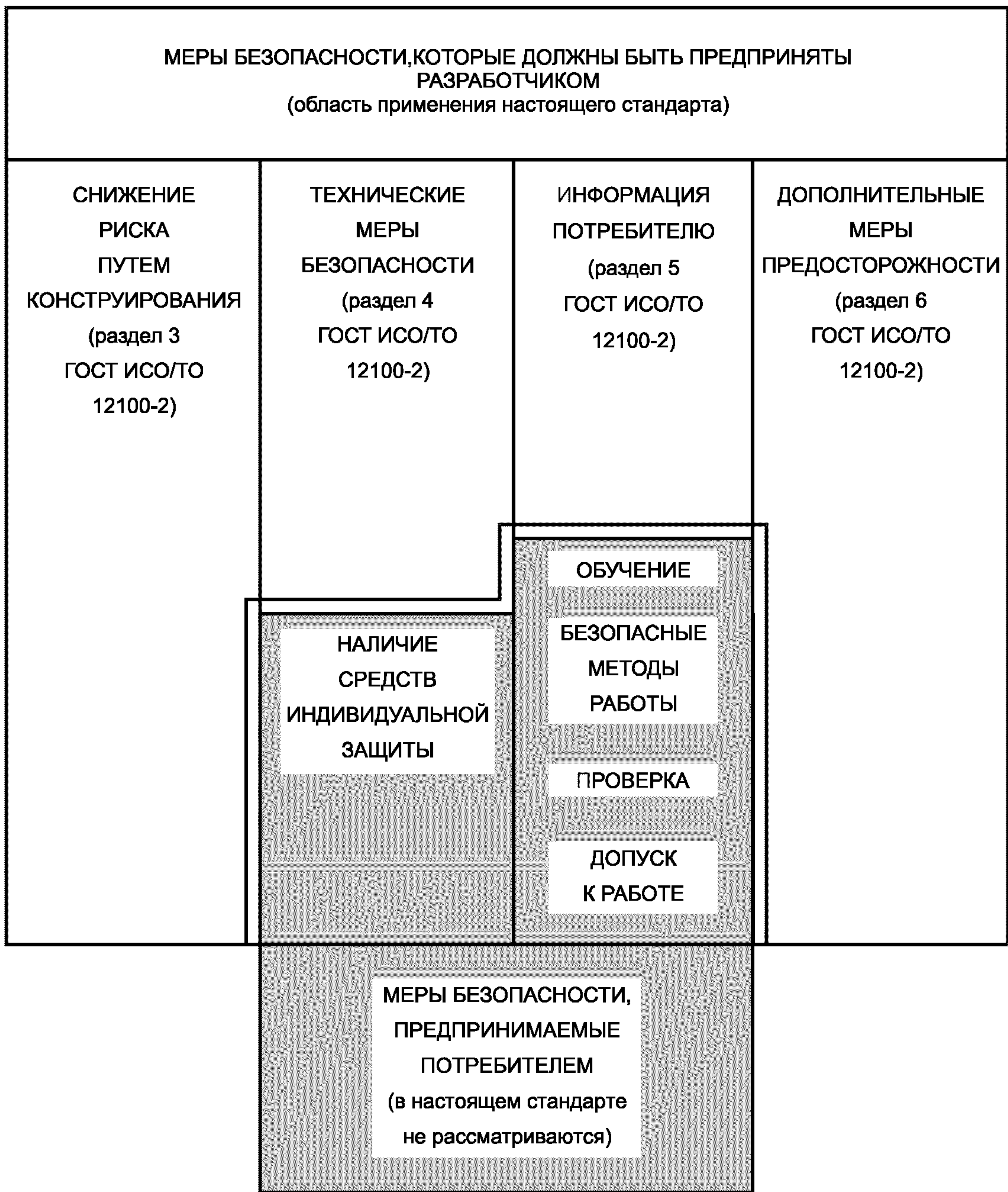
Рисунок 2 — Взаимосвязь между обязанностями разработчика и потребителя машин
