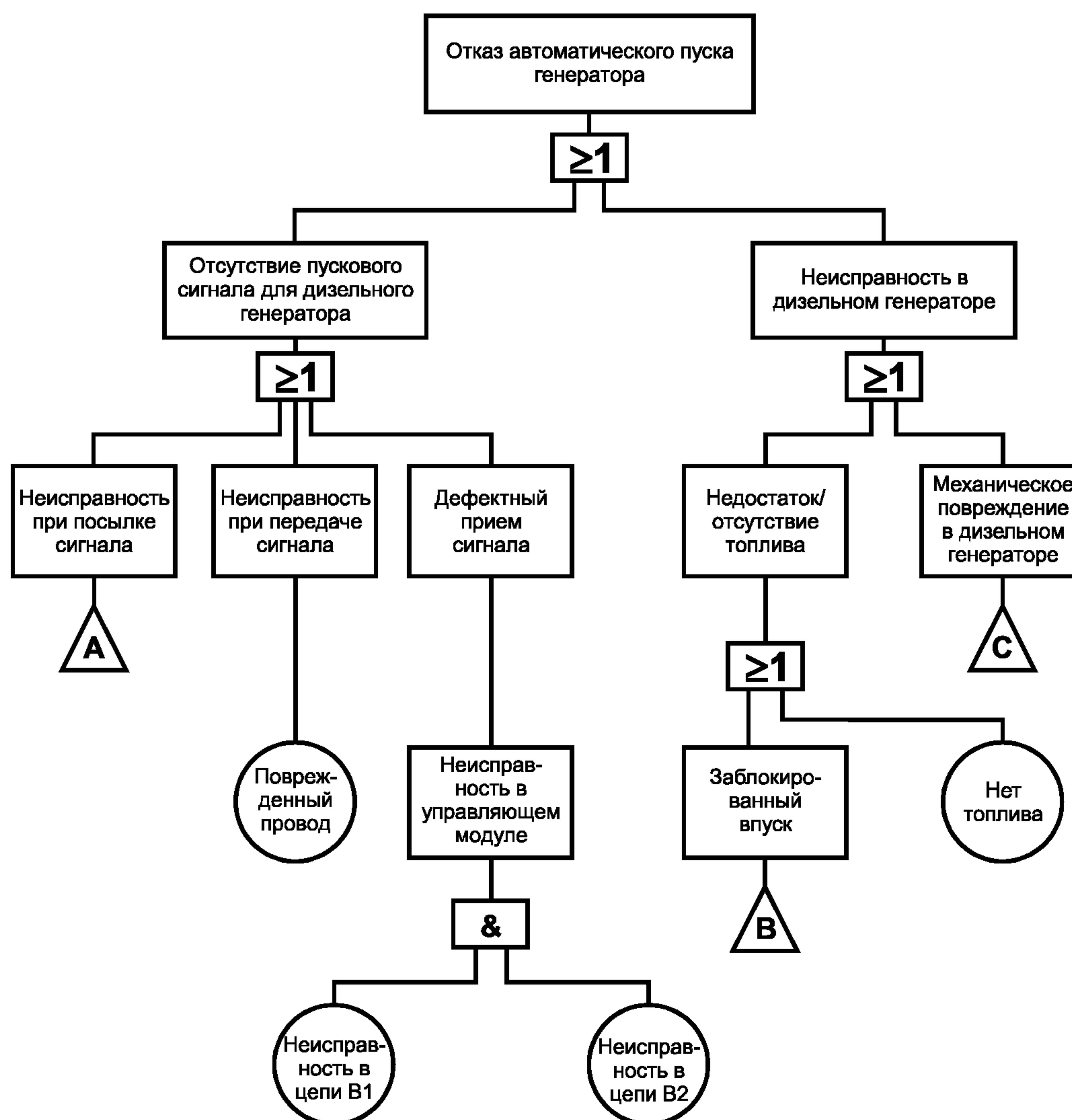
Рисунок А.1 — Пример «дерева неисправностей»
