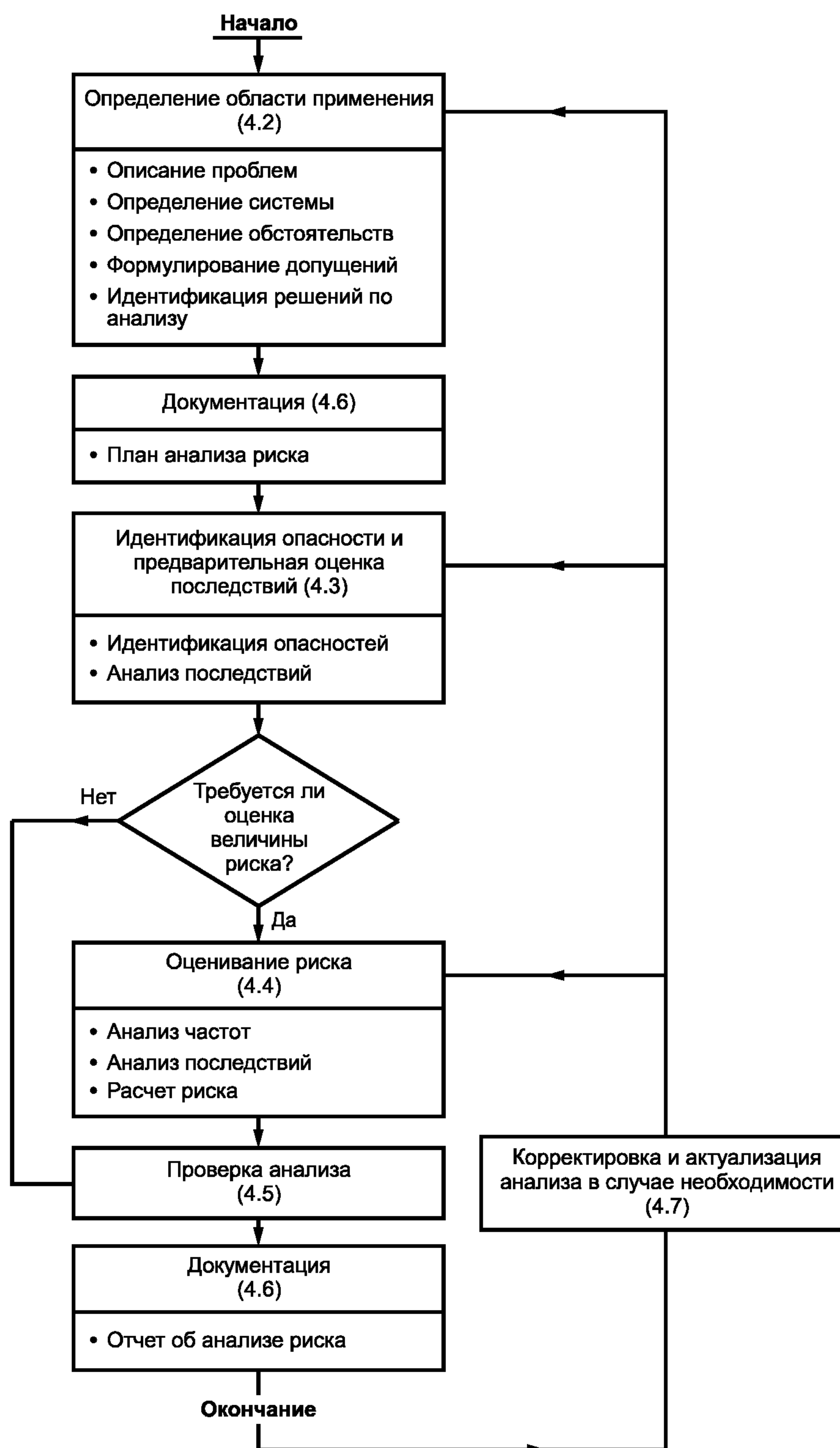
Рисунок 2 — Процесс анализа риска (раздел 4)
