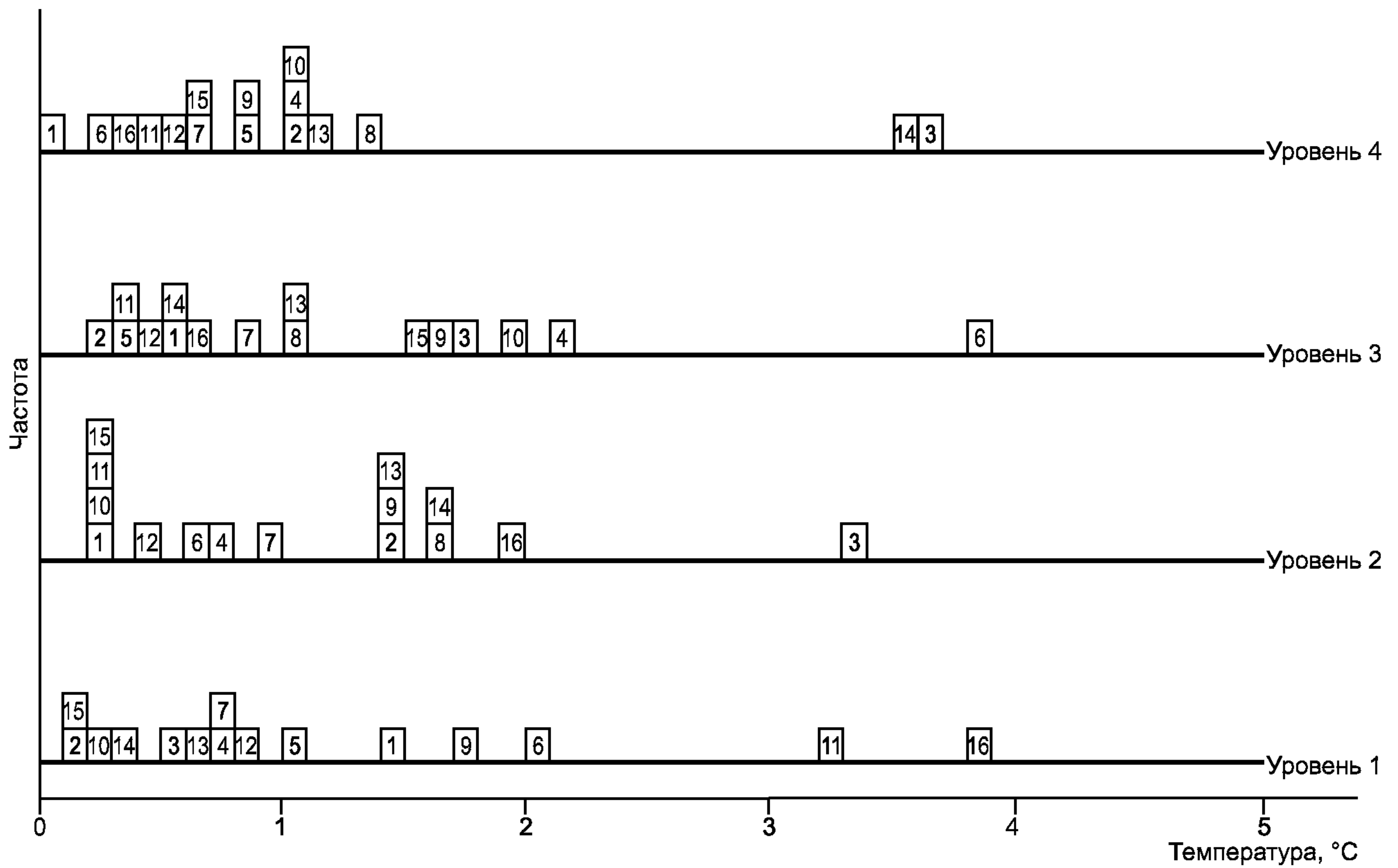
Рисунок В.6 — Точка размягчения смолы. Абсолютные расхождения в базовых элементах
