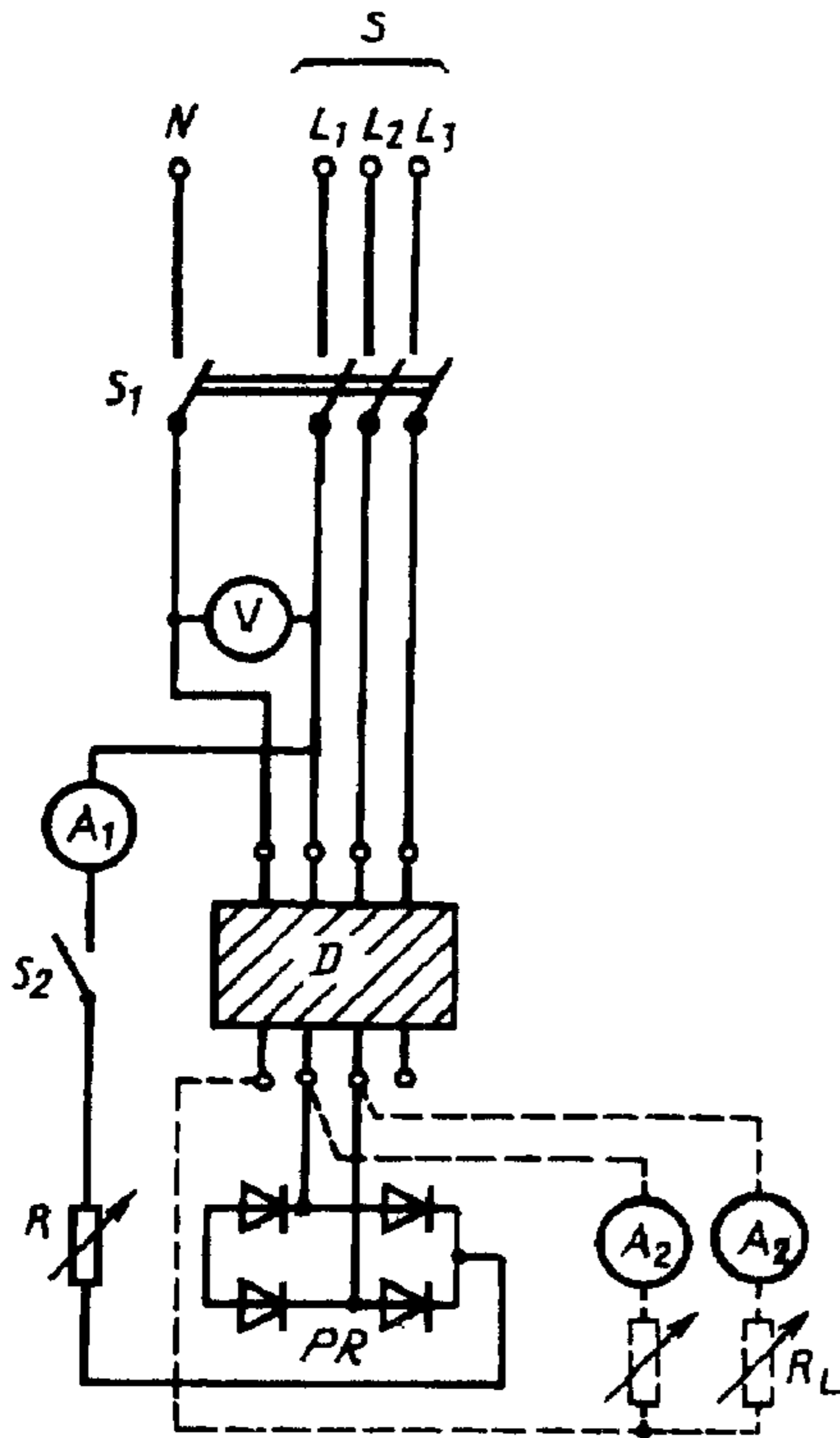
A_1 — амперметр действующих значений A_2 — амперметр переменного тока, D — испытуемое УЗО D PR — двухполупериодная мостовая схема на линейном напряжении, R — регулируемый резистор для дифференциального тока R_L — активная нагрузка, S — источник переменного тока S — многополюсный выключатель, S_2 — однополюсный выключатель, V — вольтметр
