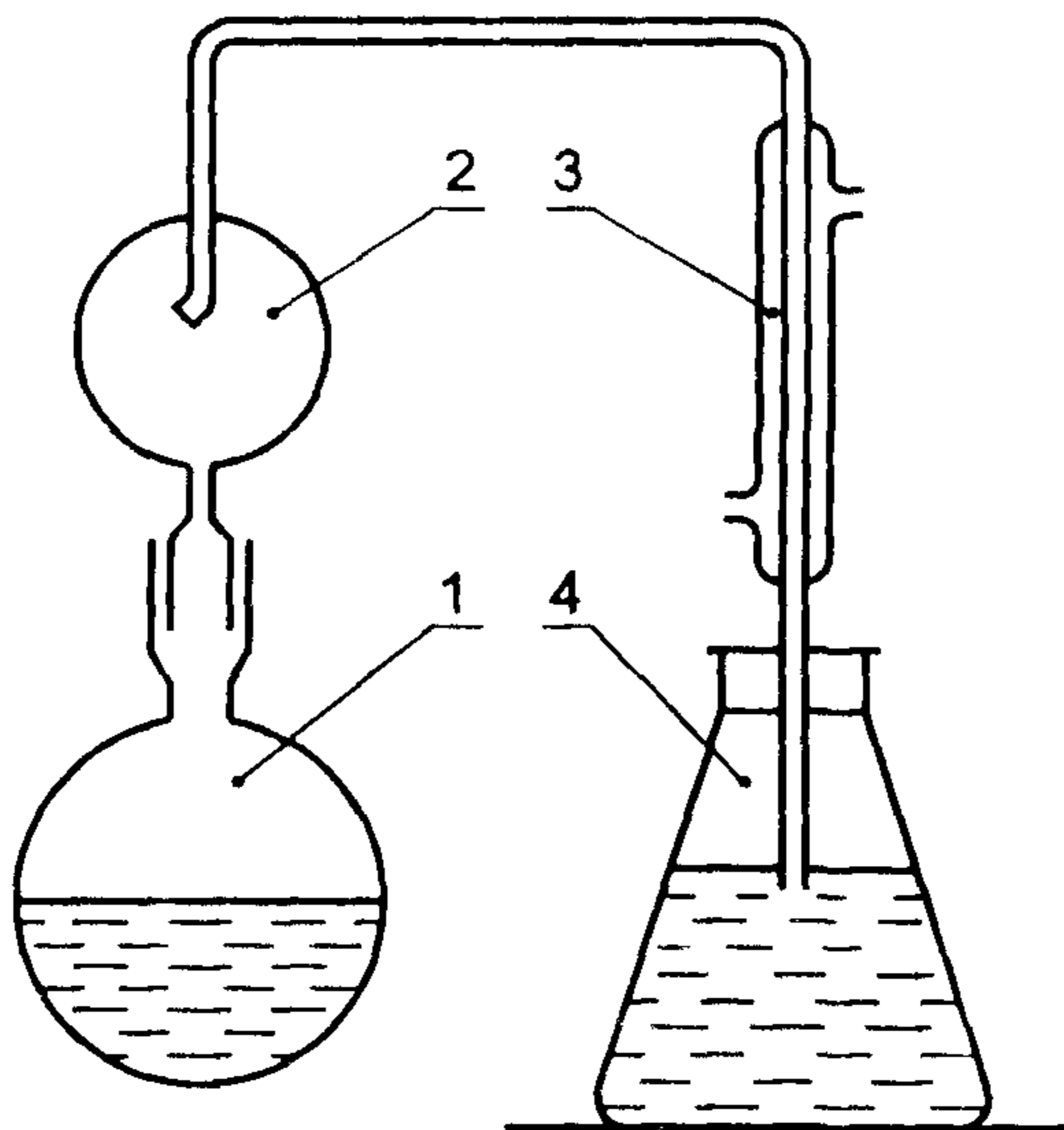
1 — круглодонная колба, 2 — каплеуловитель, 3 — холодильник, 4 — приемная колба
