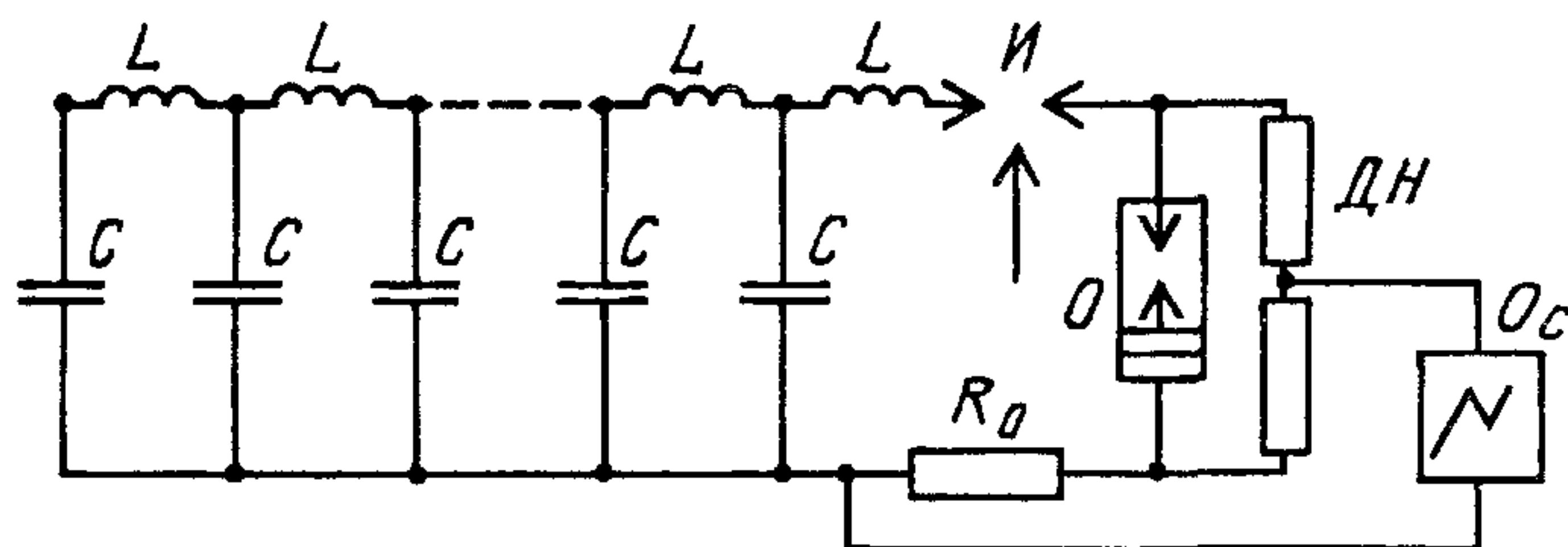
C, L — емкости и индуктивности генератора импульсов тока большой длительности соответственно; И — управляемый искровой промежуток; R_0 — шунт для измерения тока; O — испытуемый образец или разрядное сопротивление; ДН — делитель напряжения; Oс — осциллограф
