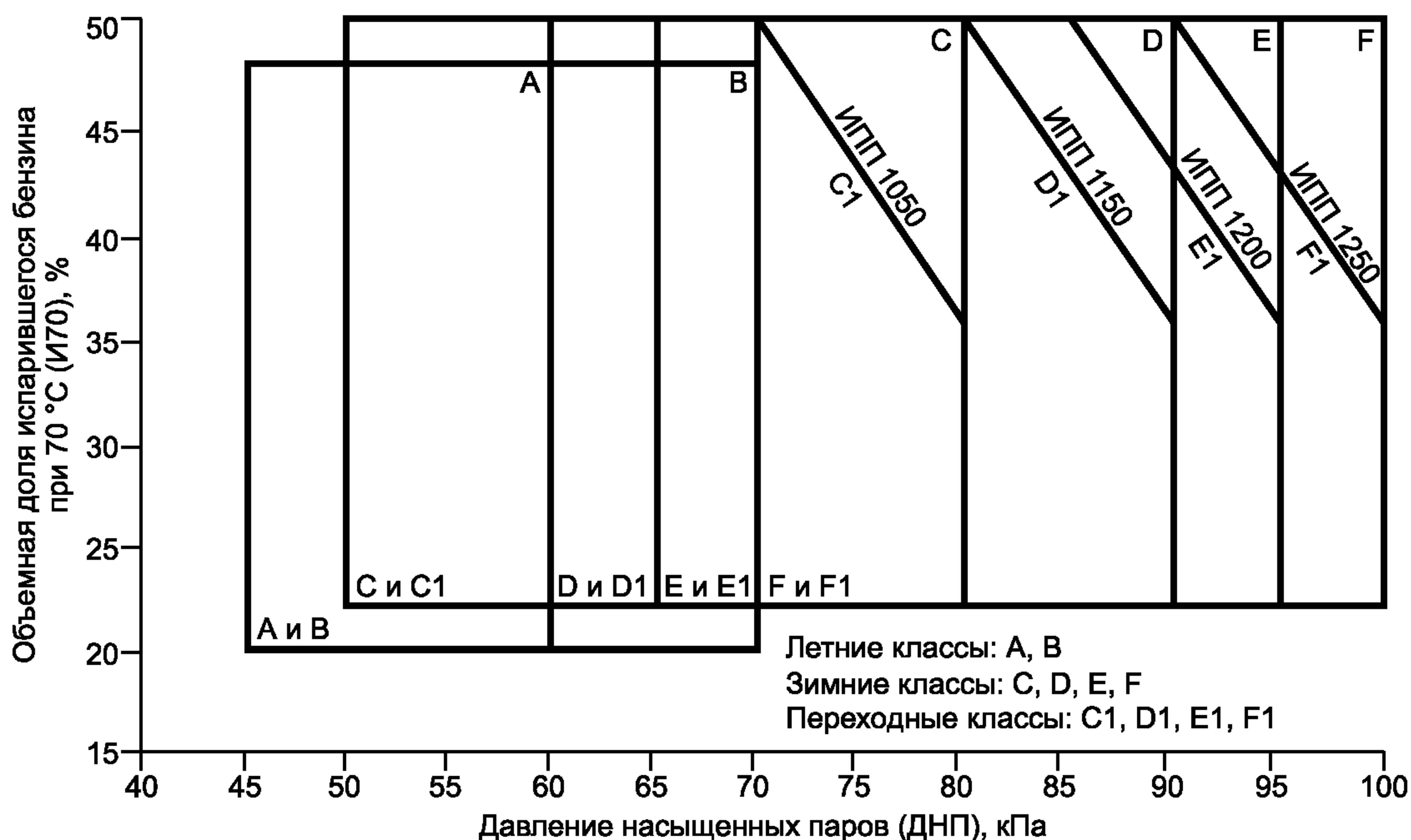
Рисунок 1 — Диаграмма определения классов испаряемости бензинов
