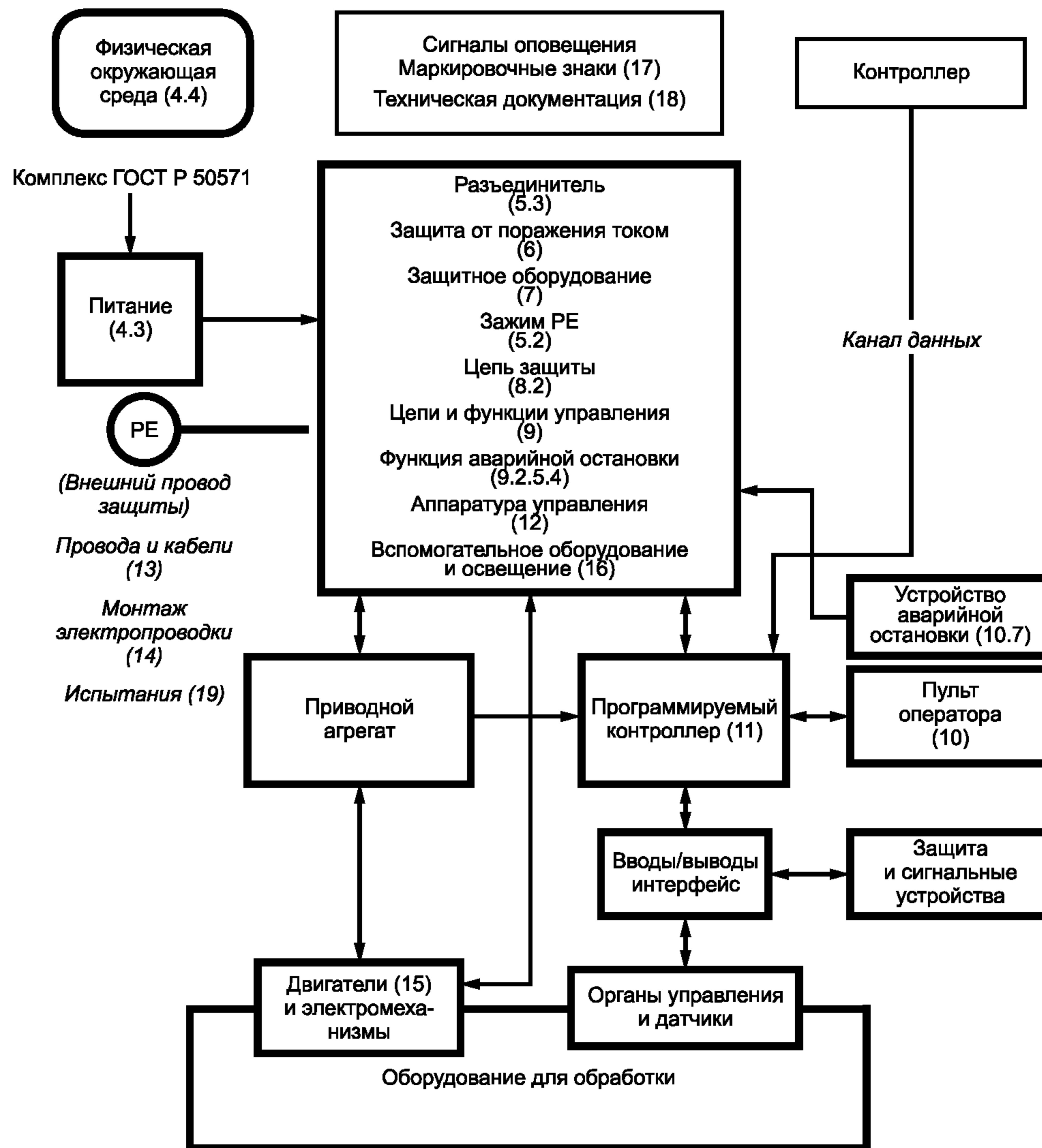
Рисунок 2 — Функциональная схема типовой машины
