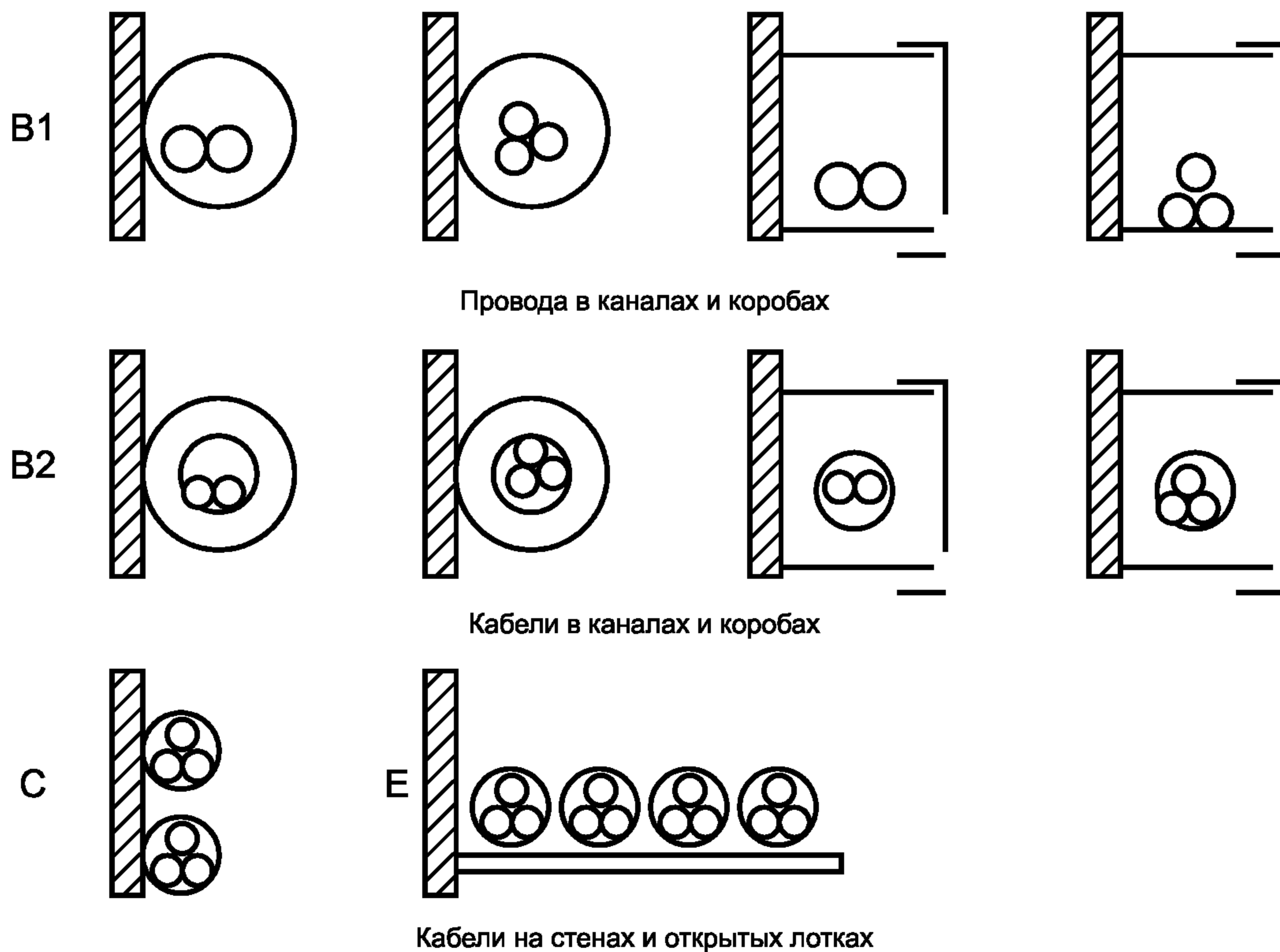
Рисунок С.1 — Методы укладки кабелей и проводов
