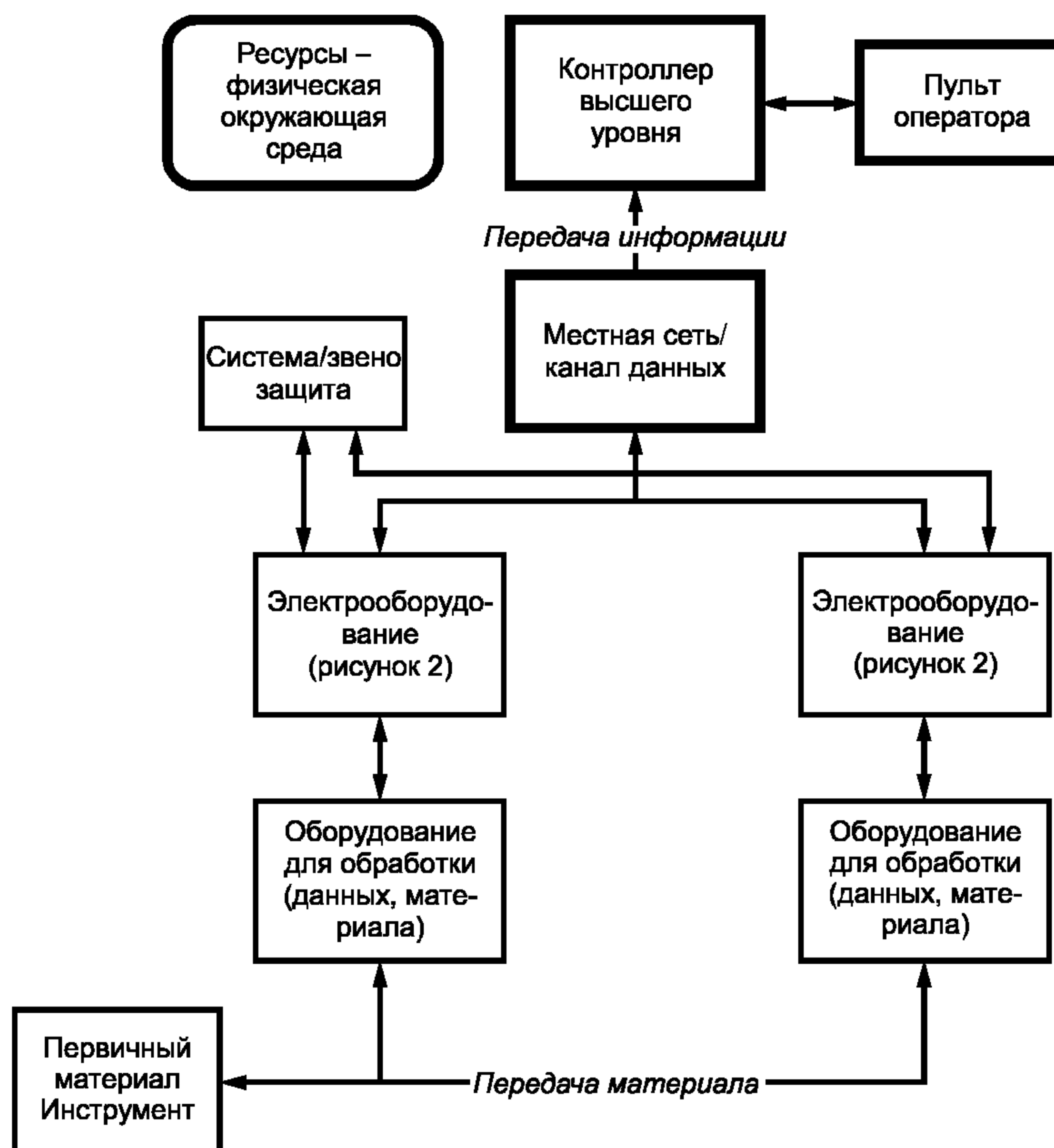
Рисунок 1 — Функциональная схема типовой производственной системы
