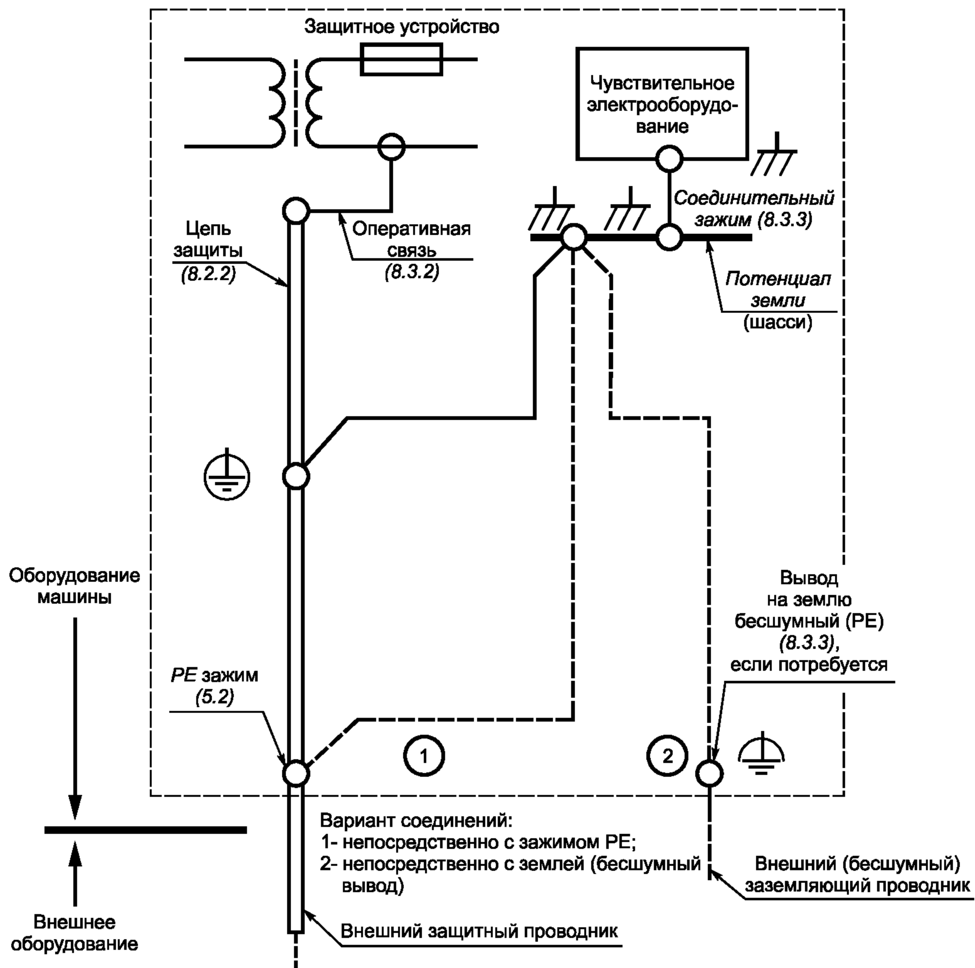
Рисунок 3 — Пример эквипотенциального соединения машины
