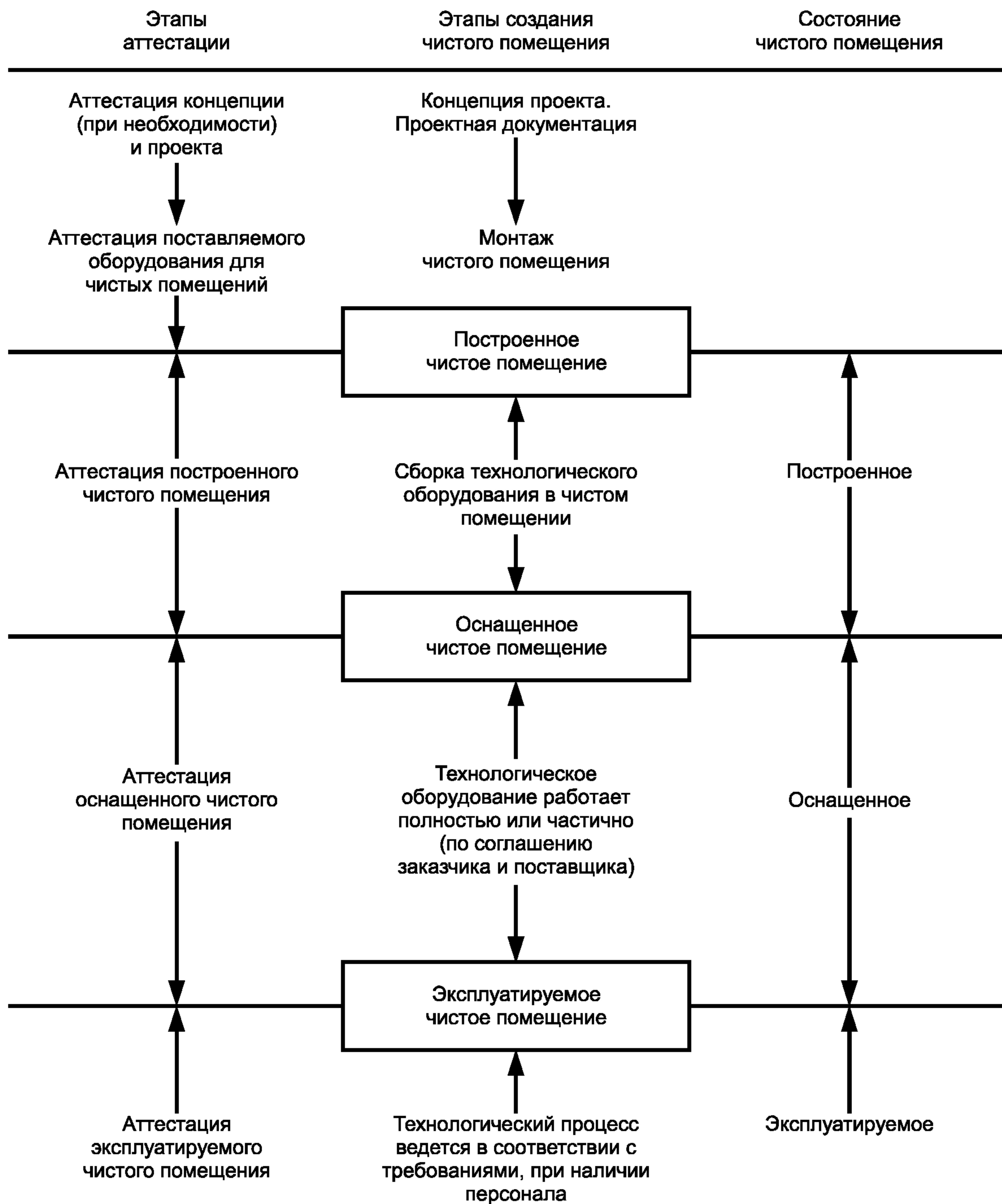
Рисунок С.1 — Аттестация чистых помещений
