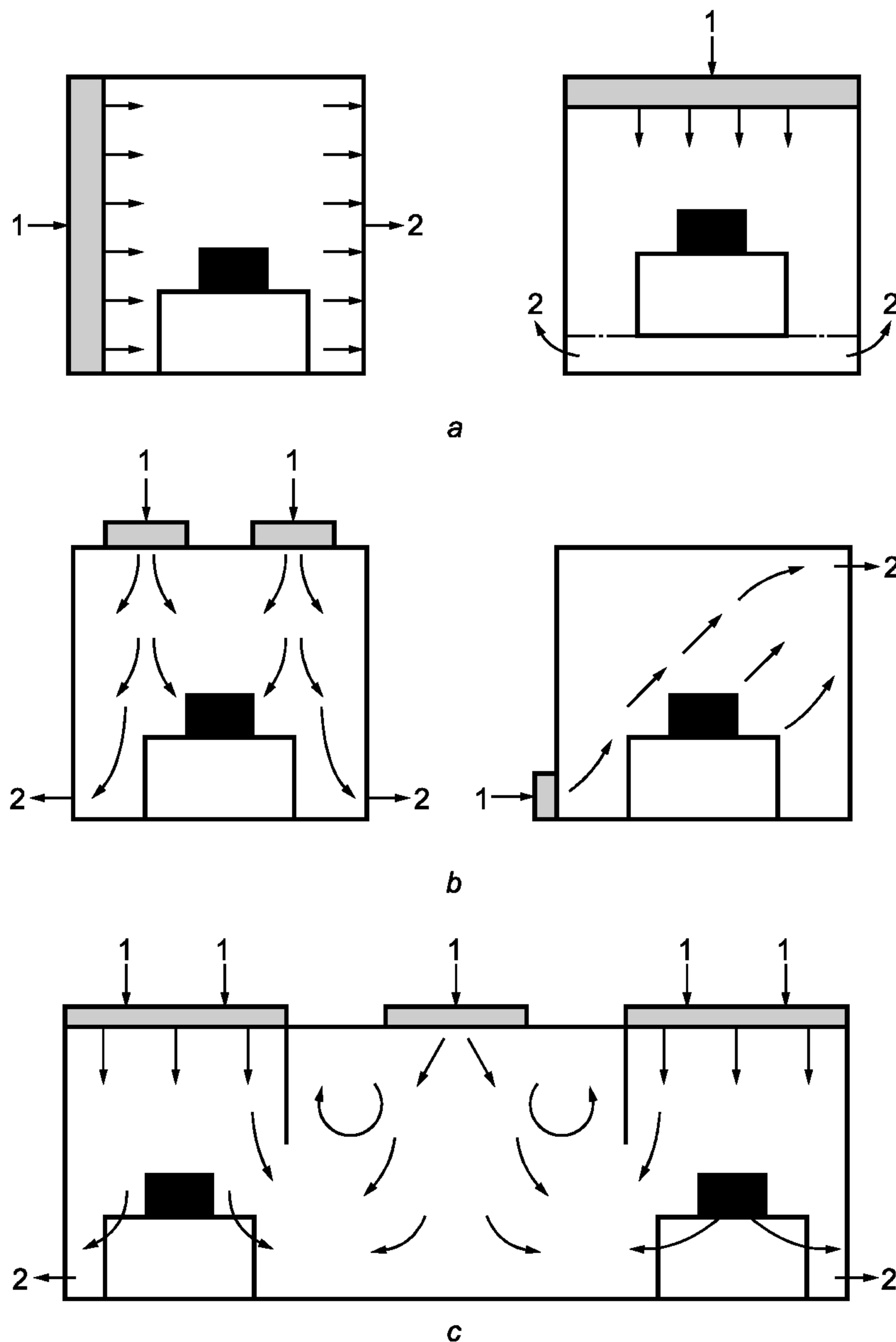
a — одинаправленный поток воздуха; b — неоднаправленный поток воздуха; c — смешанный поток воздуха; 1 — приточный воздух; 2 — вытяжной воздух
