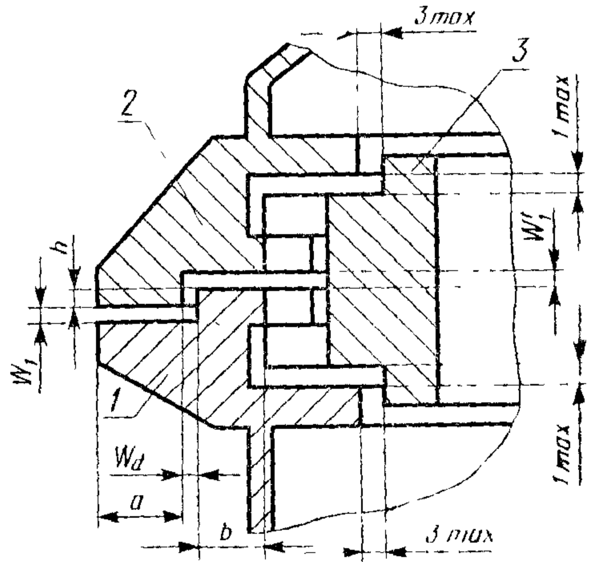
Лабиринтное взрывонепроницаемое соединение
