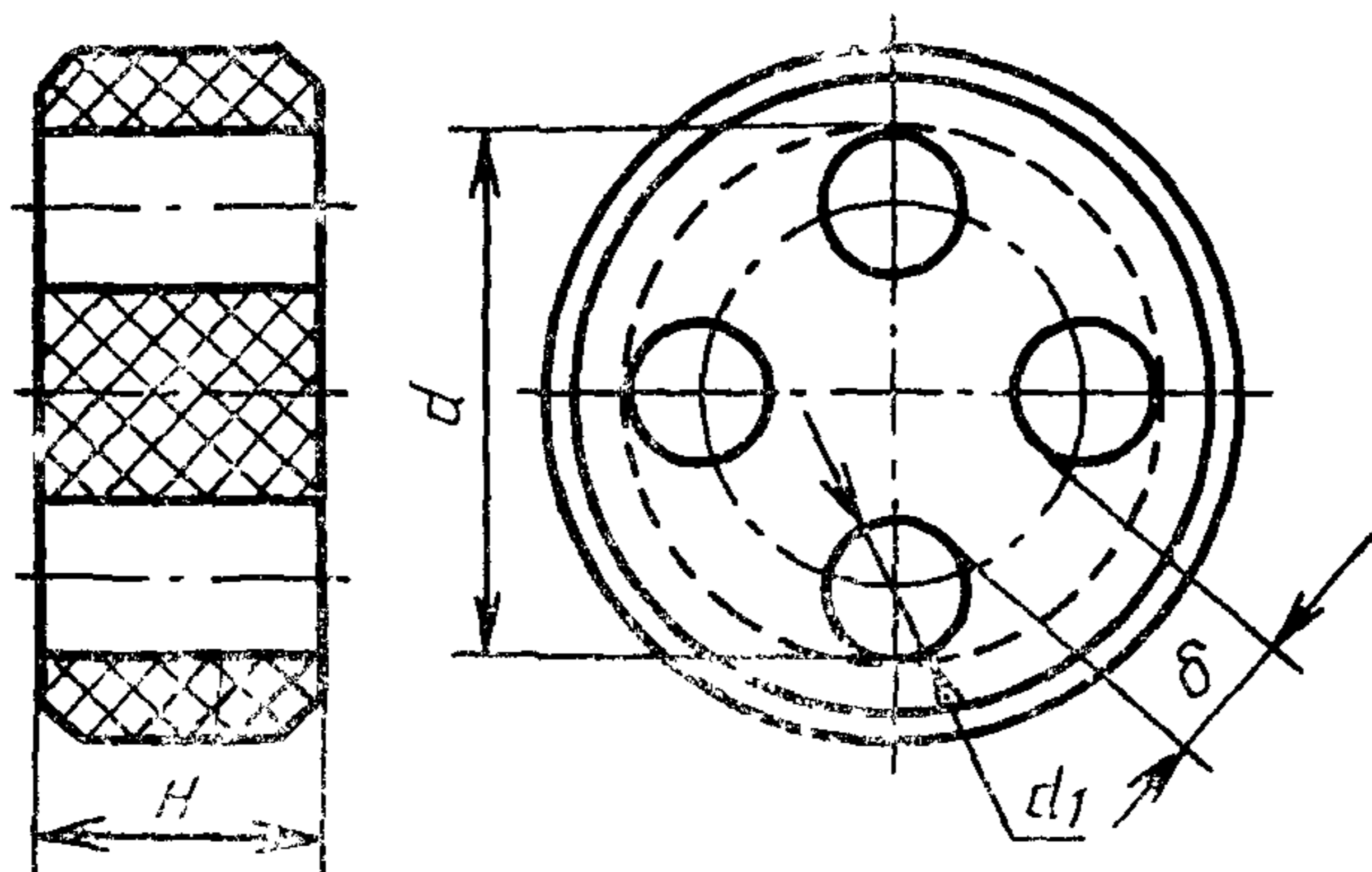
d — диаметр проходного отверстия в расточке кабельного ввода (см. черт. 12), d_1 — диаметр отверстия в уплотнительном кольце, \delta — минимальное расстояние между отверстиями, H — высота уплотнительного кольца
