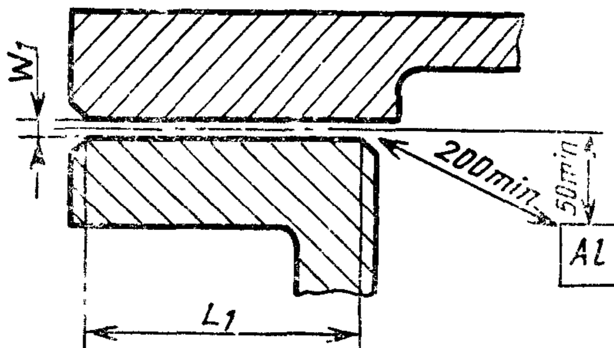
Плоское взрывонепроницаемое соединение
