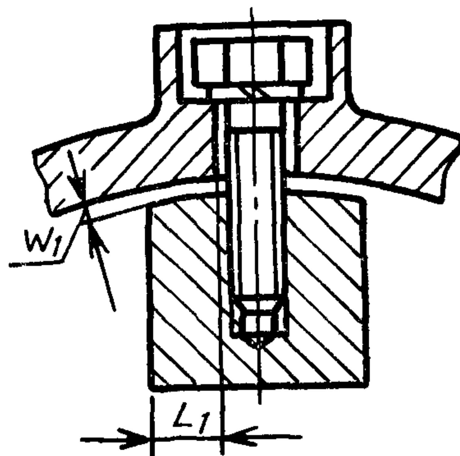
Вариант крепления полюсов электрических машин
