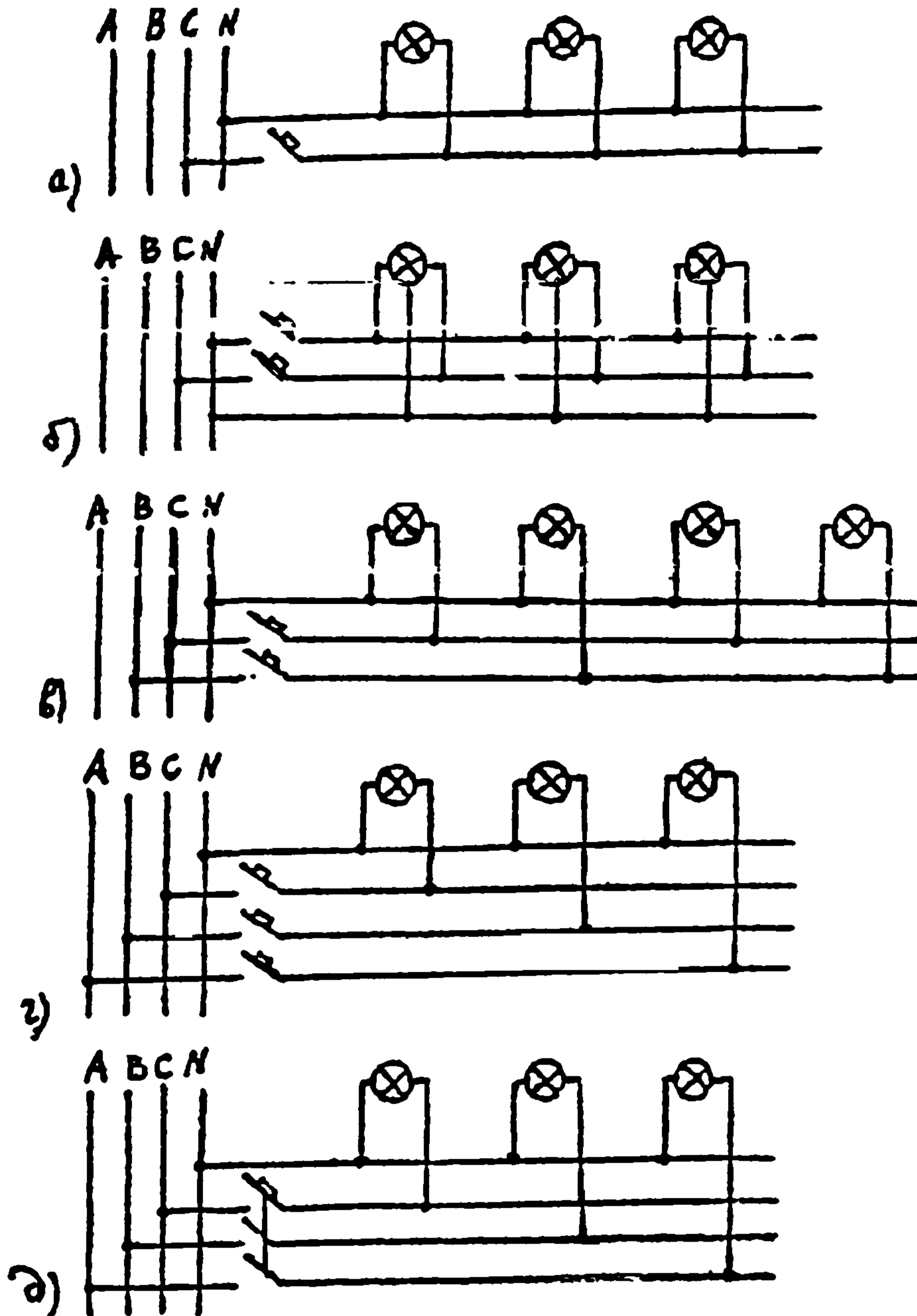
Рис. 1. Схемы групповых линий при системах напряжения напряжения 660/380, 380/220 и 220/127 В и питания ОП напряжением соответственно 380, 220 и 127 В.
