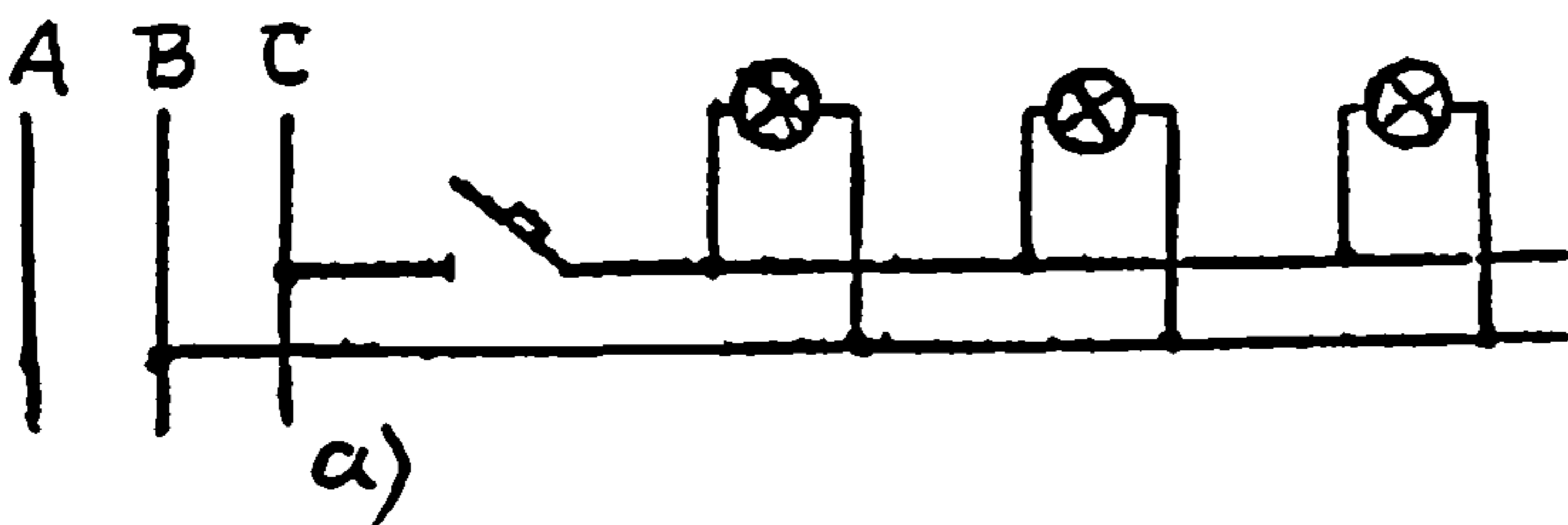
Рис.3. Схемы групповых линий при системах 3х220 и 220/127 В при питании ОП напряжением 220 В и отсутствии необходимости заземления или зануления ОП.
