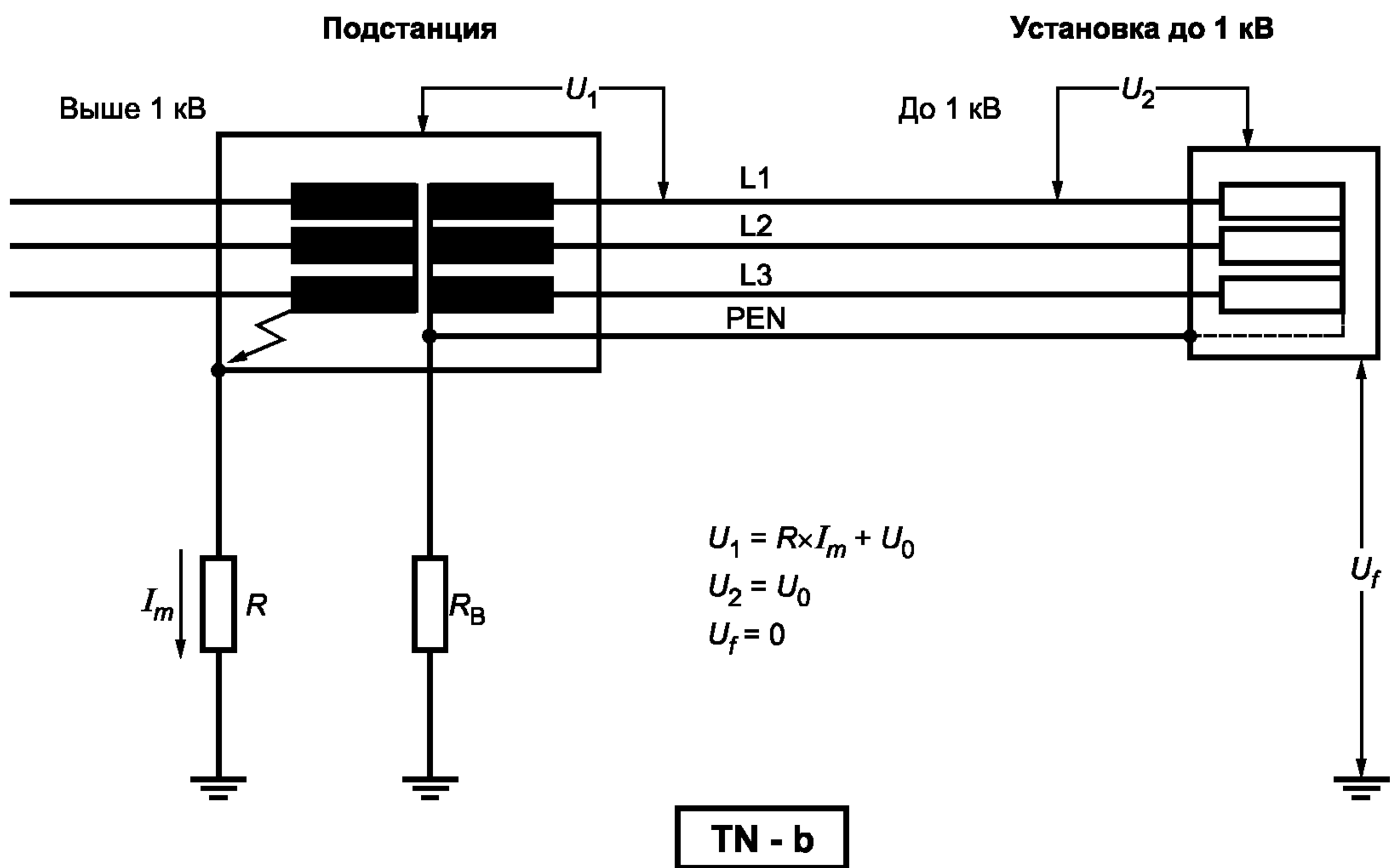
Рисунок 44В — TN-системы
