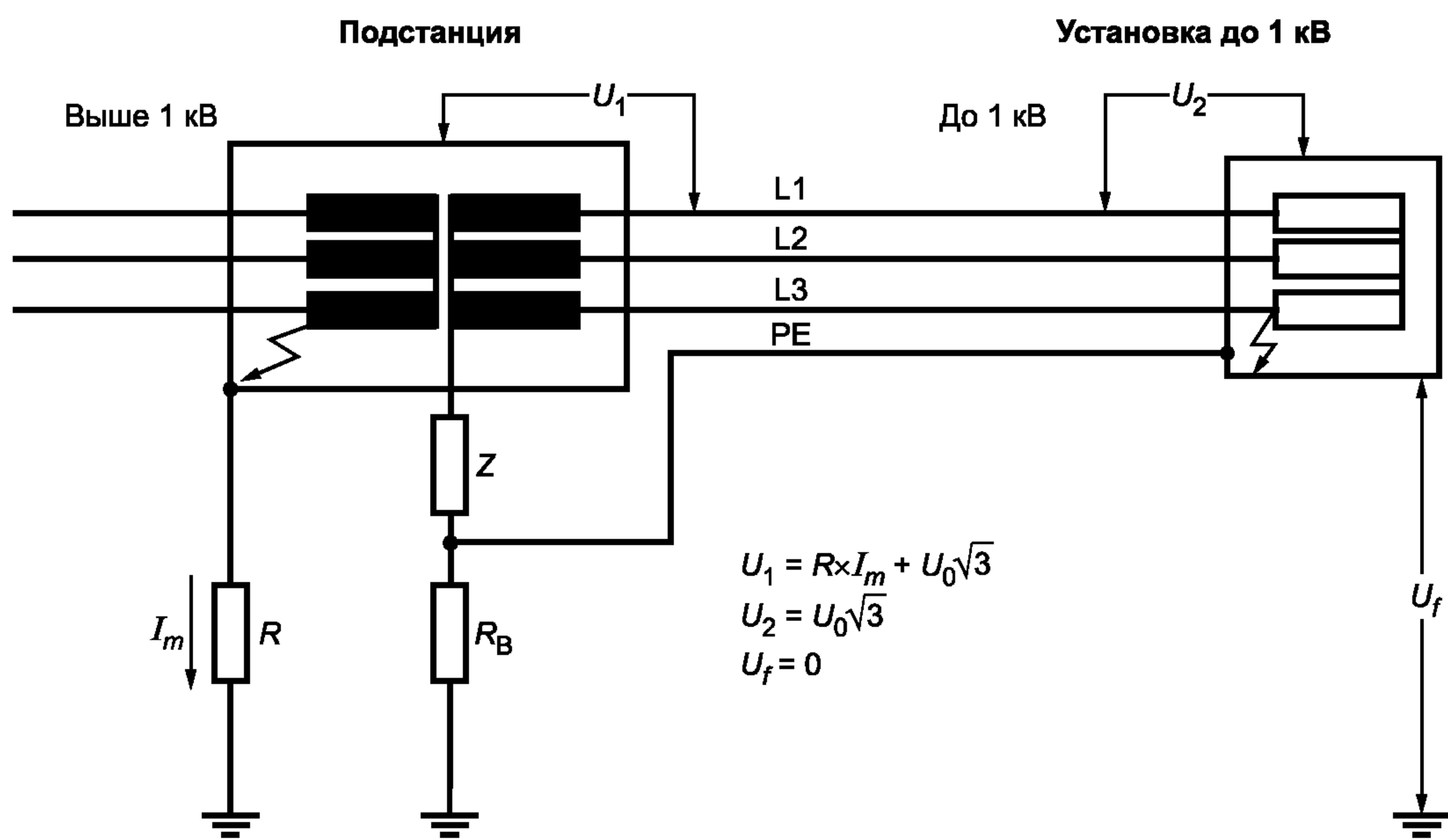
2) Первое замыкание в установке до 1 кВ
