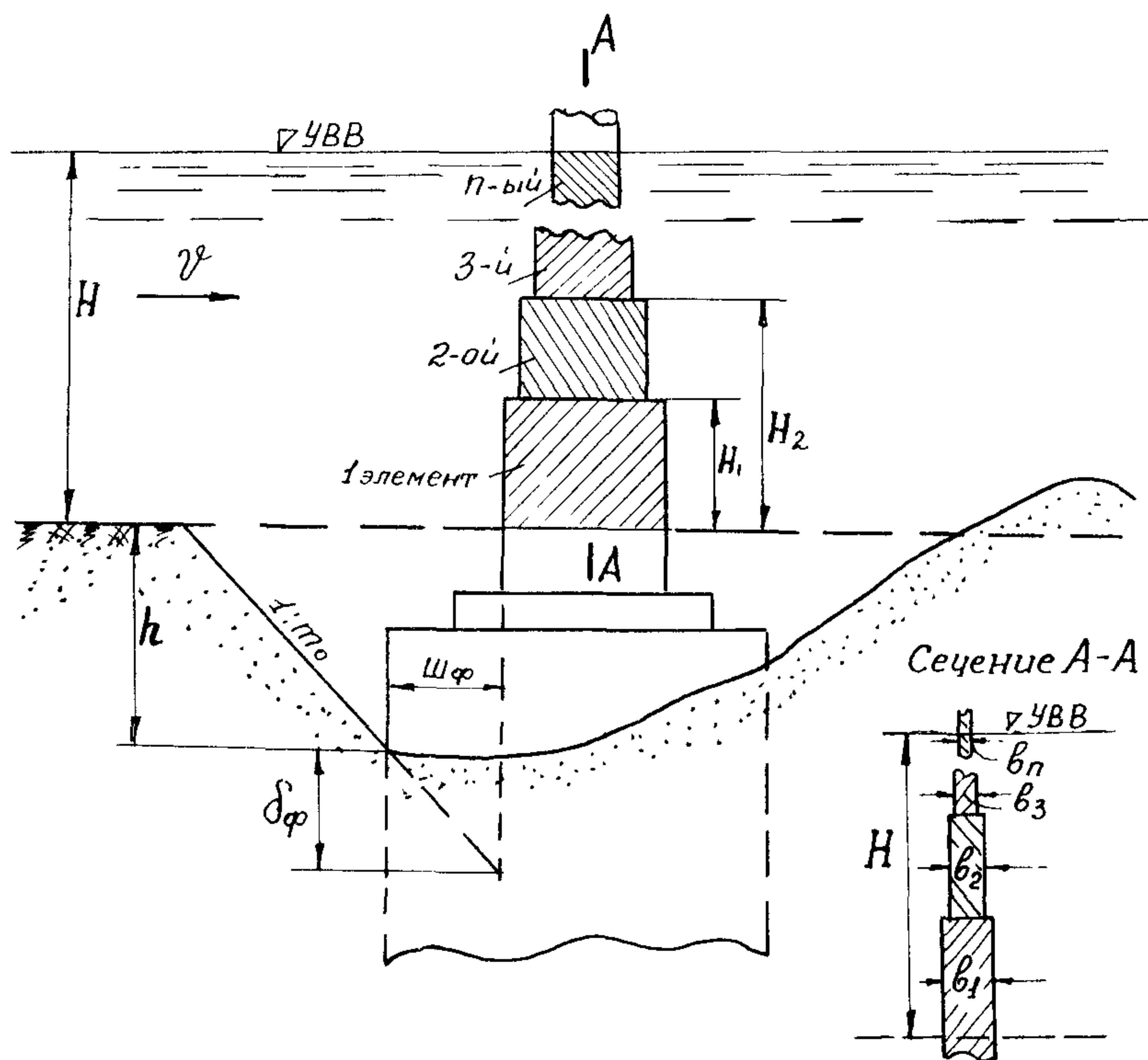
Рис. 10.7. Разделение опоры на элементы с постоянной шириной
