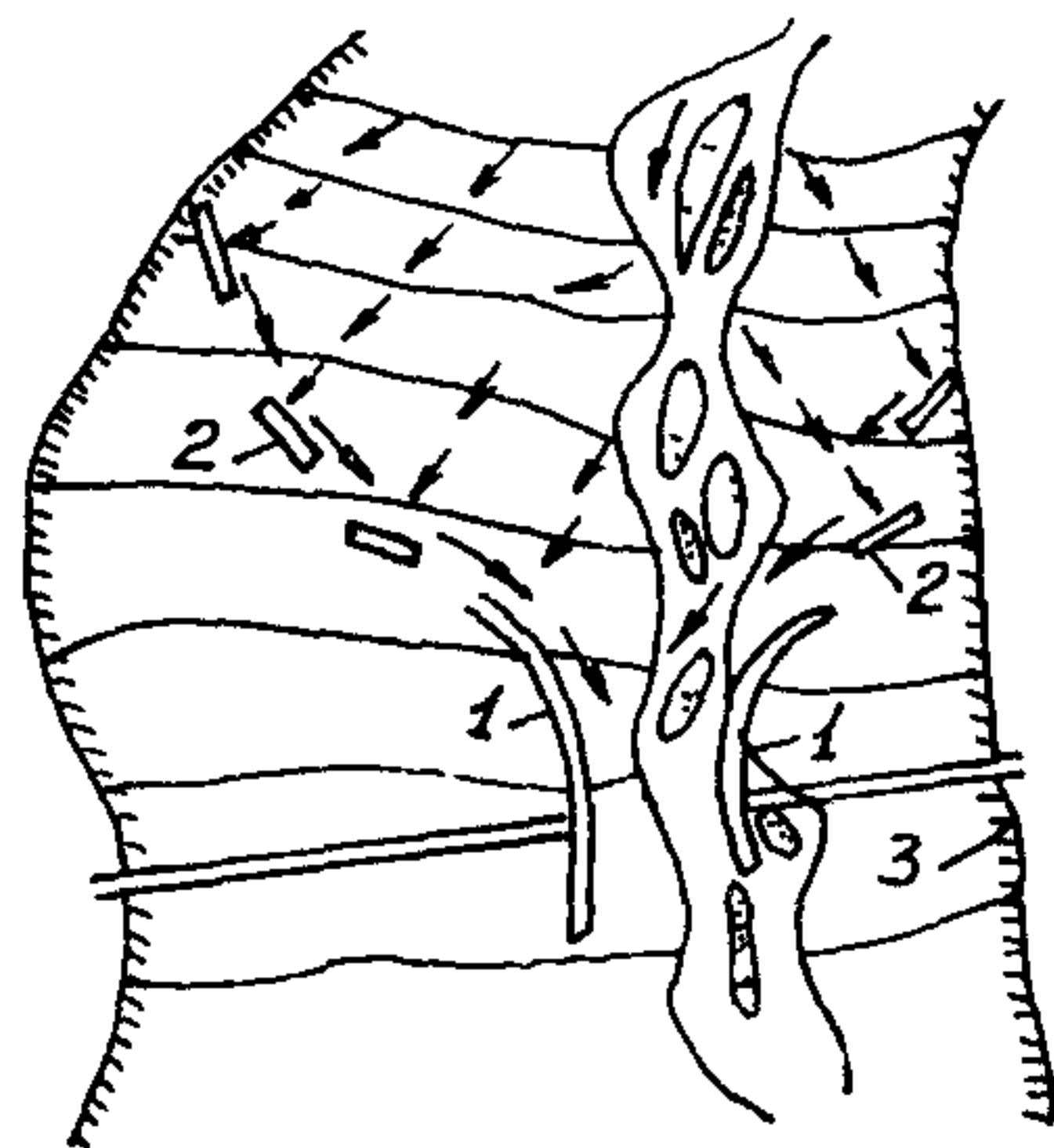
Рис 11.5 Регулирование потока дамбами и шпорами 1—дамбы, 2—шпоры 3—границы зоны блуждания
