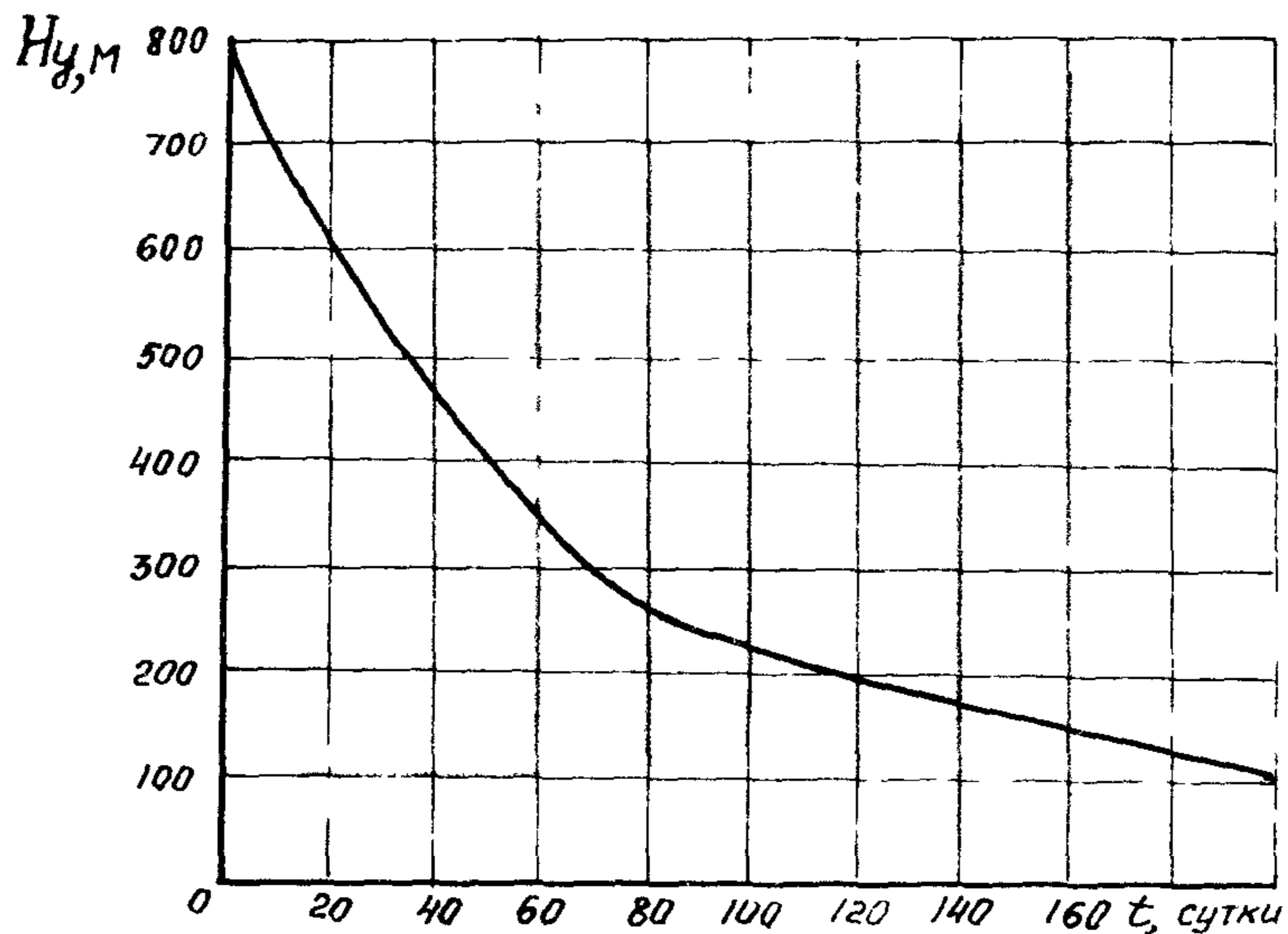
Рис. 7.12 График продолжительности стояния уровня N_y = f(t)
