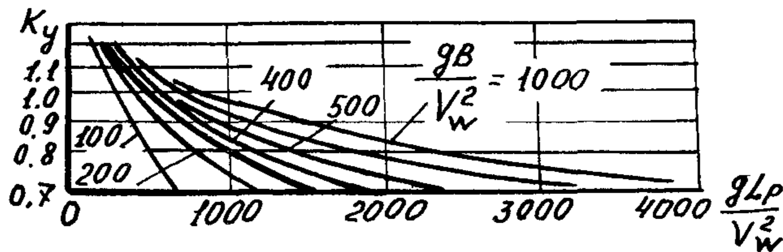
Рис 12.5 График значений коэффициента k_y
