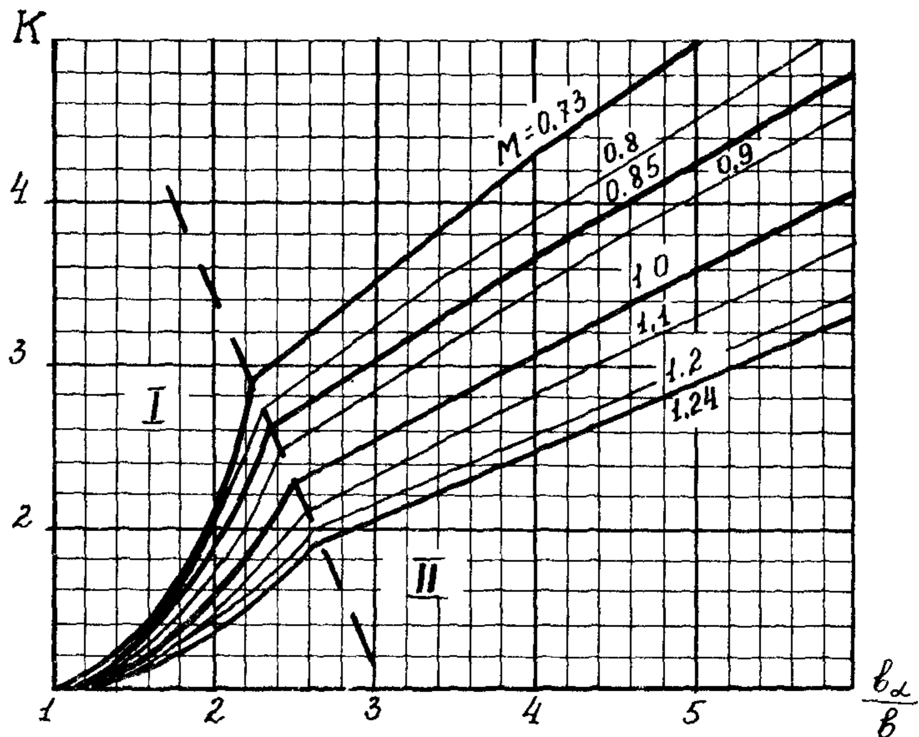
Рис 109 График для определения коэффициента косины К
