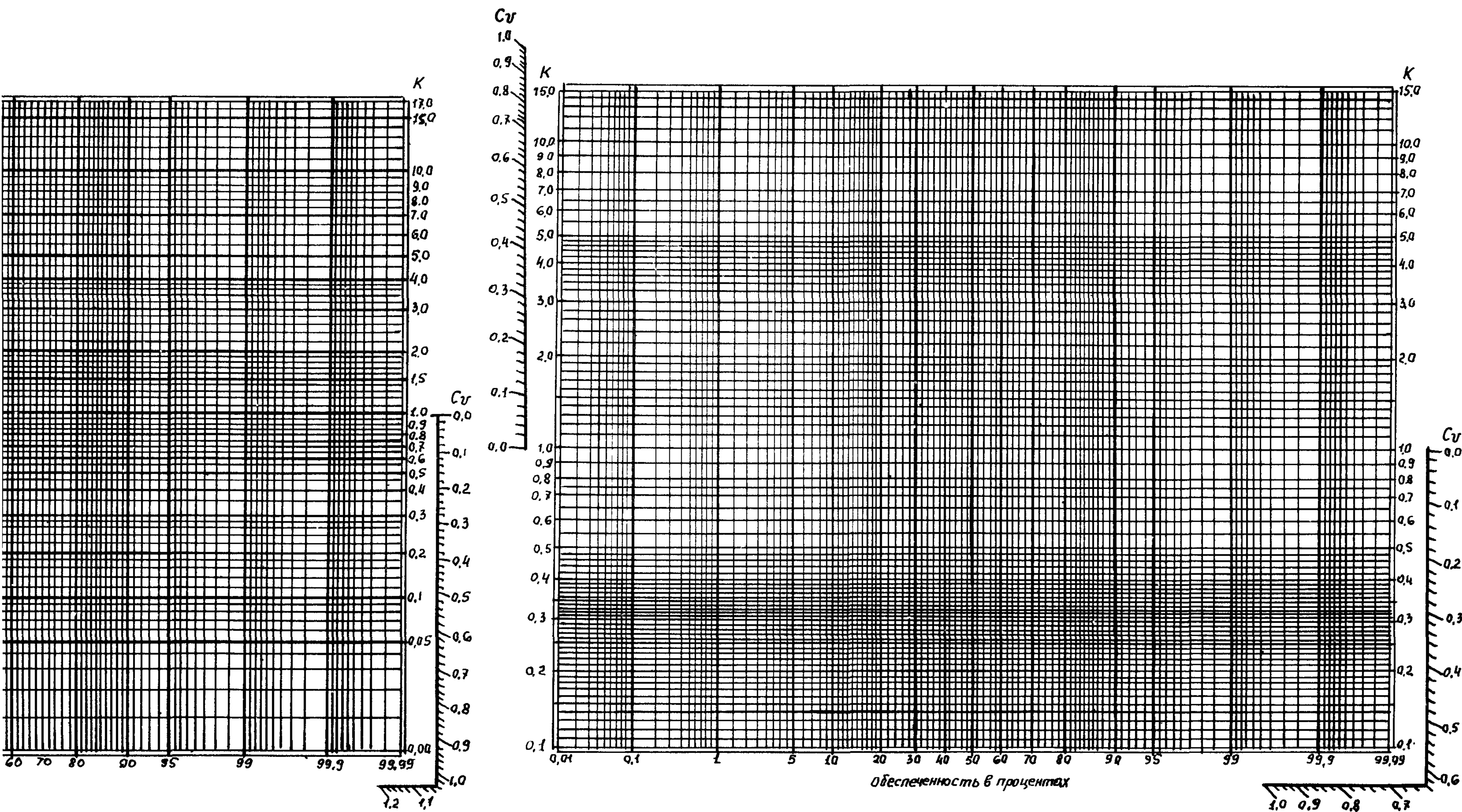
Рис 6 Клетчатка вероятности, спрямляющая кривые обеспеченности при C_s = 4,0C_v
