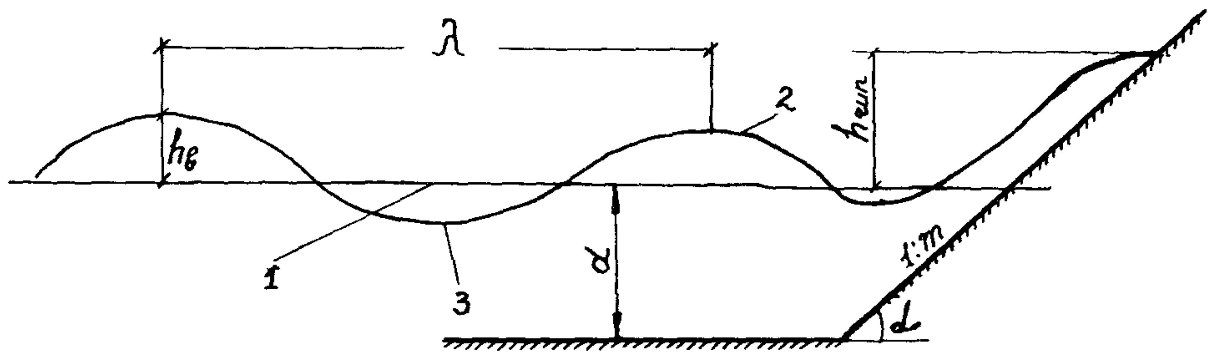
Рис 12.1. Профиль ветровой волны и ее наката на откос: 1—статический уровень; 2, 3—вершина и подошва волны
