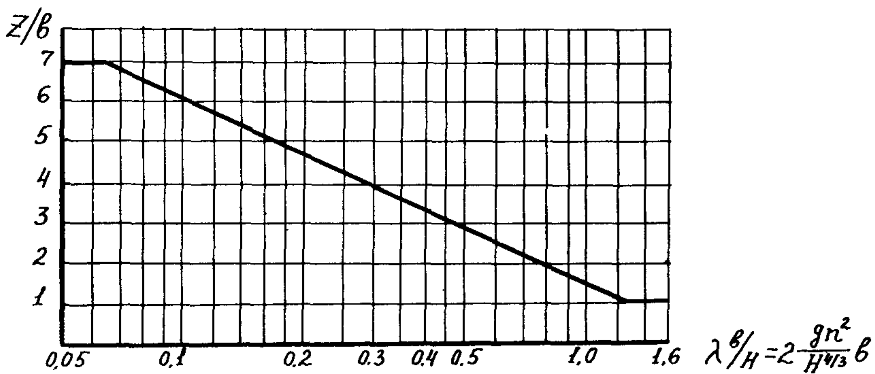
Рис 14.8. График для определения длины защитного фронта z , создаваемого поперечным сооружением расчетной длиной b на прямолинейных и слабокриволинейных участках
