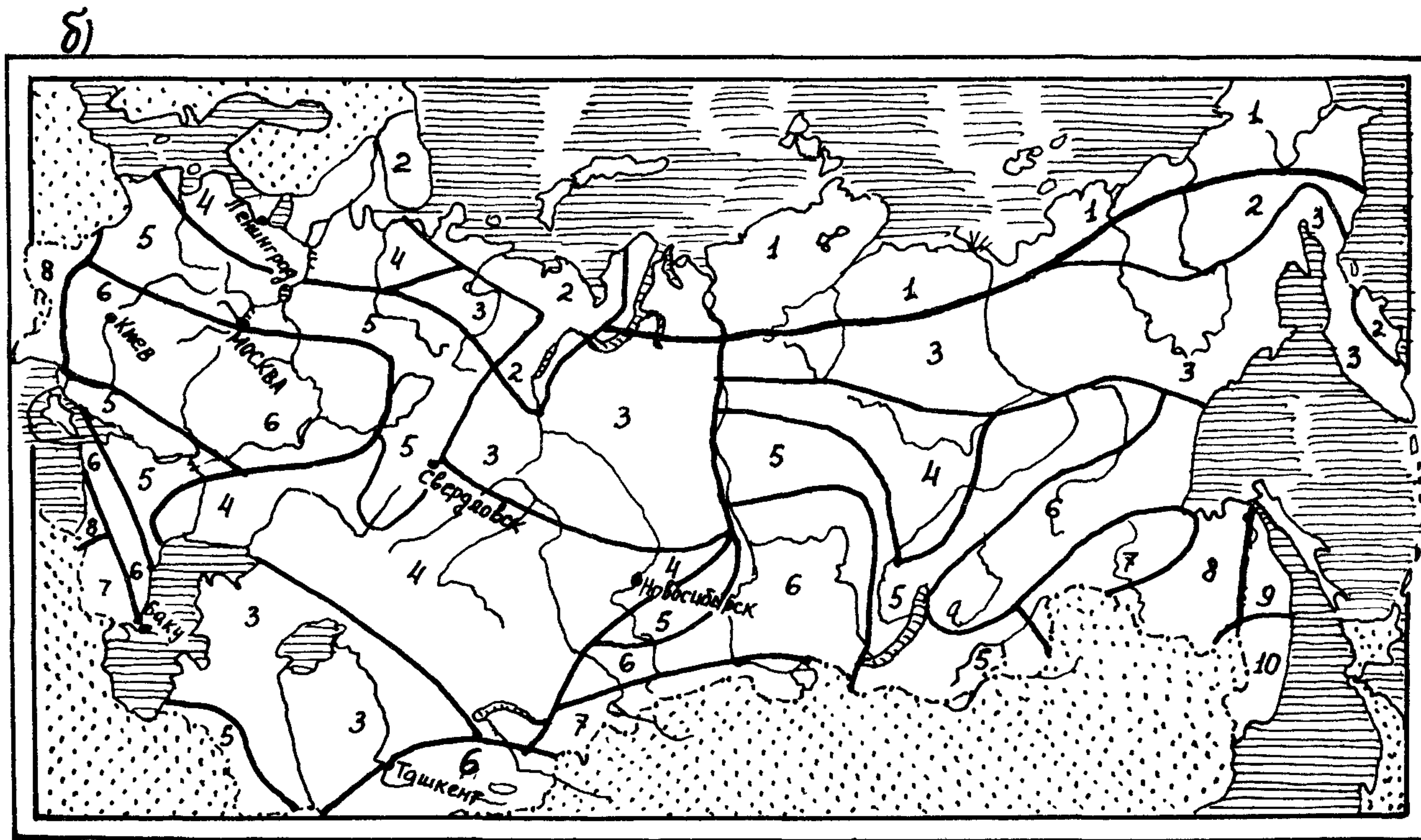
Рис Карта-схема ливневых районов: а—земного шара; б—СССР (Цифрами показаны номера районов)
