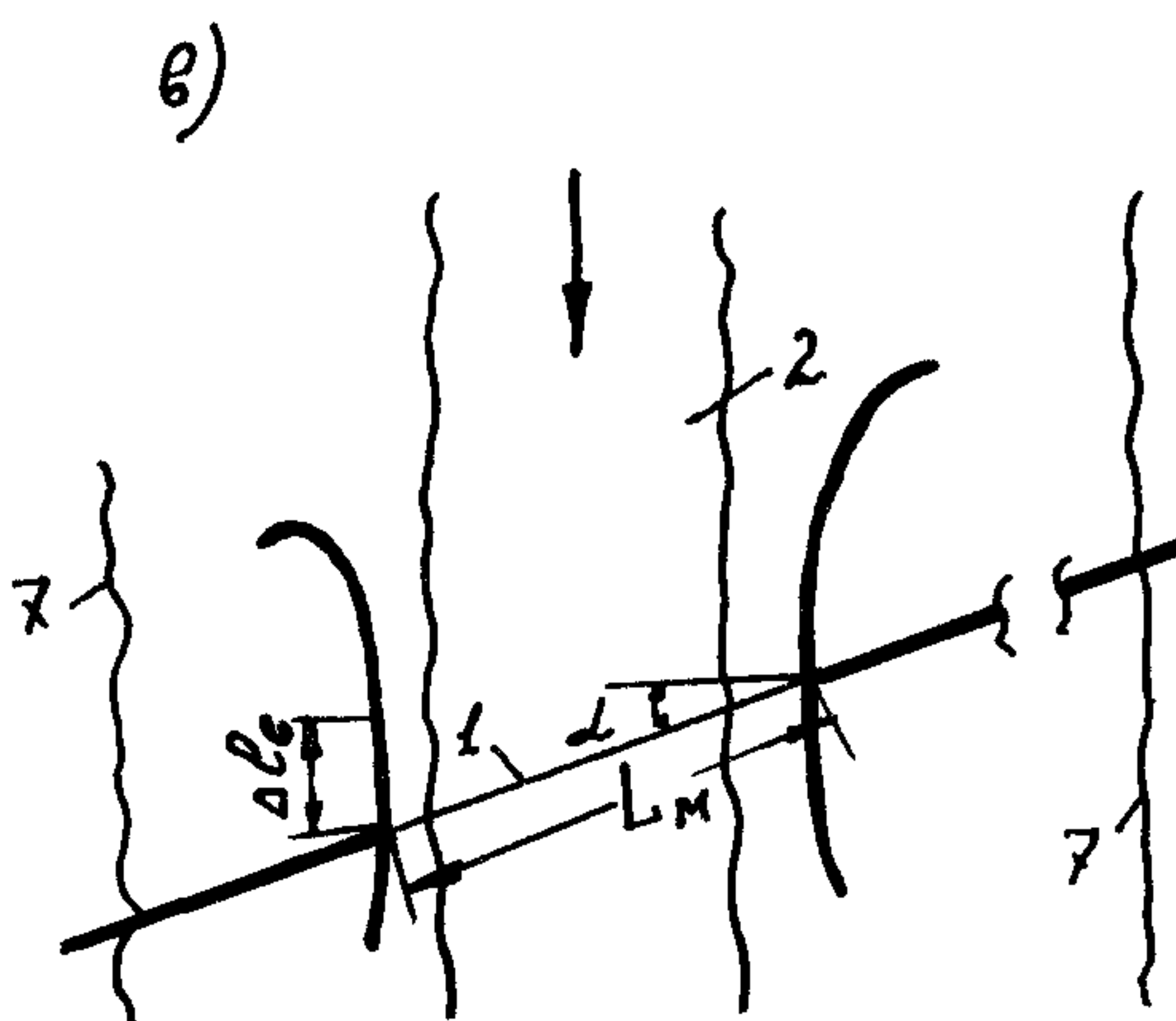
Рис. 14.4. Увеличение размеров дамб по ситуационным условиям:
