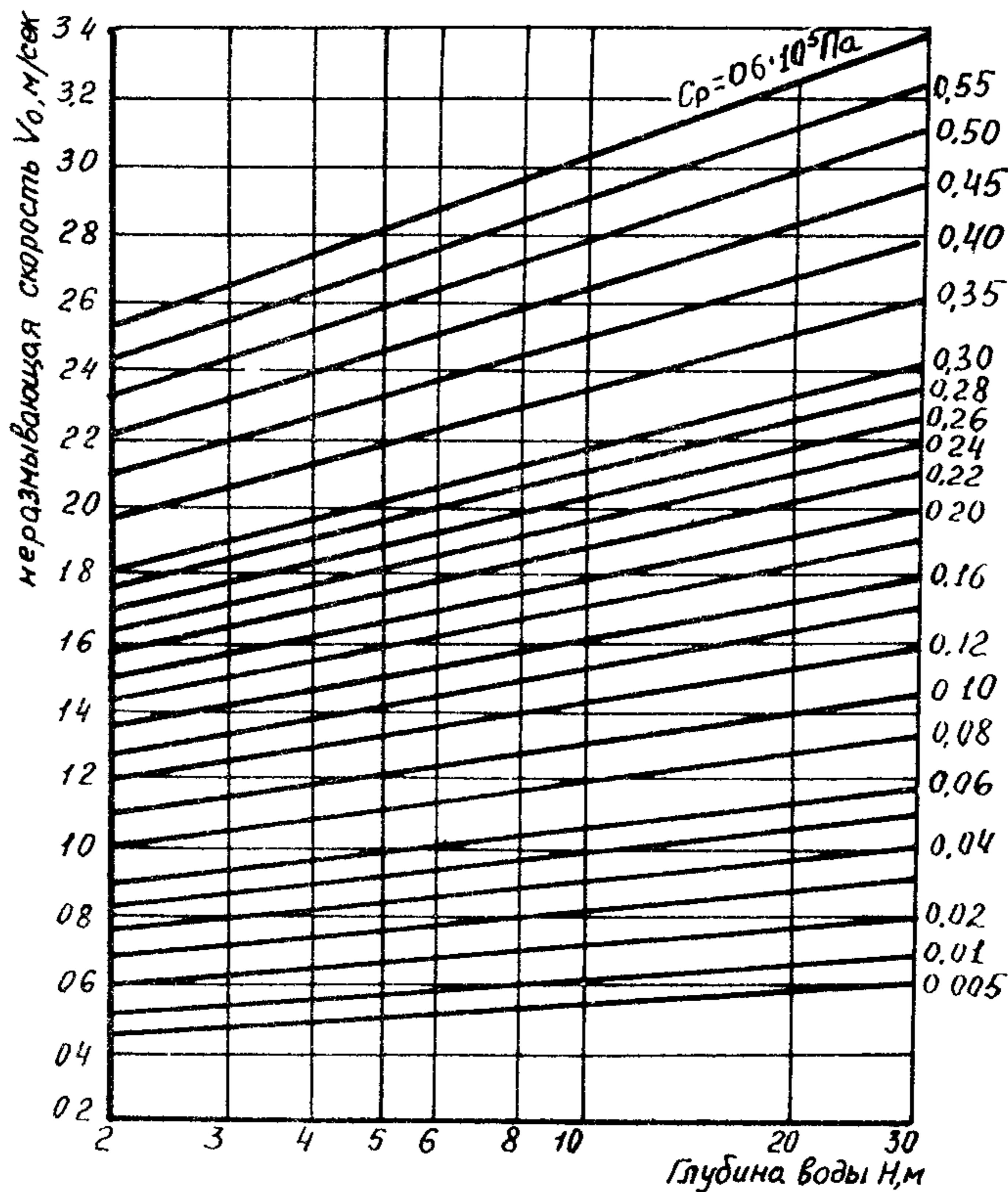
Рис 10.3 График для определения неразрывающей скорости связных грунтов по формуле Ц. Е. Мирцхулавы
