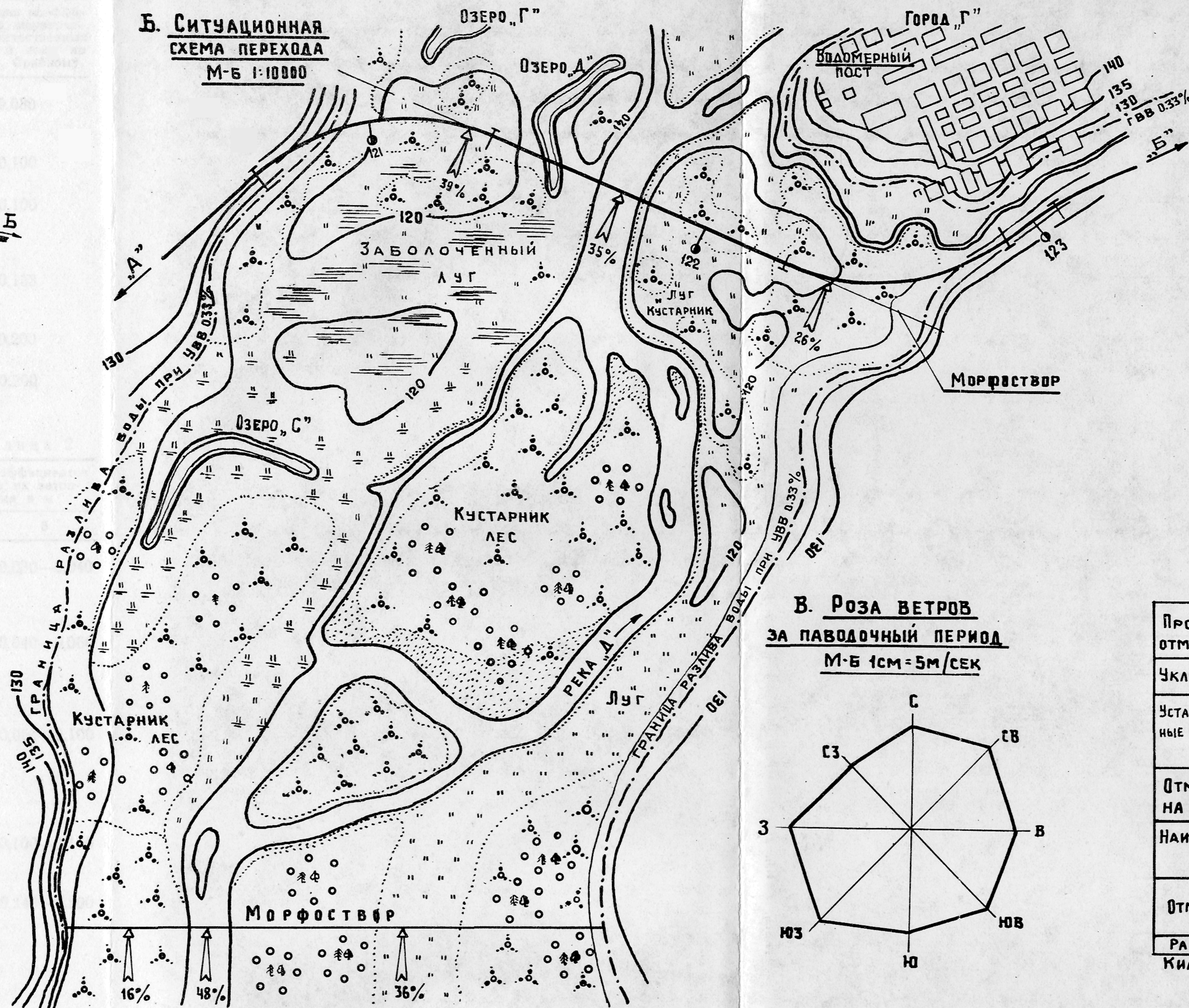
Рис. Пример оформления чертежей морфометрических работ: А—план бассейна; Б—ситуационная схема перехода; В—Роза ветров; Г—продольный профиль реки; Д—зависимости расхода и средней скорости течения воды для морфоствора выше оси перехода на 3100 м
