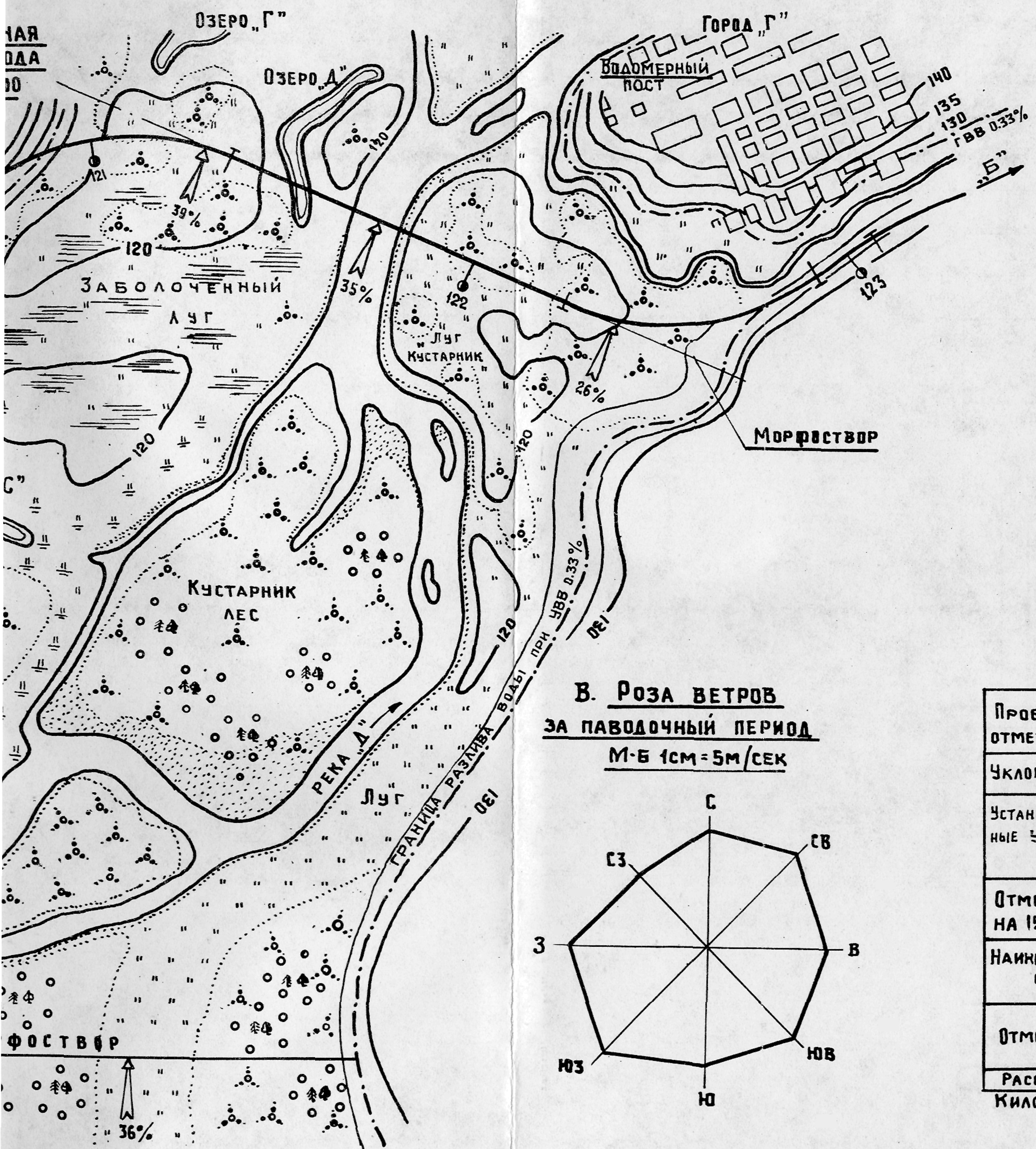
Рис. Пример оформления чертежей морфометрических работ: А—план бассейна; Б—ситуационная схема перехода; В—Роза ветров; Г—продольный профиль реки; Д—зависимости расхода и средней скорости течения воды для морфоствора выше оси перехода на 3100 м
