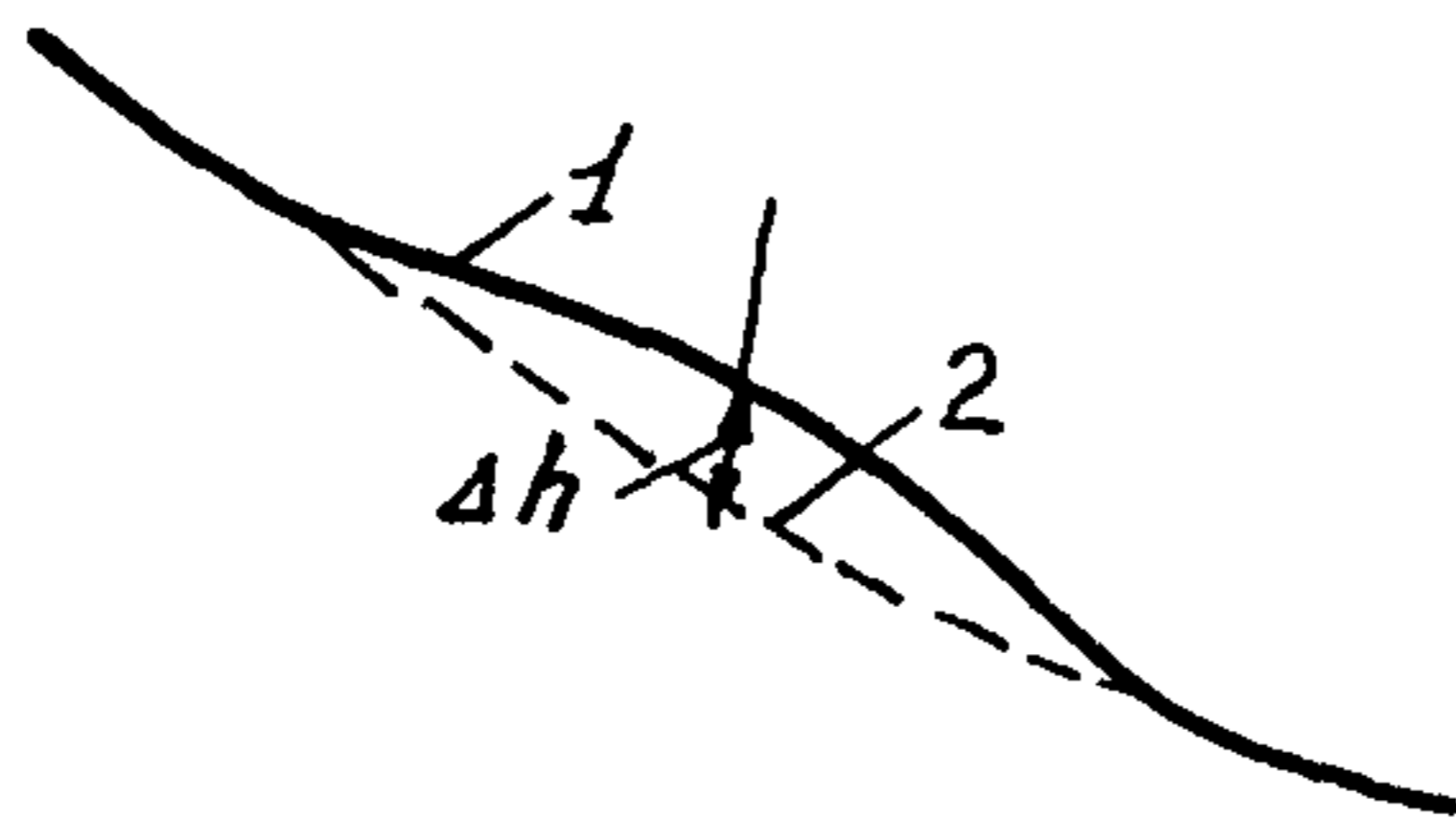
Рис. 119 Схема продольного профиля селевого лога на конусе выноса.
