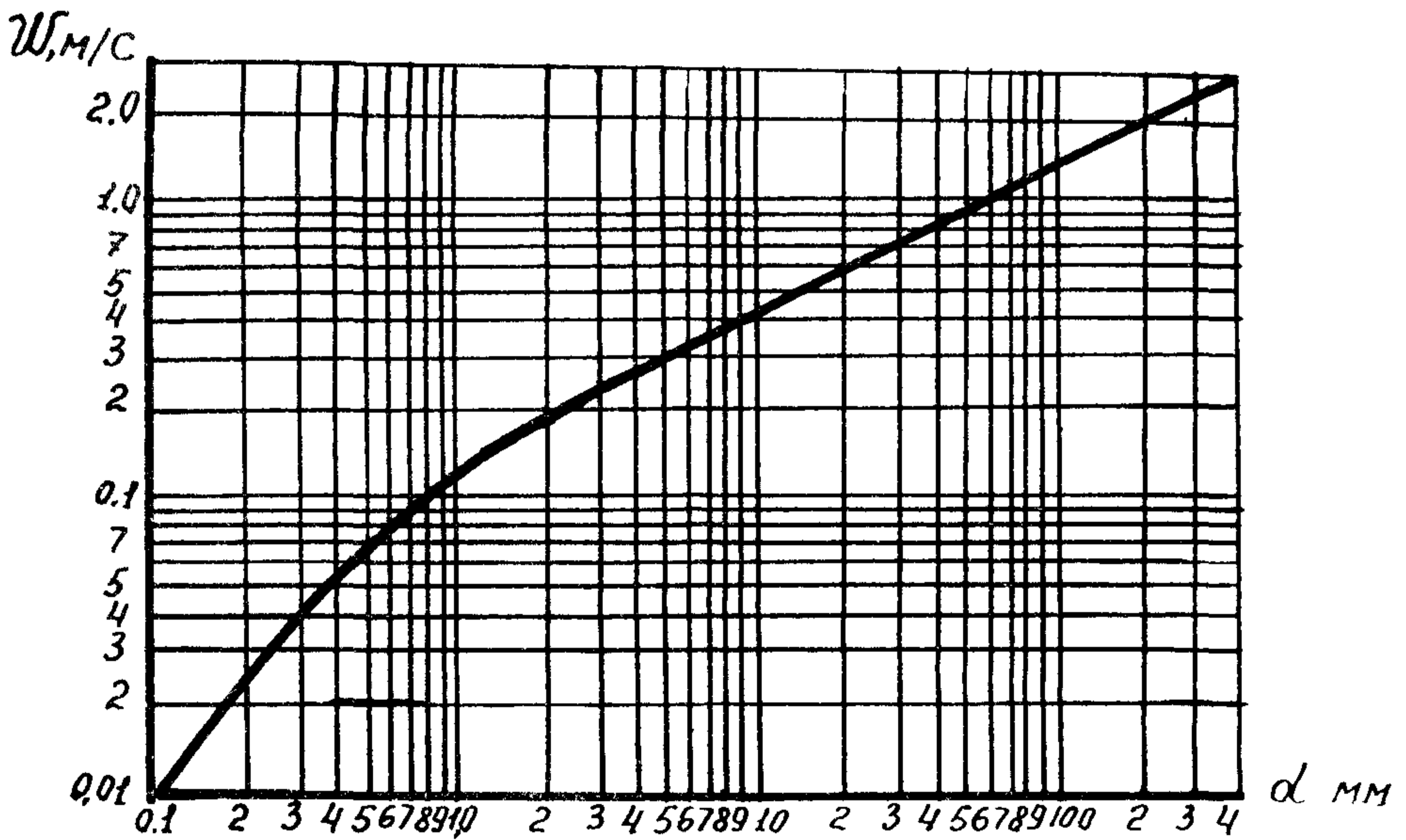
Рис 10.1 График для определения гидравлической крупности несвязных грунтов
