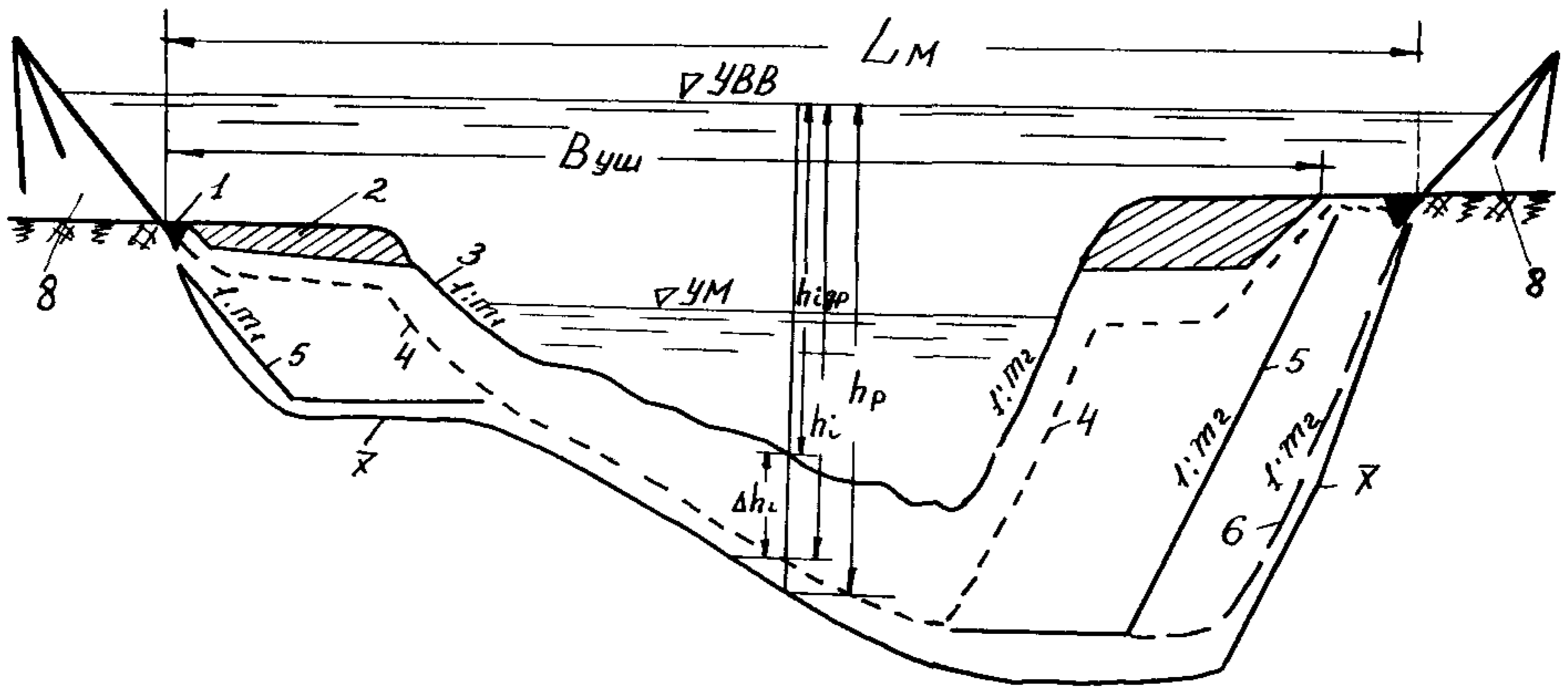
Рис 106 Расчетная линия общего размыва в подмостовом сечении:
