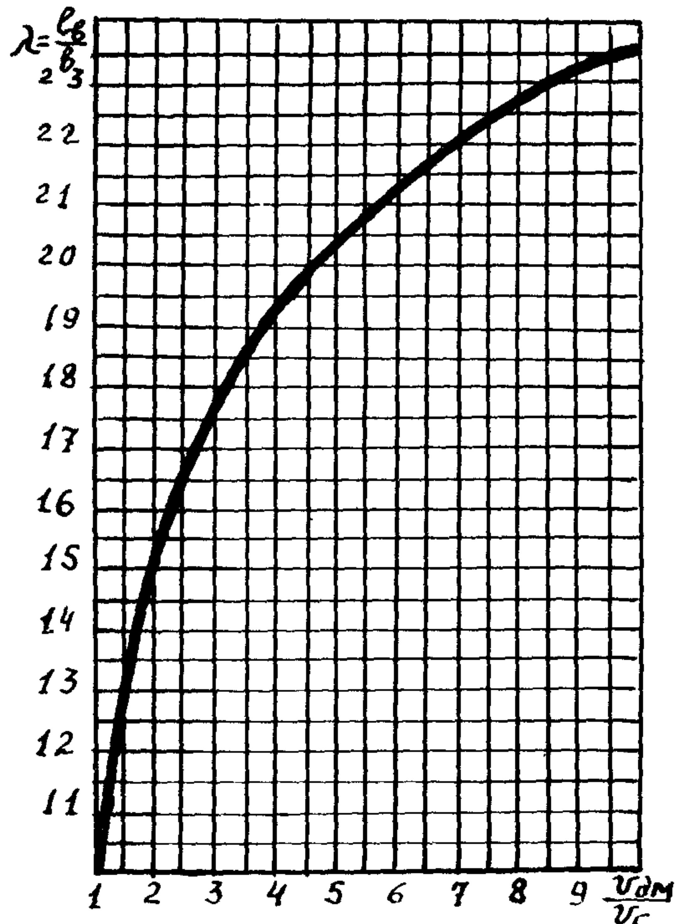
Рис. 14.5. График для определения полуосей дамбы \lambda = f\left(\frac{v_{\text{дм}}}{v_{\Gamma}}\right)
