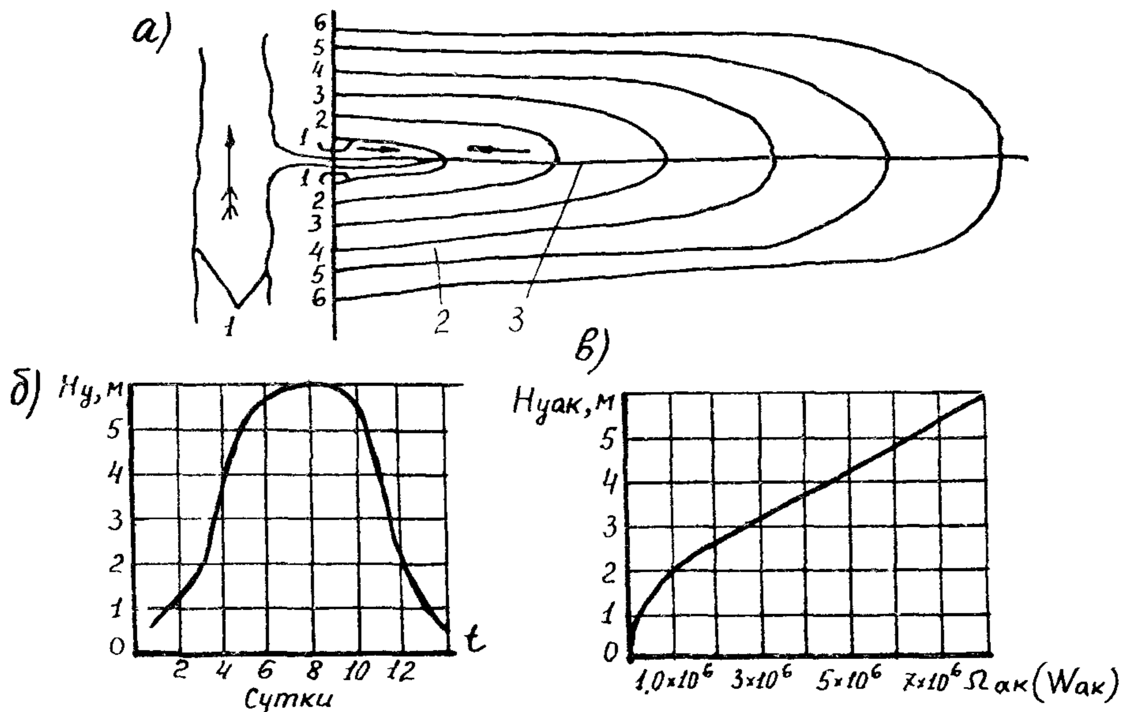
Рис. 11.2. Исходные материалы для расчета отверстий при переменном подборе: а—план затапливаемой акватории в горизонталях; б—график колебания уровня воды на источнике подпора; в—график изменения площади водного зеркала \Omega_{ак} или объемов воды W_{ак} в зоне аккумуляции в зависимости от уровня воды H_{уак} перед мостом;
