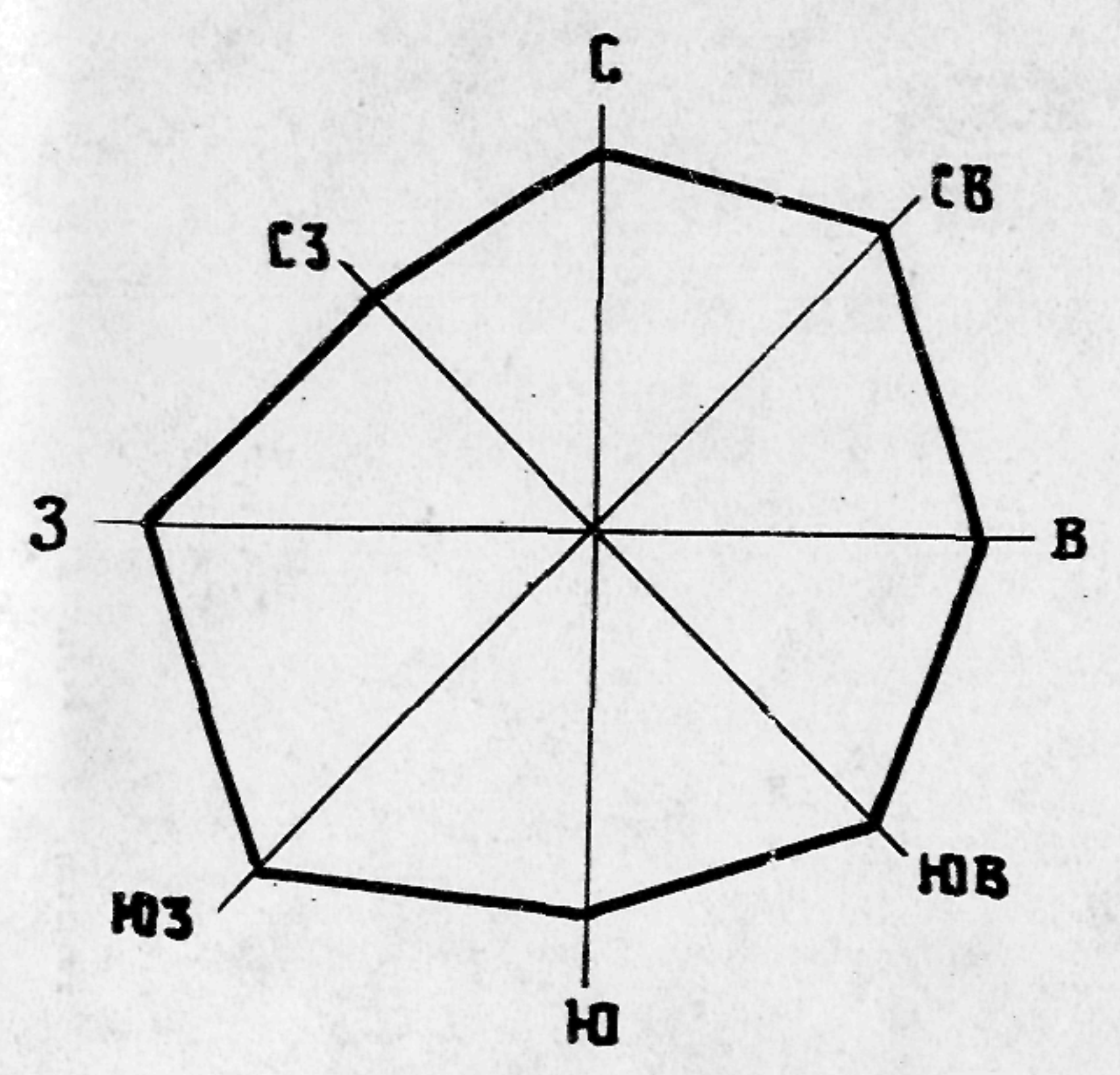
В. Роза ветров ЗА ПАВОДОЧНЫЙ ПЕРИОД М-Б 1см = 5м/сек
