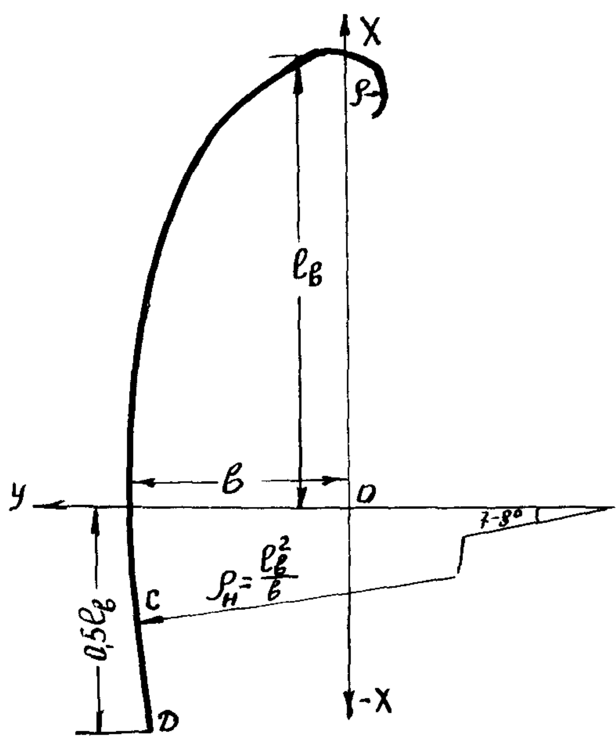
Рис. 14.2 Форма и размеры в осях верховой и низовой струенаправляющих дамб
