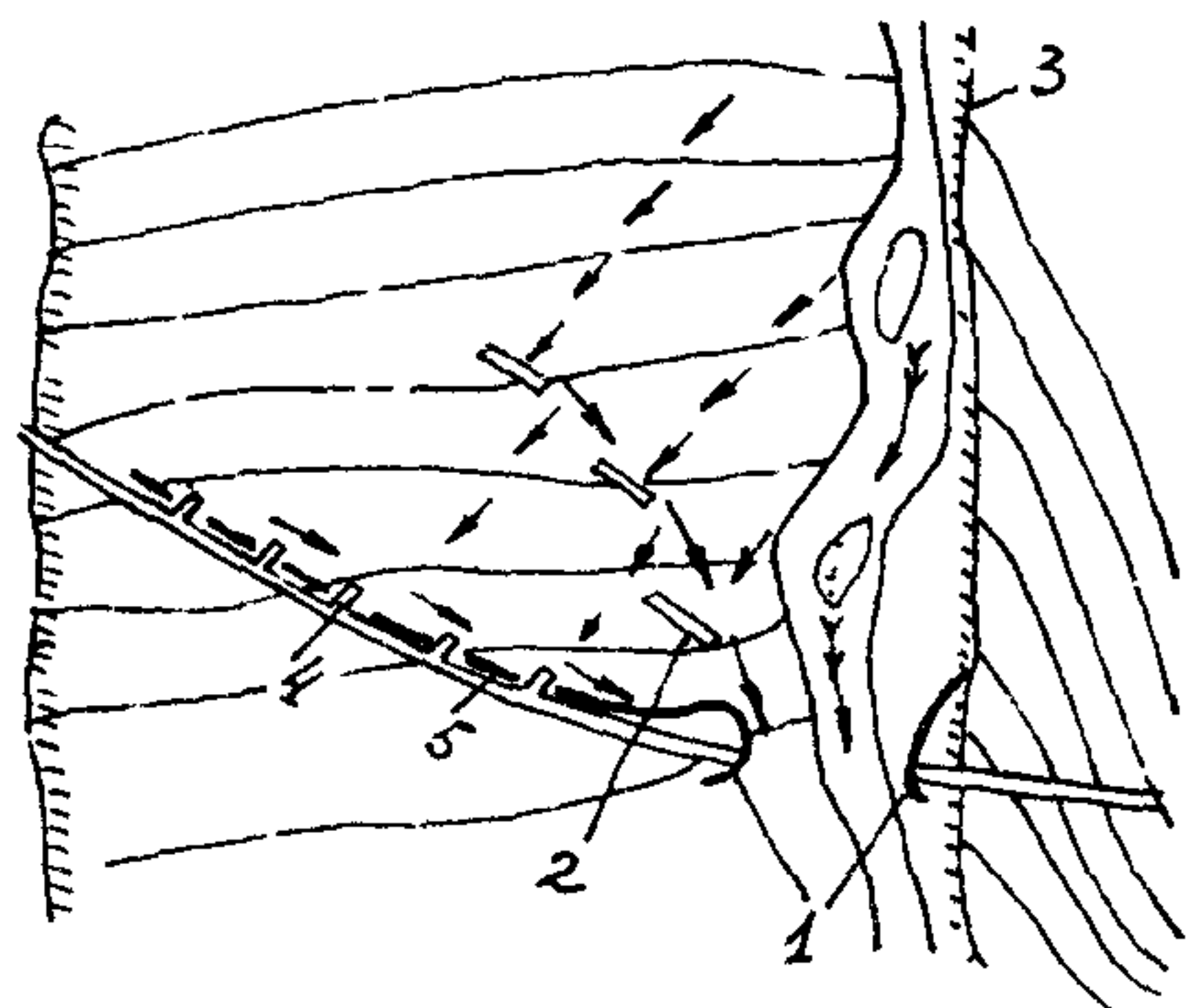
Рис 11.6 Регулирование потока шпорами с усилением подходов 1—дамбы замкнутого контура 2—шпоры 3—границы зоны блуждания, 4—траверсы 5— усиление подхода
