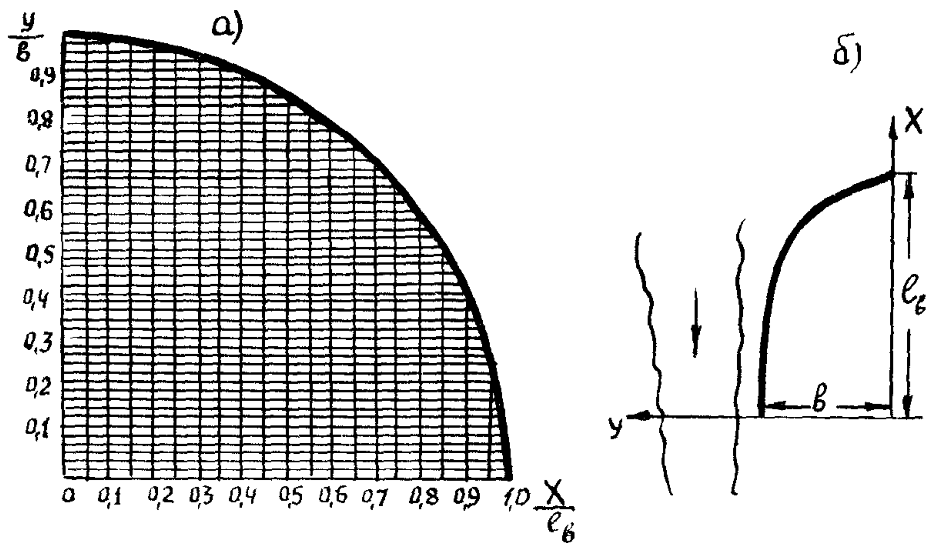
Рис. 14.3. Определение координат верховых струенаправляющих дамб:
