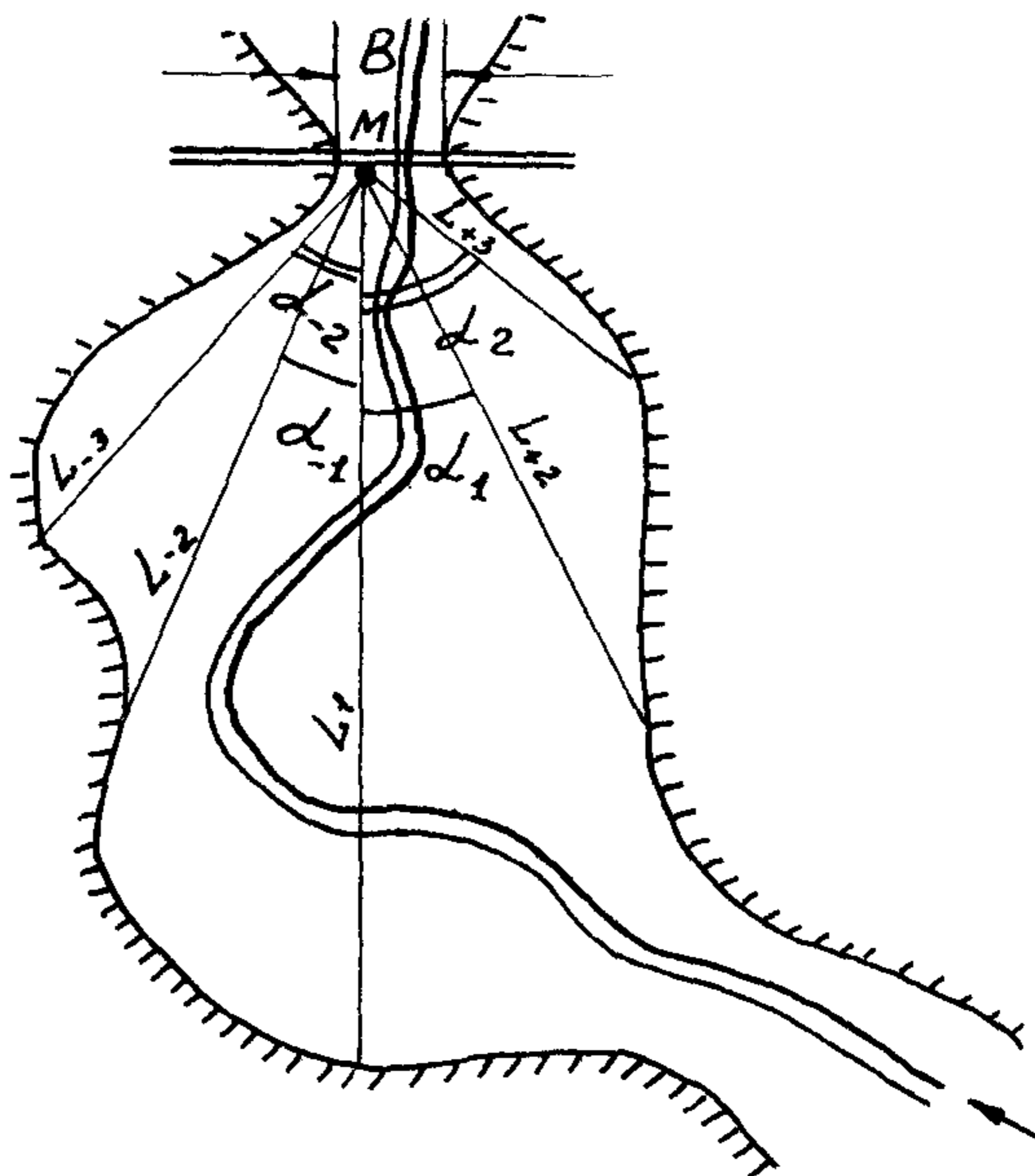
Рис. 12.4. Схема к расчету волн в узкости затопляемой поймы
