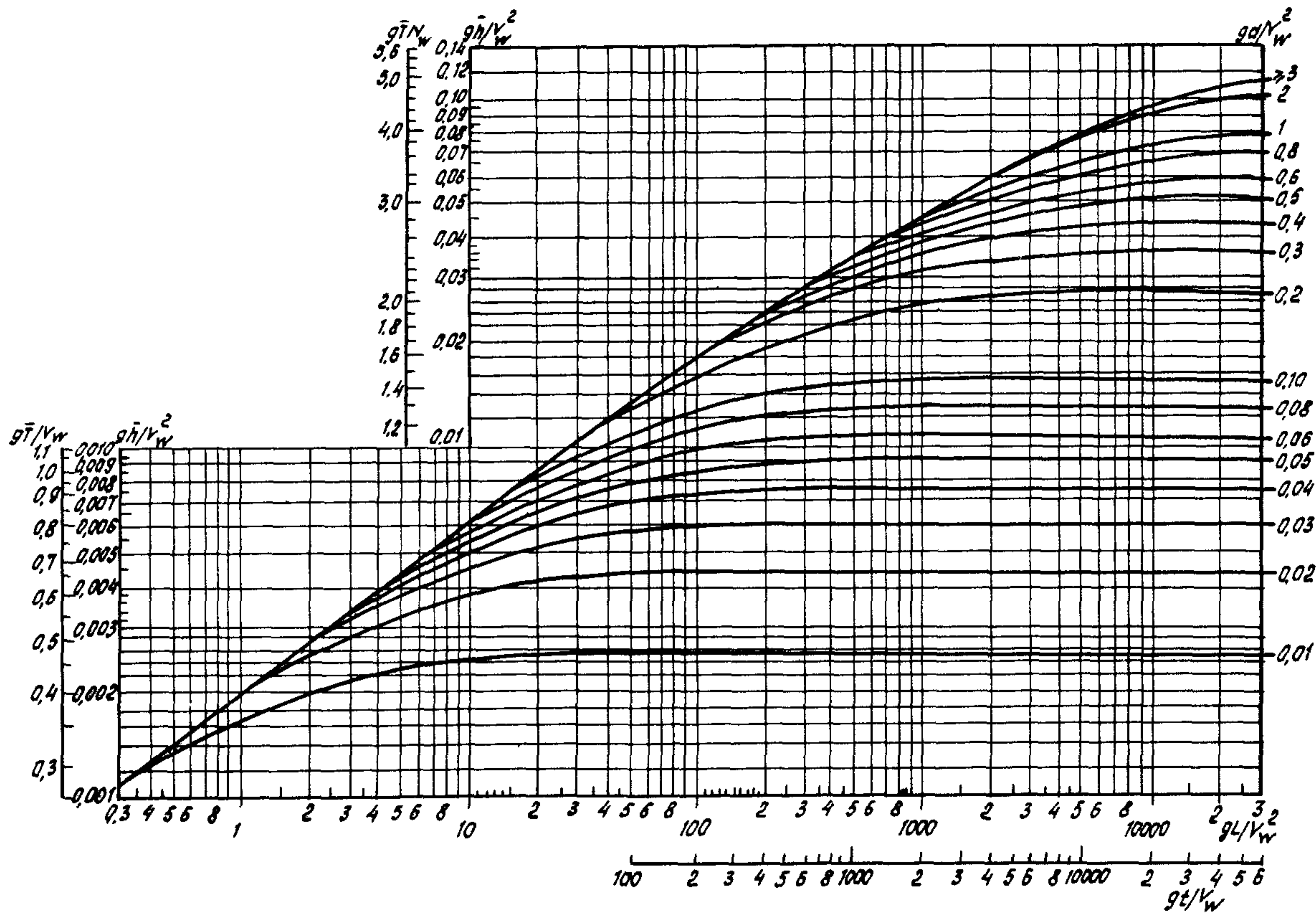
Рис. 12.3. Графики для определения элементов ветровых волн в глубоководной и мелководной зонах
