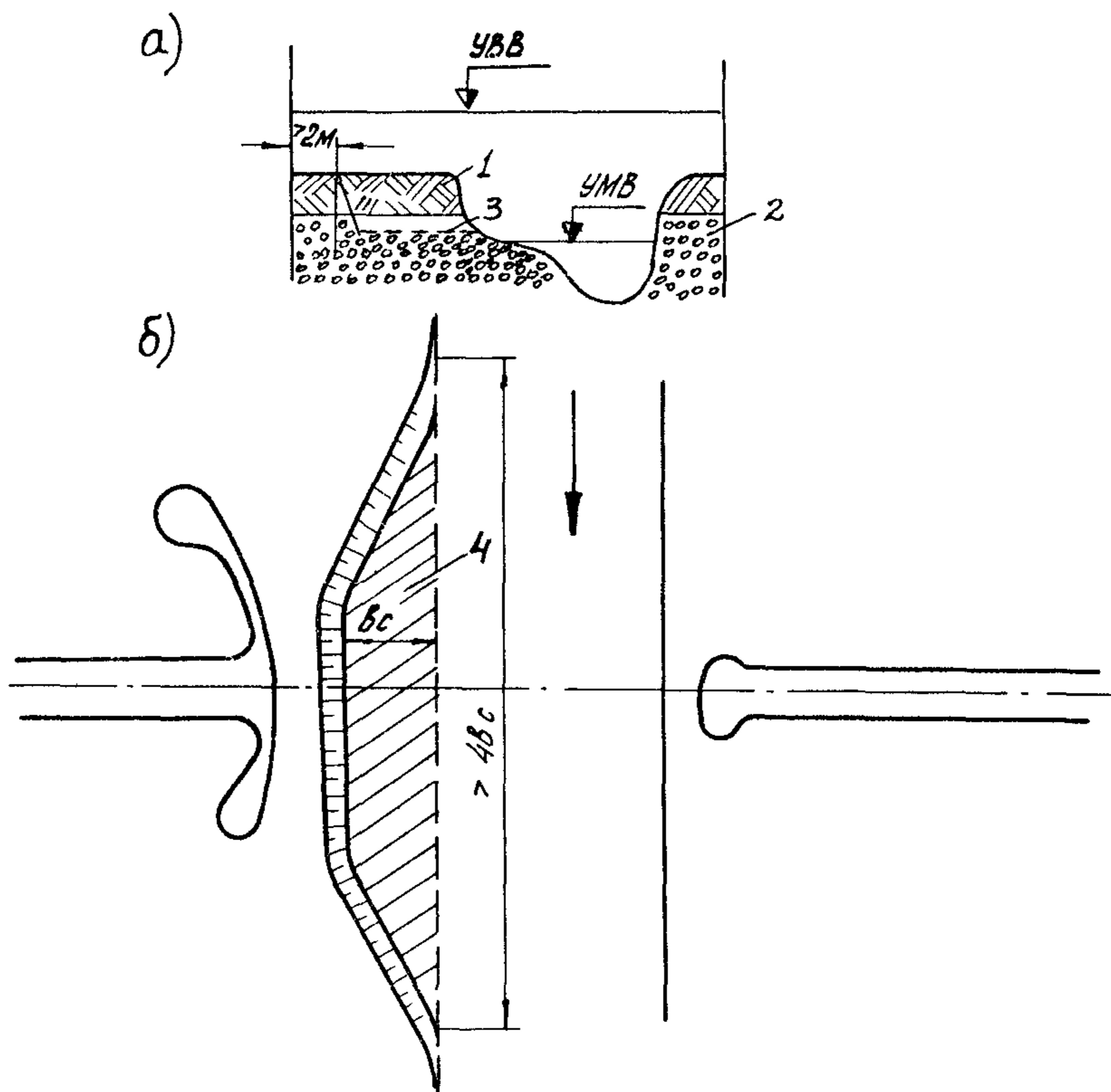
Рис. 14.1. Срезка грунта в подмостовом русле: а—поперечное сечение русла; б—план; 1—пойменный наилок; 2—аллювий; 3, 4—срезка грунта в профиле и плане
