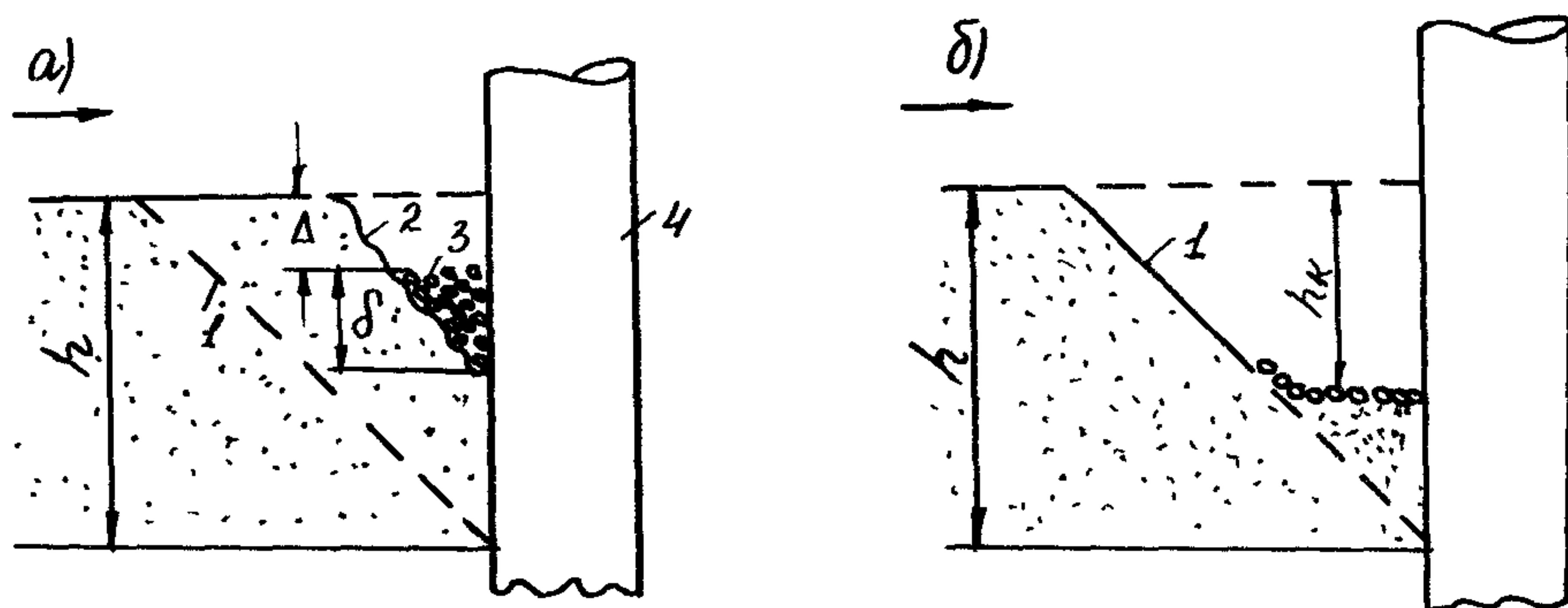
Рис 14.11. Укрепление опоры каменной наброской
