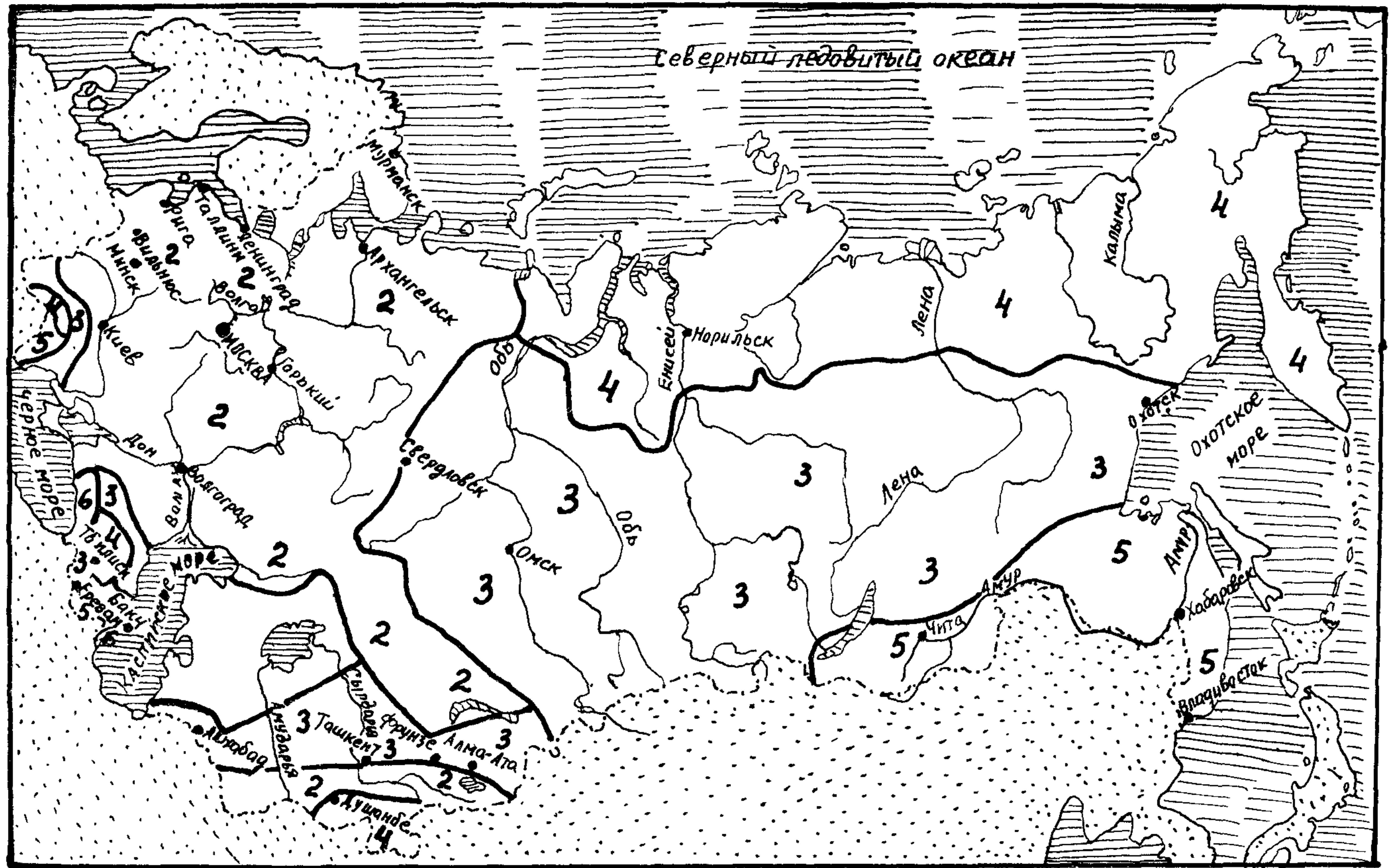
Рис. 7.14. Карта-схема гидрологического районирования типов внутригодичного распределения стока СССР
