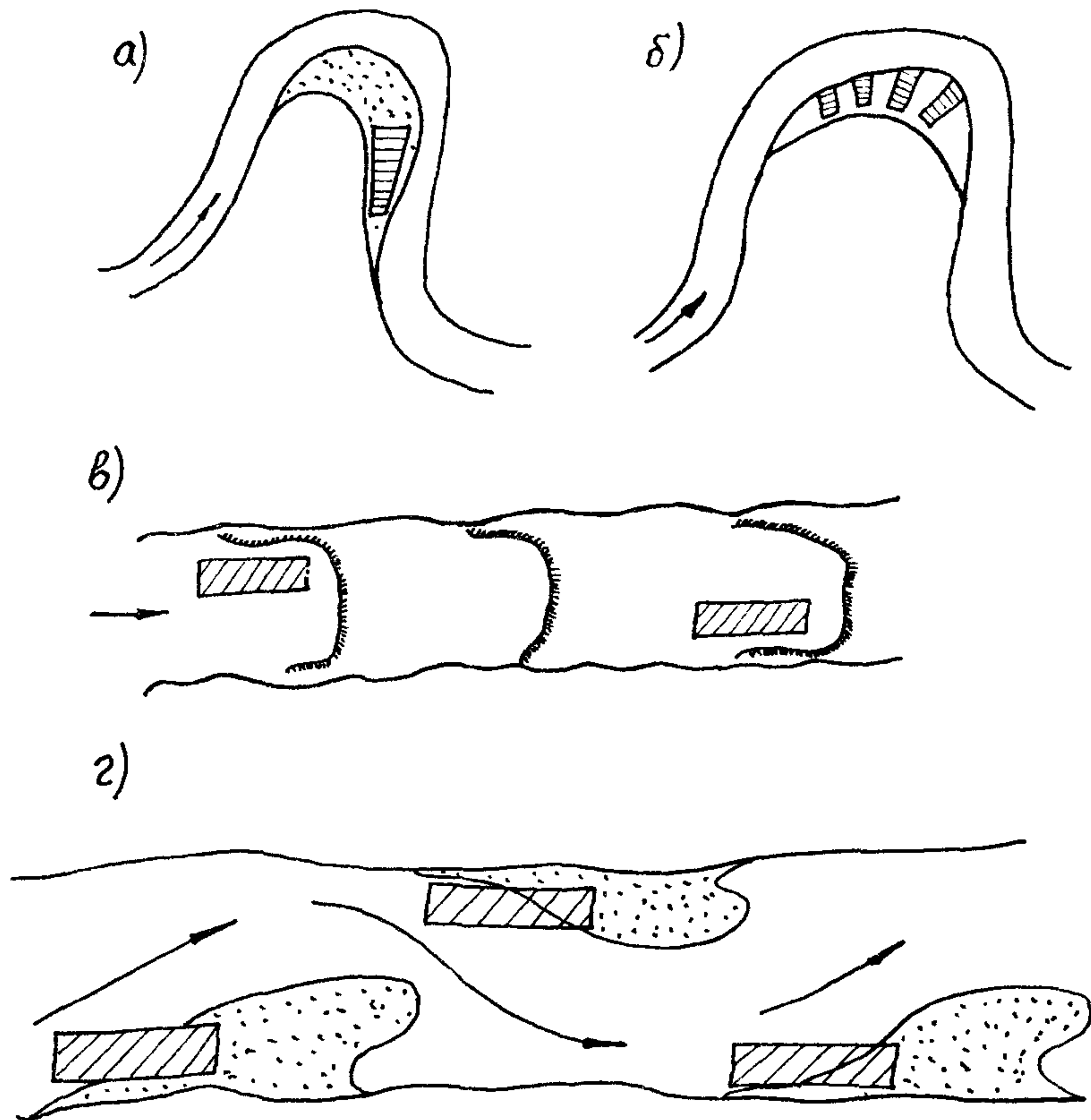
Рис. 15.4. Схема размещения карьеров:
