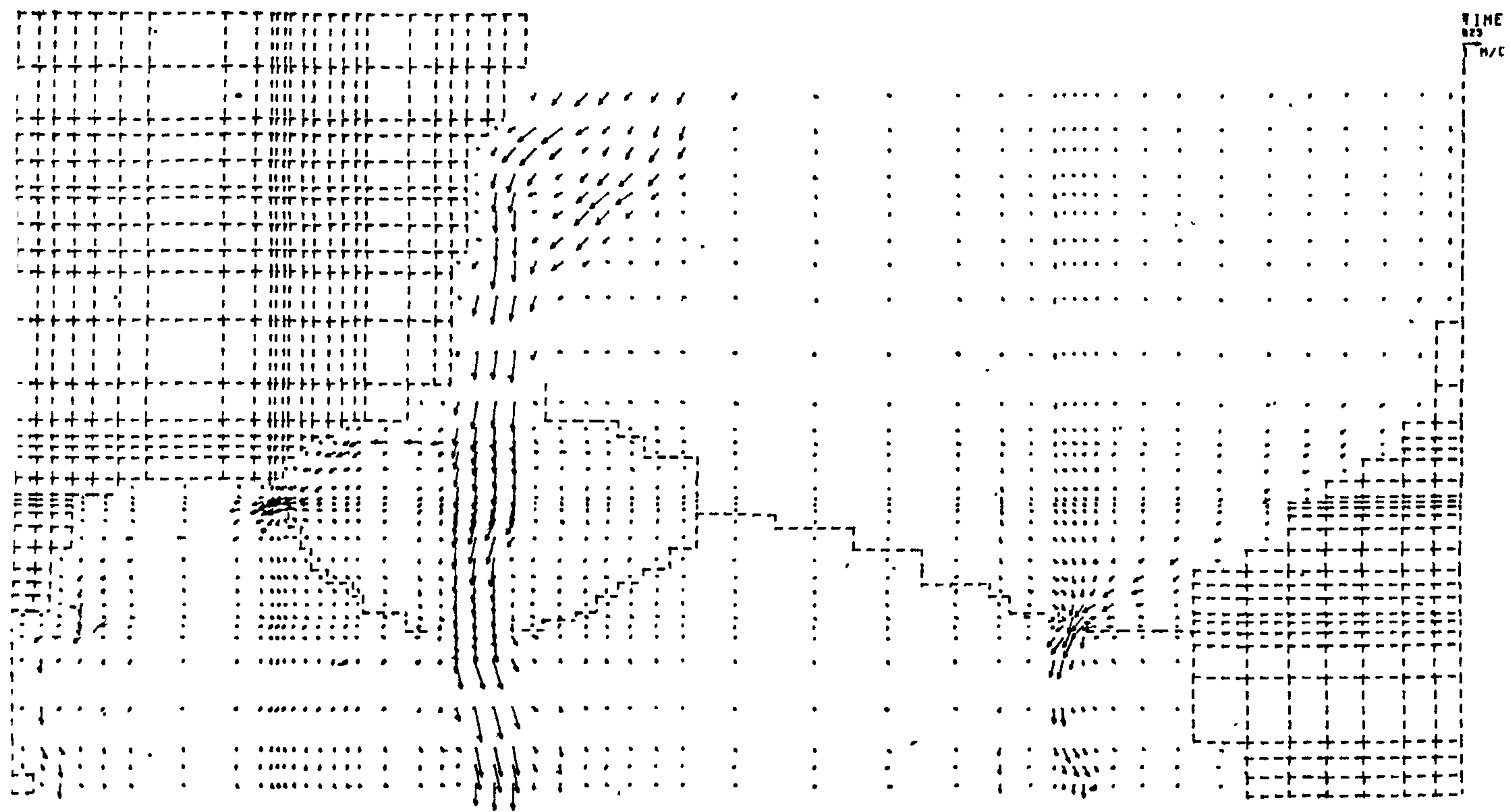
Рис. 2. План скоростей течений, полученный на графопостроителе
