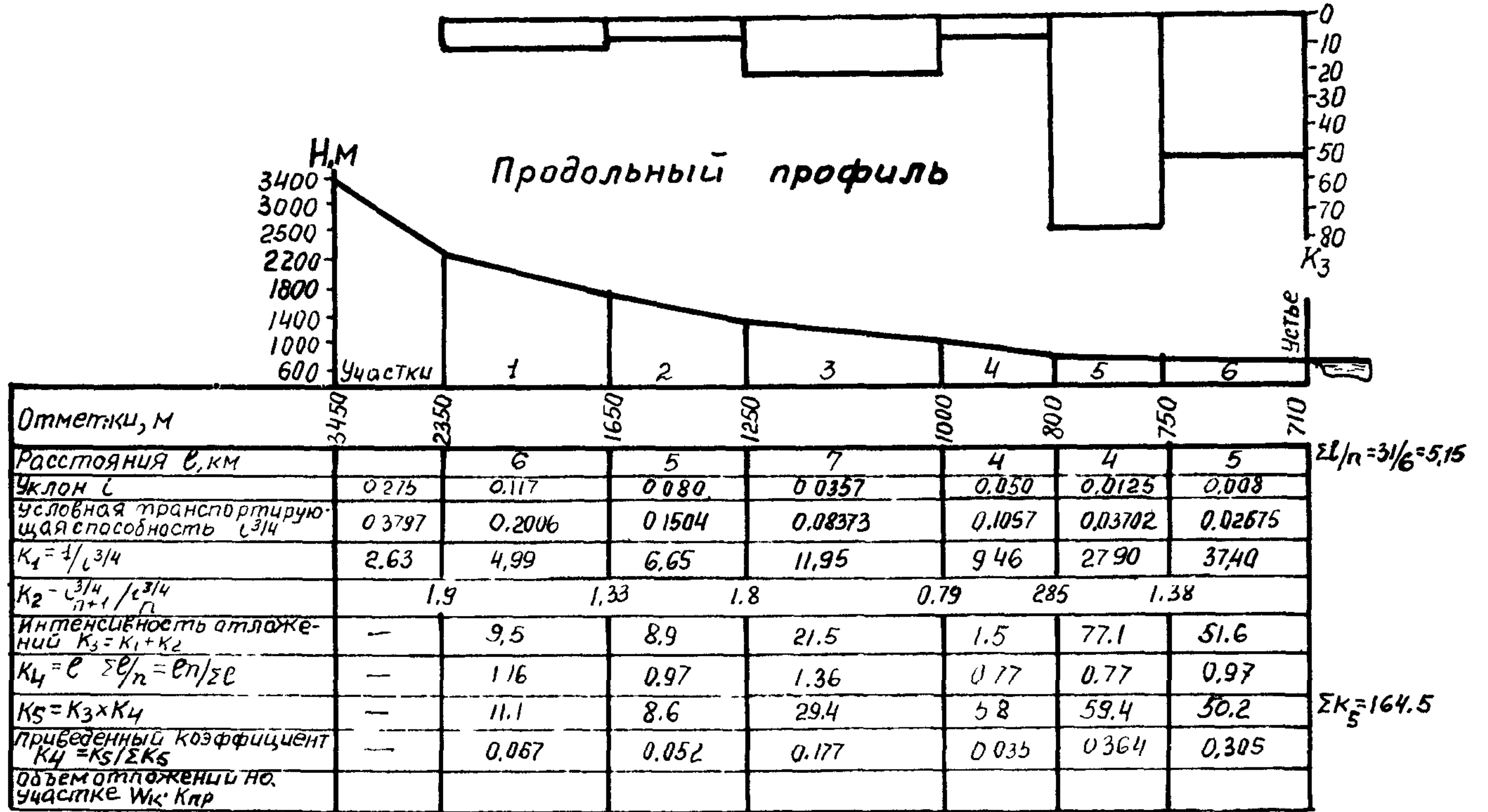
Рис 11.12 Пример определения высоты отложений наносов
