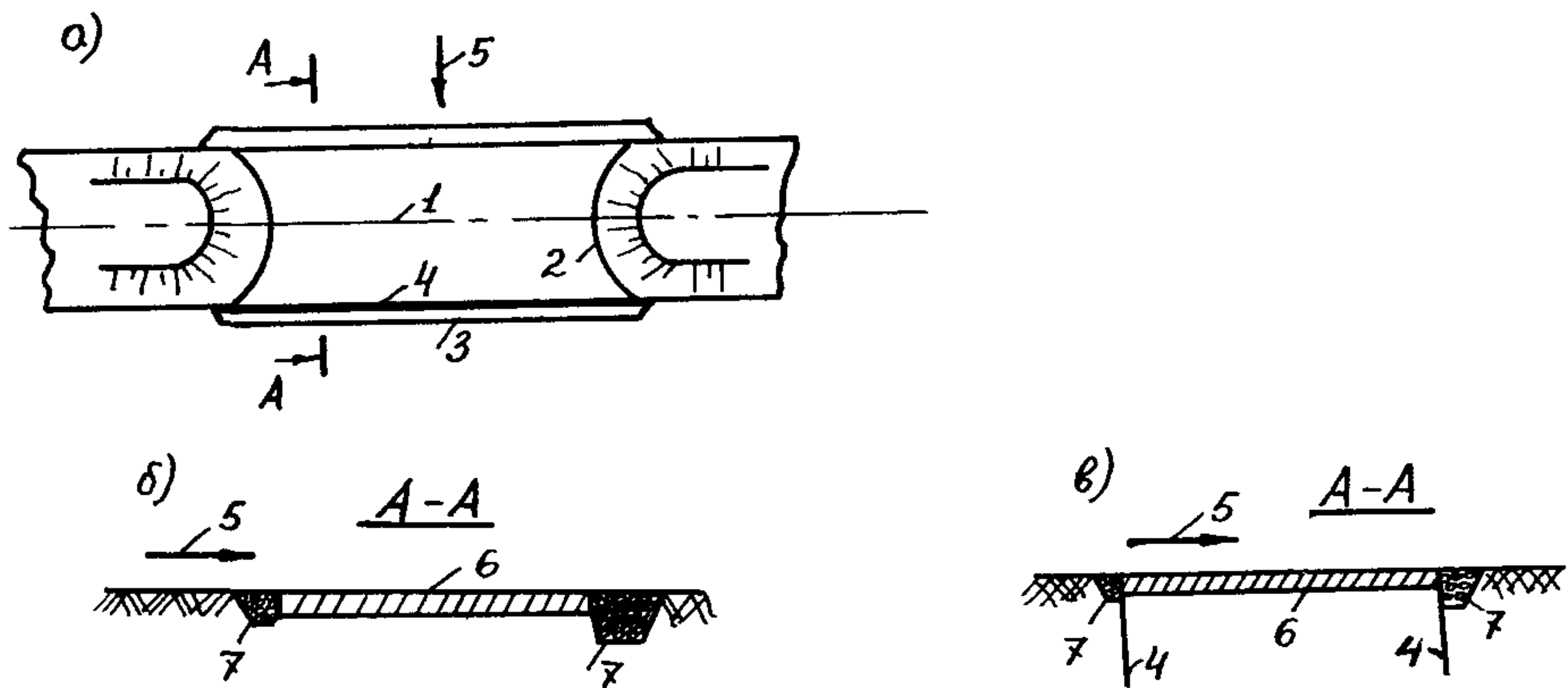
Рис. 14.13 Укрепление подмостового сечения
