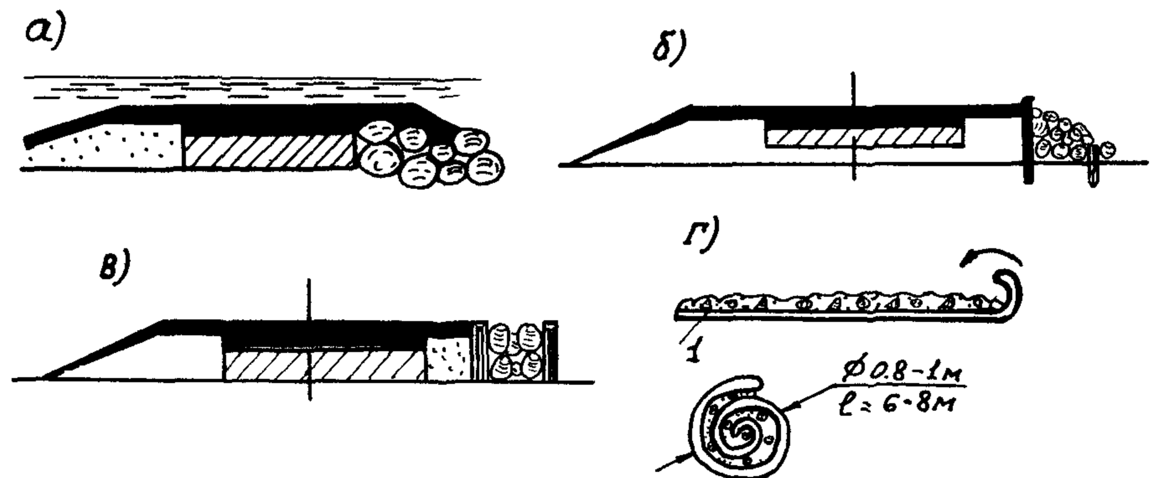
Рис. 13.2. Укрепление низового откоса при высоте насыпи до 0,5 м: а—низовой откос из каменной наброски; б—плетни с заполнением камнем и грунтом; в—ряжи, заполненные камнем, г—карабуры; 1—камень, грунт, дерн, хворост, солома
