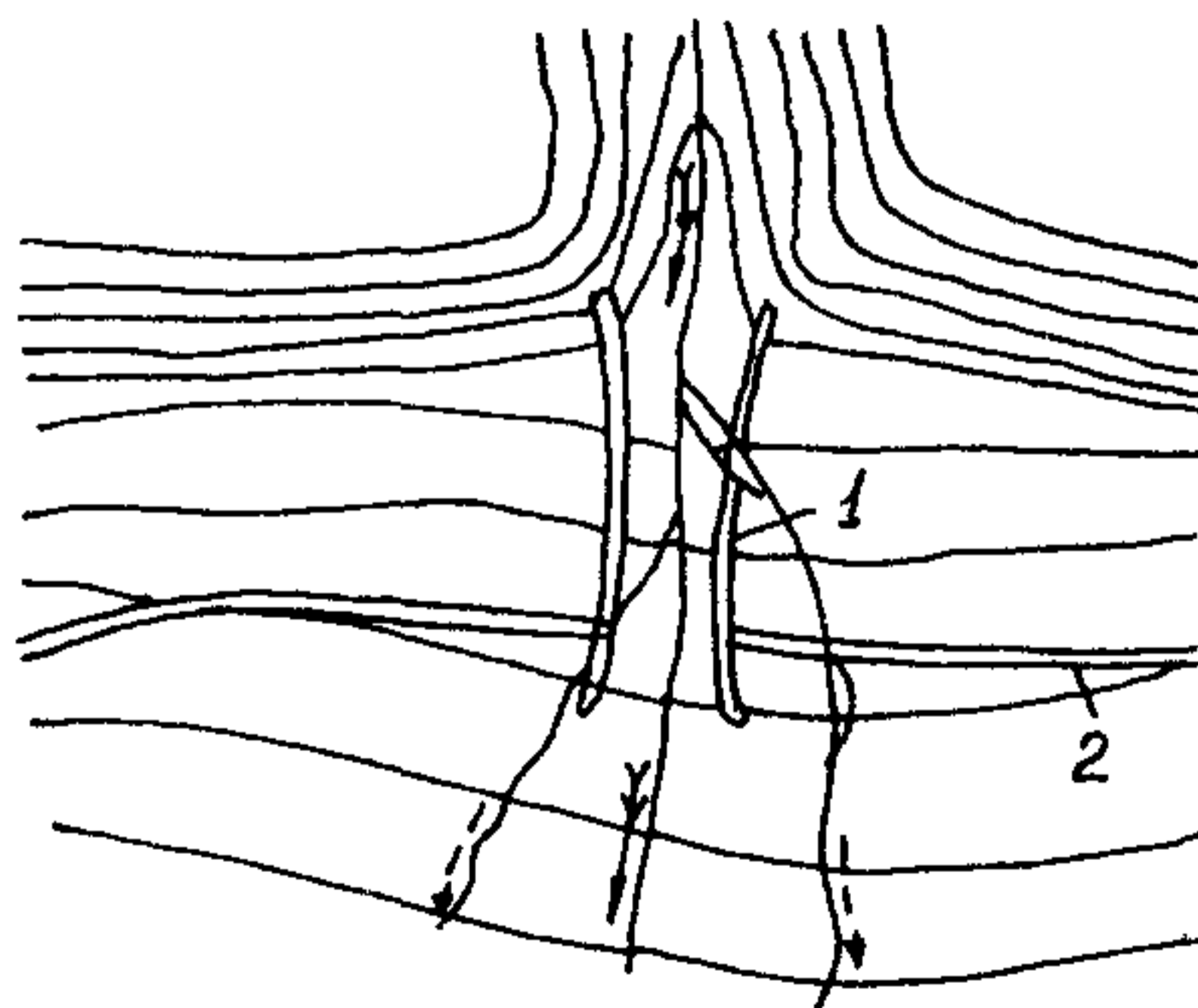
Рис 11.8 Схема струенаправляющих дамб на переходе через конус выноса
