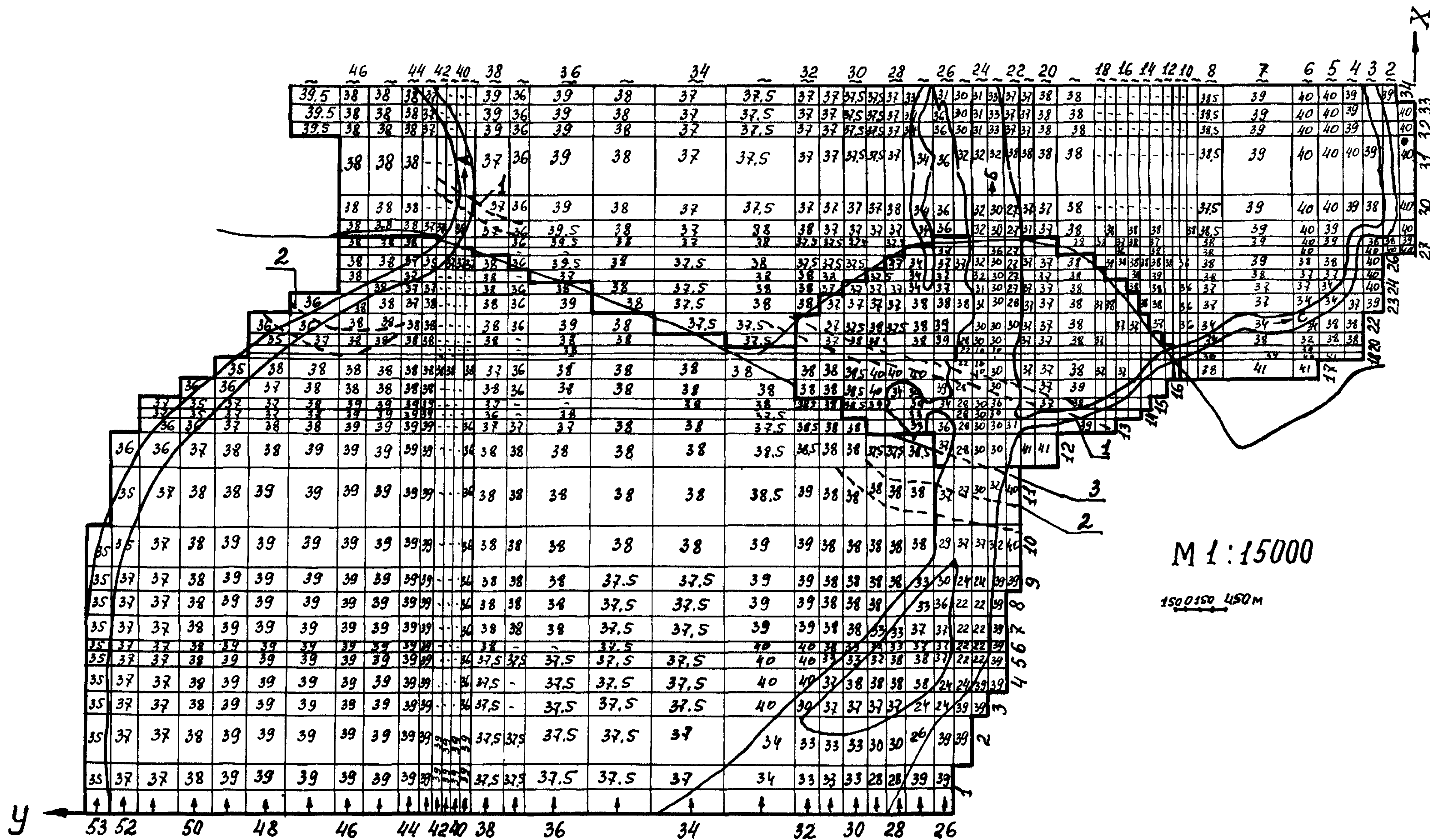
Рис. 1. Расчетная сетка конечных элементов: Цифрами в ячейках показаны отметки земли (в м); по контуру сетки—номера ячеек по осям X и Y; стрелками показан участок, где задан расход воды; волнистыми линиями—уровень; 1—газопровод; 2—нефтепровод; 3—паромная переправа
