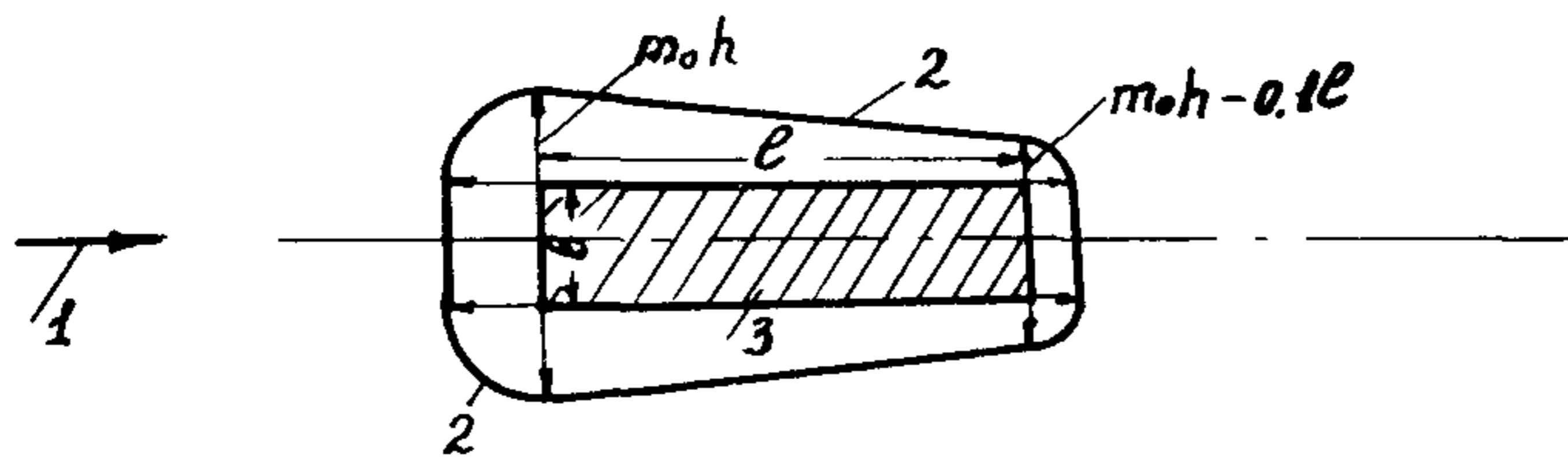
Рис. 14.10. Размеры схематизированной воронки в плане: 1—направление течения, 2—бровка воронки; 3—опора
